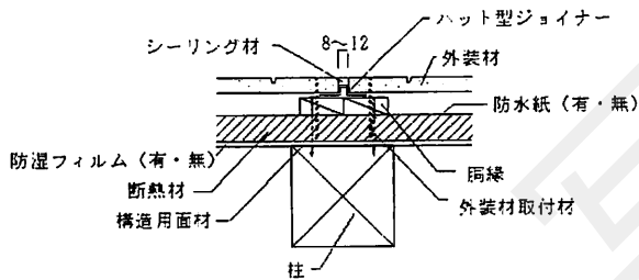
A部詳細図
