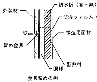
B部詳細図
