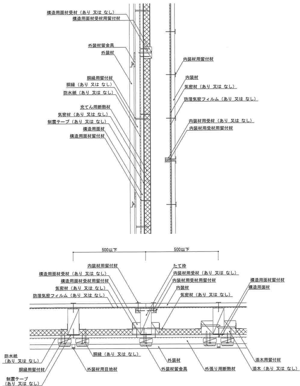
図2 構造説明図
