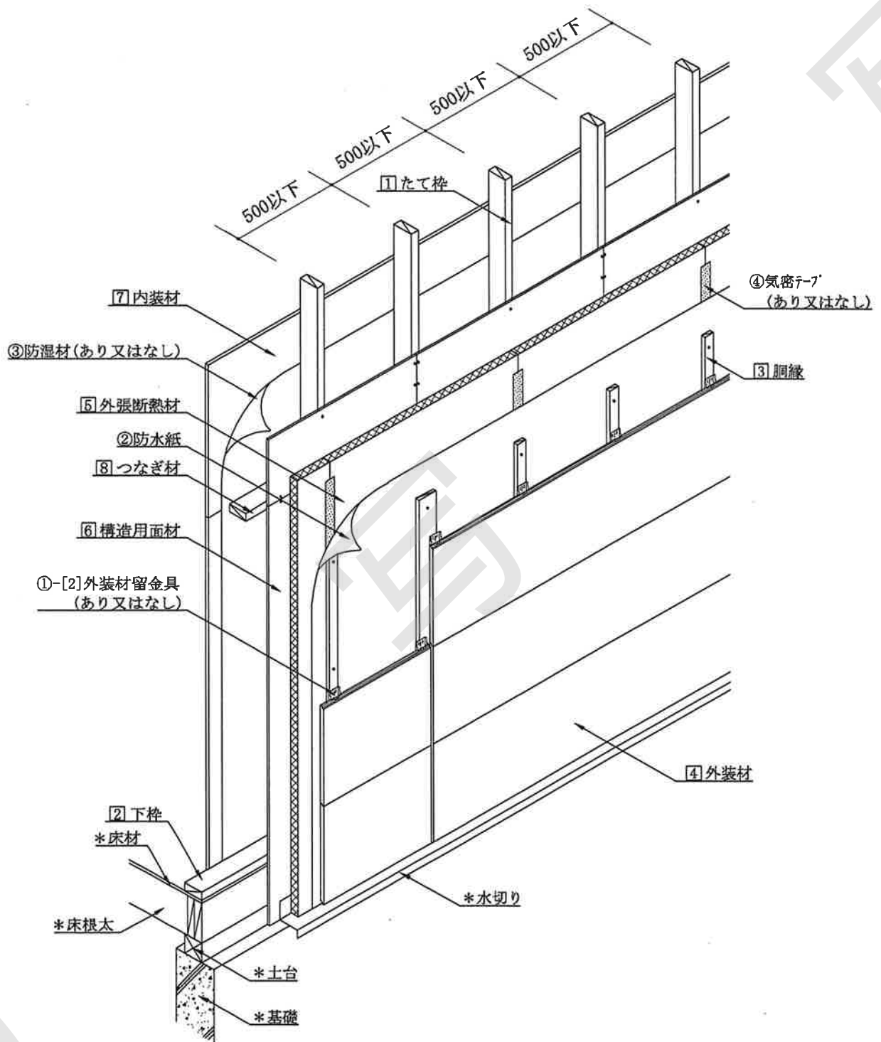
透視図
