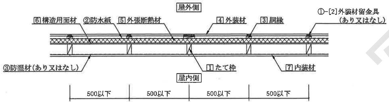
水平断面図
