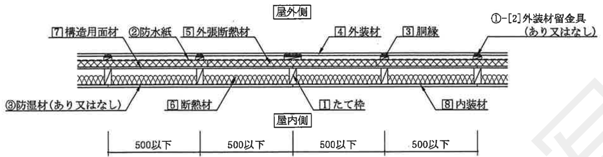
水平断面図
