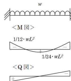
図-5 大梁(両端固定)の 長期許容応力度計算時モデル
