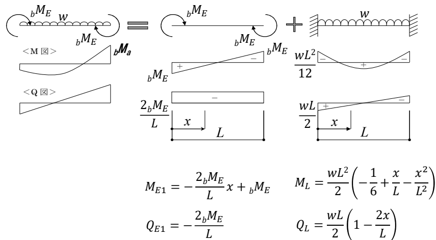
図-3 大梁(両端固定)の短期許容応力度計算時モデル
