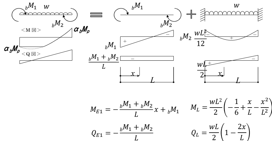
図-1 大梁(両端固定)の終局時応力モデル
