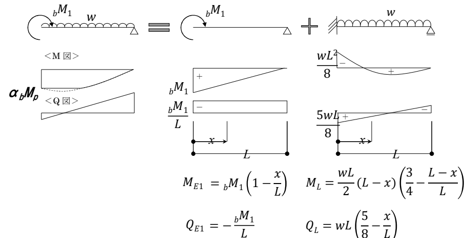
図-2 大梁(片側ピン接合)の終局時応力モデル
