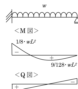
図-6 大梁(片側ピン接合)の 長期許容応力度計算時モデル
