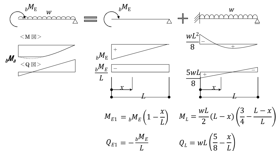
図-4 大梁(片側ピン接合)の短期許容応力度計算時モデル
