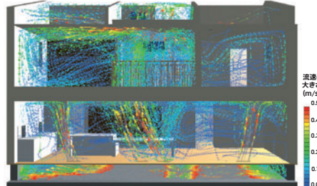
※ 首都大学東京 須永研究室による、ネオマの家 IBARAKI SAKAI MODEL における CFD 解析 (シミュレーション結果) の一例。(共同研究)
