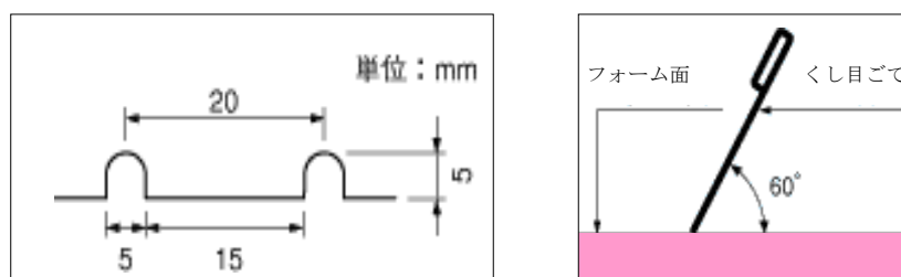
図一 4 くし目ごてくし目例及び施工方法
