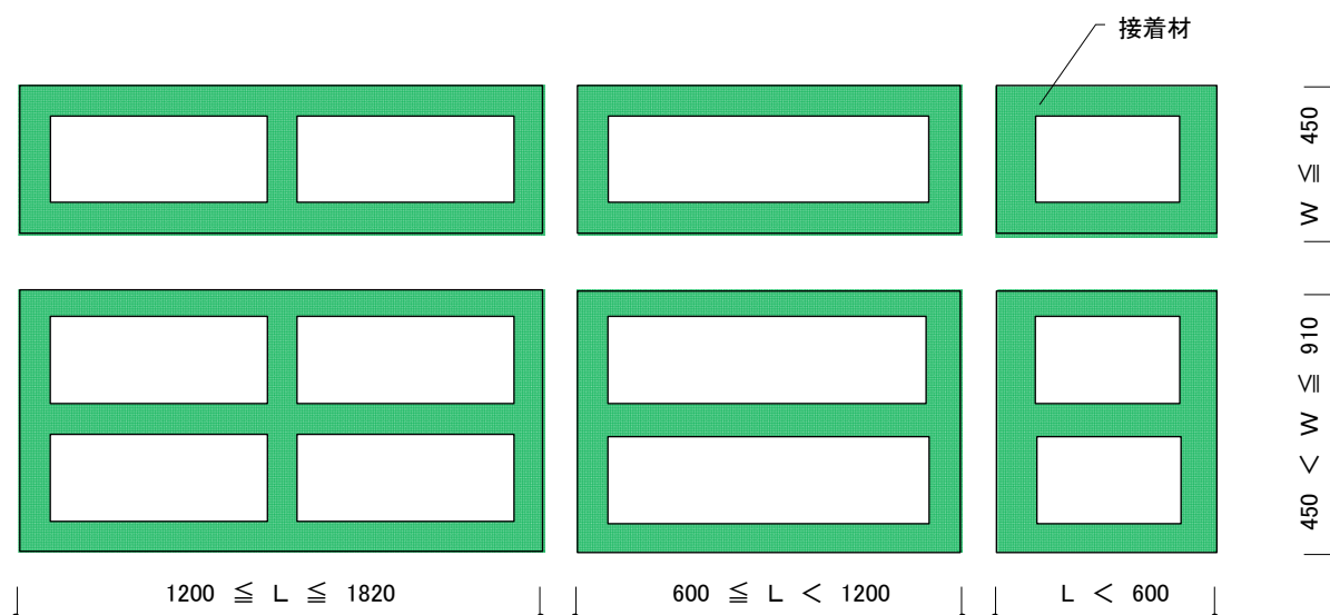
図一 3 パネル幅、長さ毎の接着剤の塗布位置
