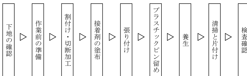
図-1 施工手順
