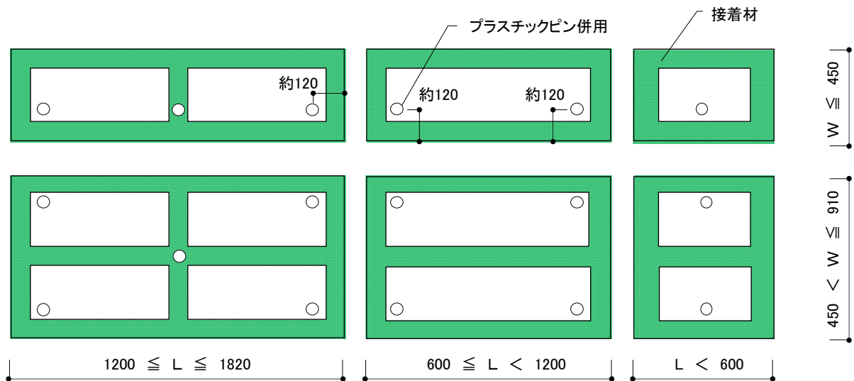
図ー5 プラスチックピンの標準位置
