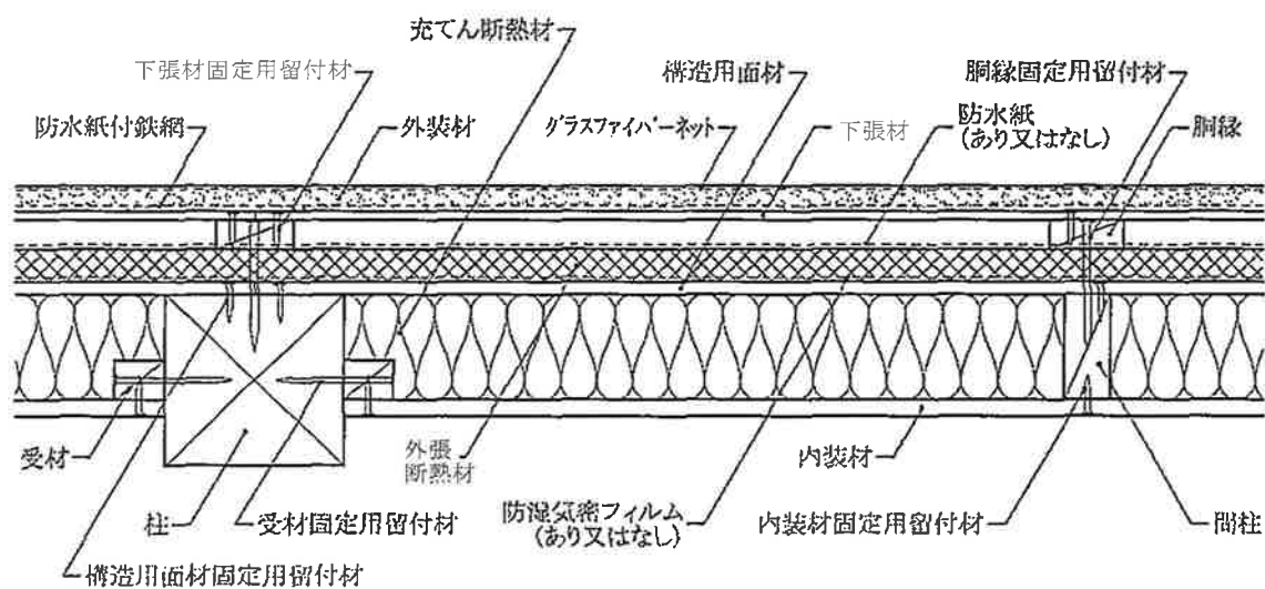
水平断面図
