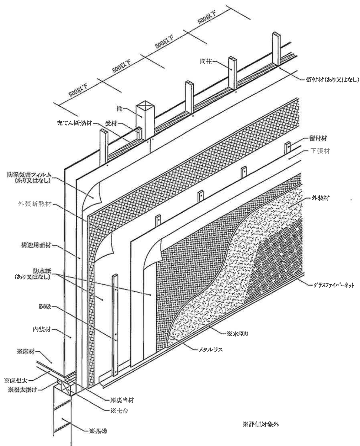
透視図
