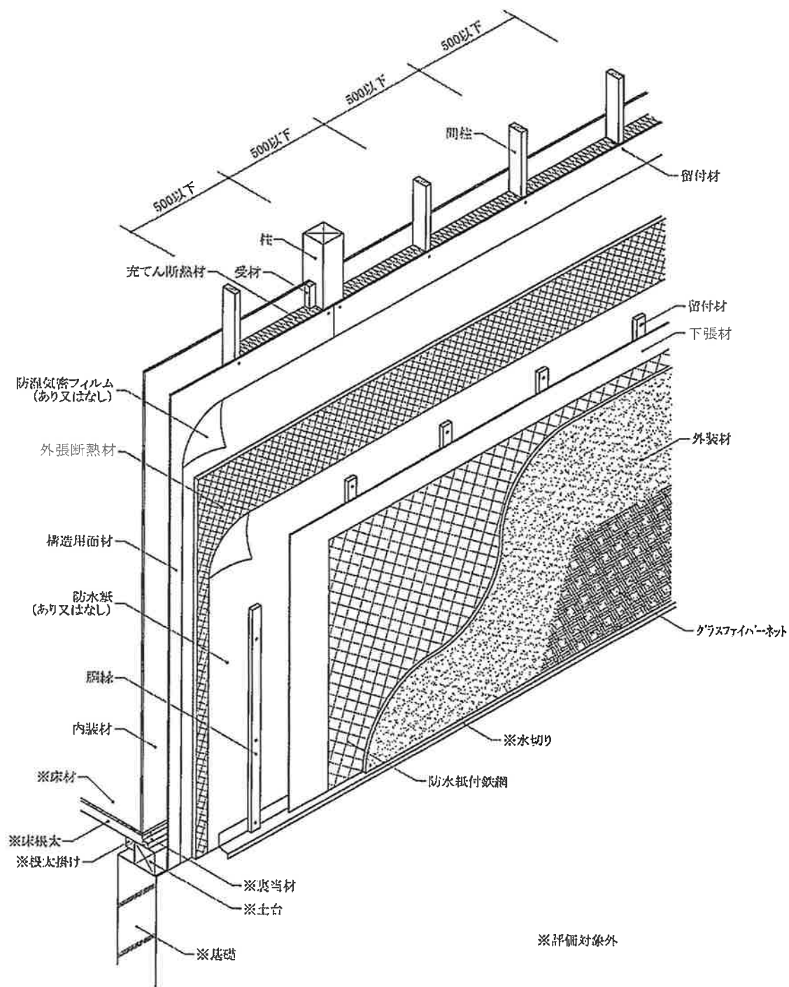
透視図
