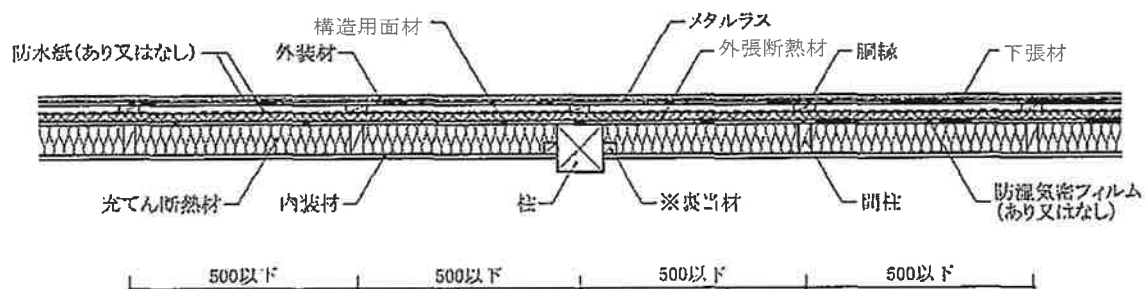
水平断面図
