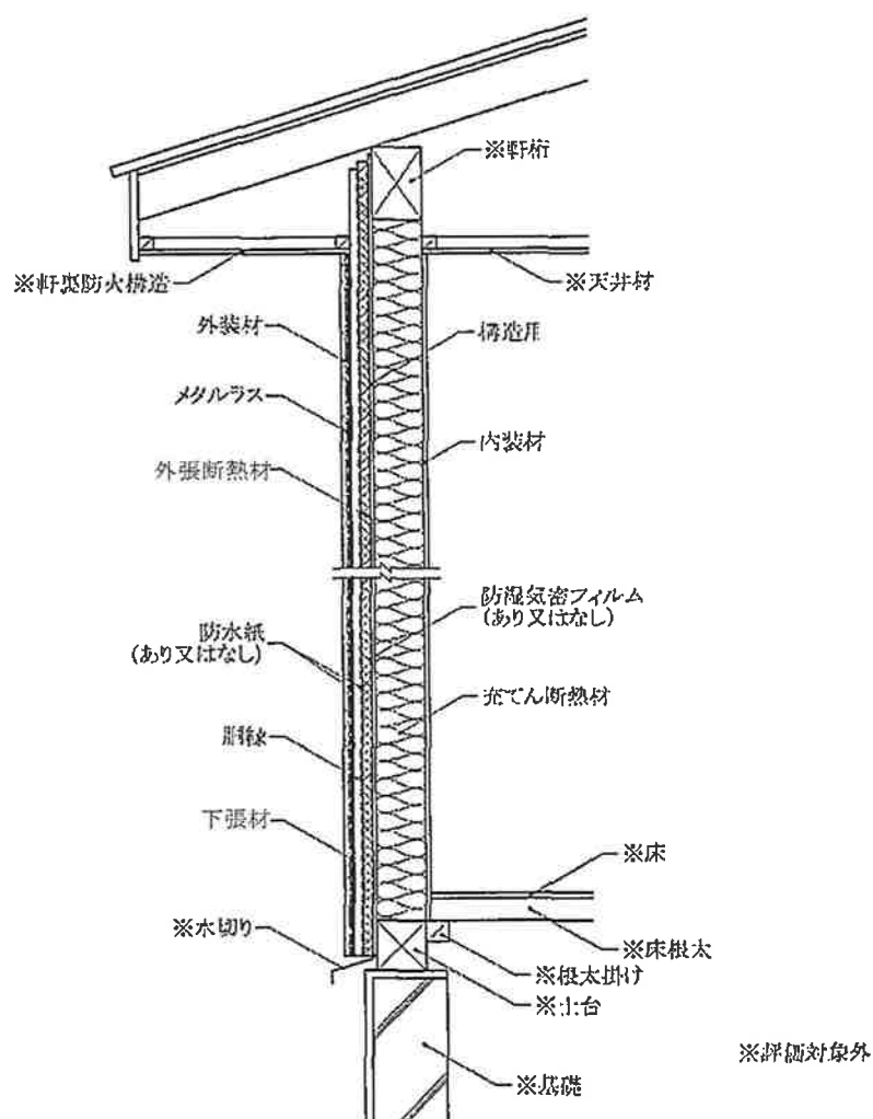
鉛直断面図
