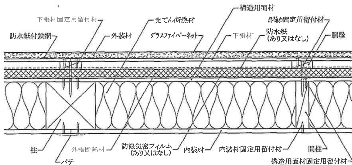
水平断面図
