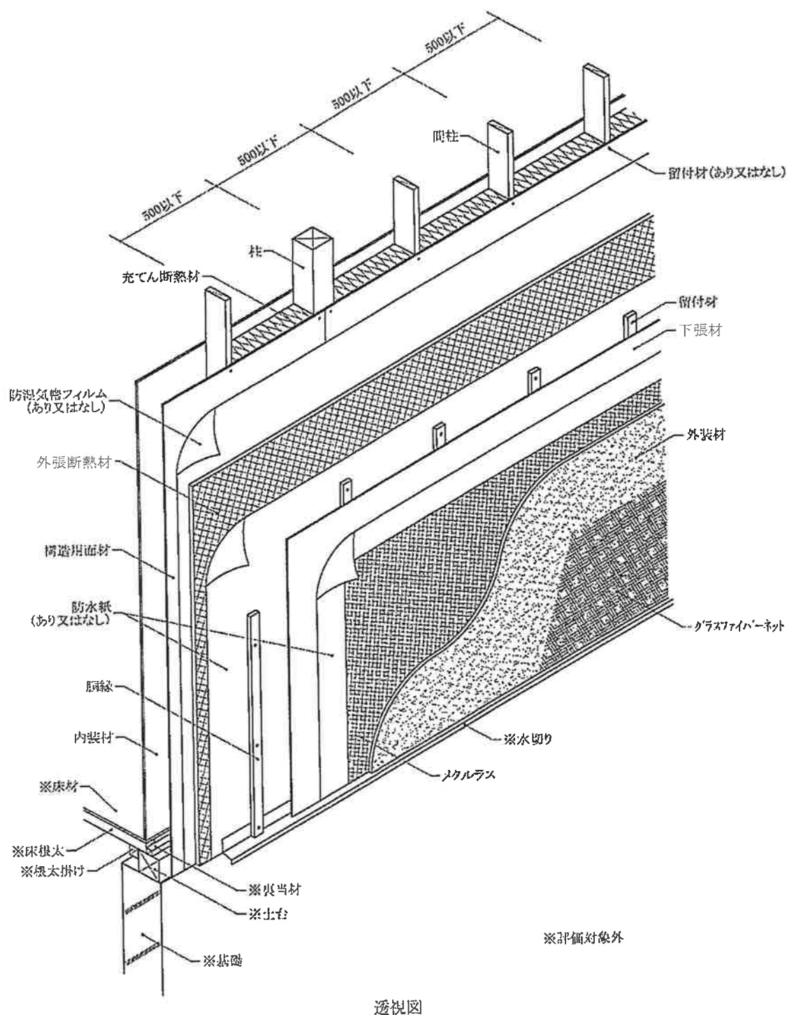
図11 構造説明図 (充てん断熱材あり／構造用面材あり／下張材あり)
