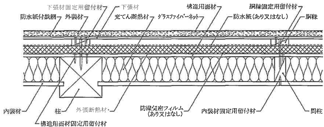
水平断面図
