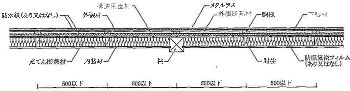
水平断面図
