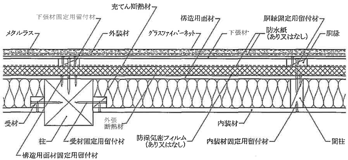
水平断面図
