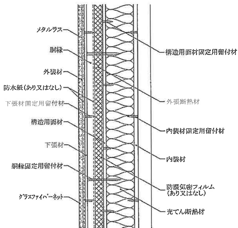
鉛直断面図
