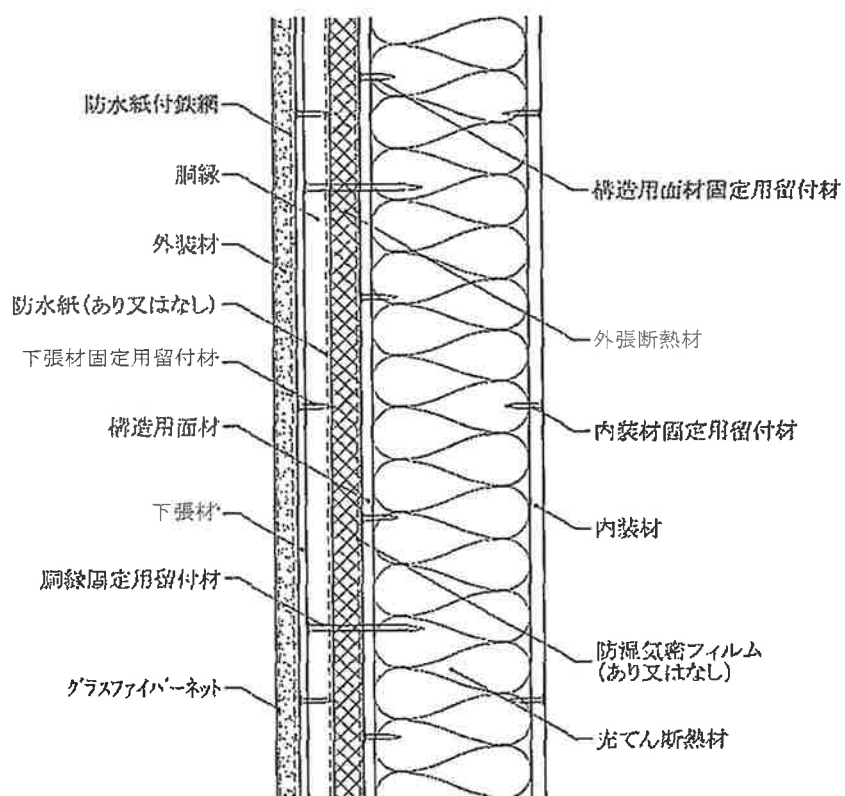
鉛直断面図
