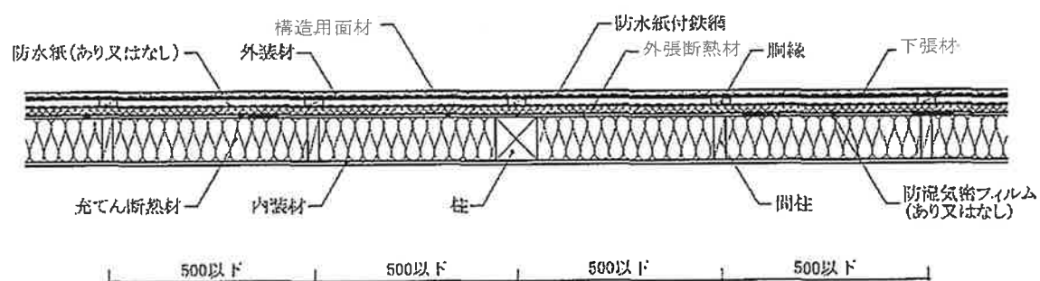
水平断面図
