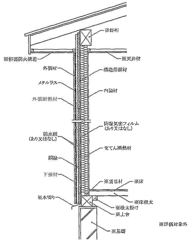
鉛直断面図
