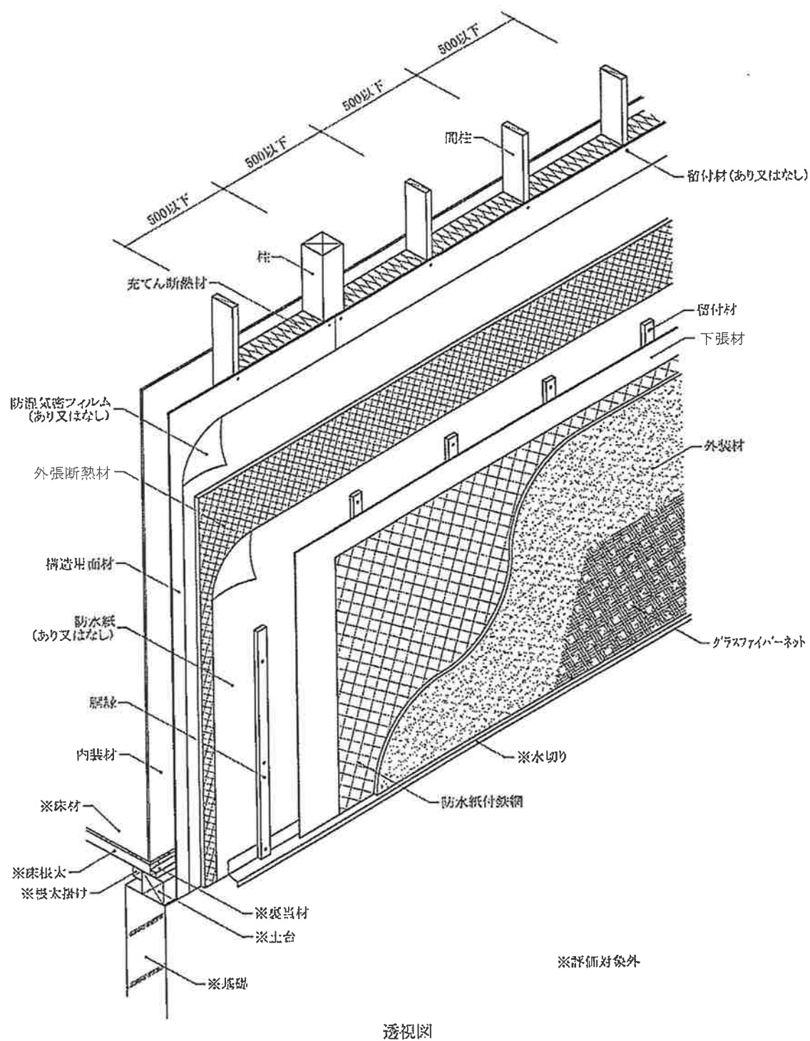
図9 構造説明図 (充てん断熱材あり／構造用面材あり／下張材あり)
