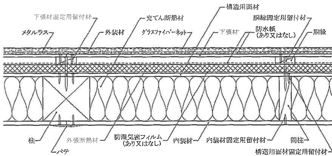
水平断面図
