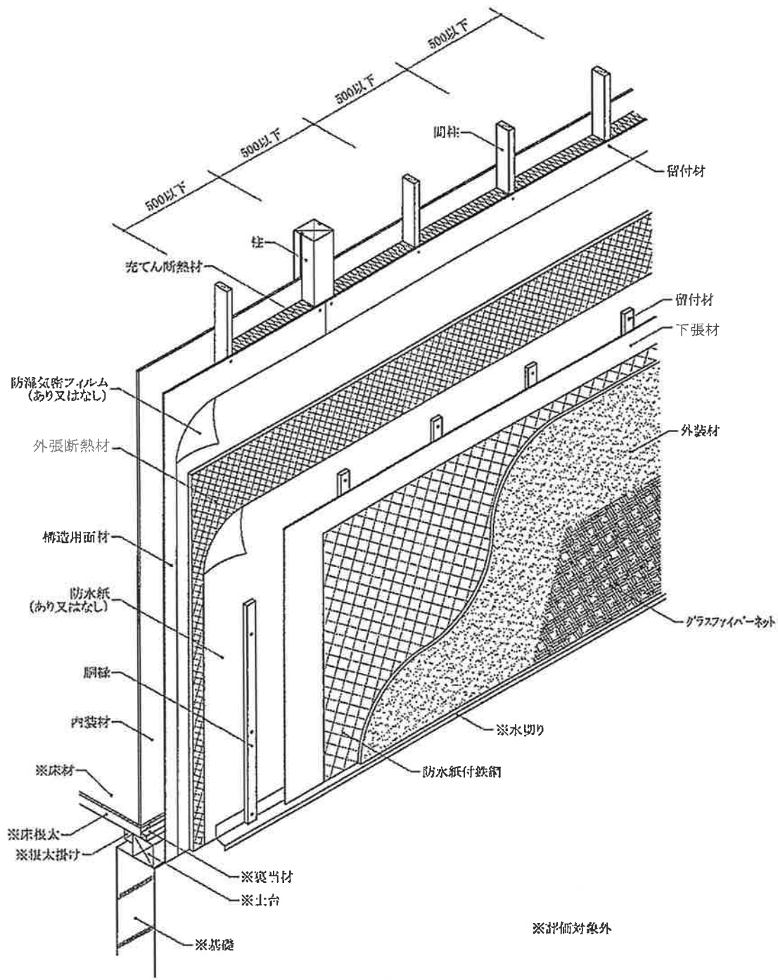
透視図
