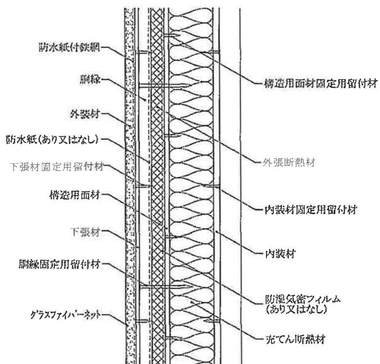
鉛直断面図
