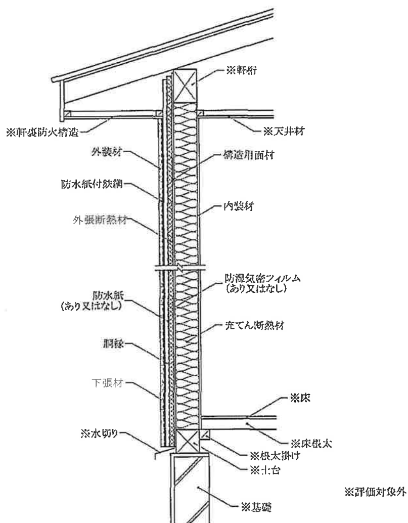
鉛直断面図
