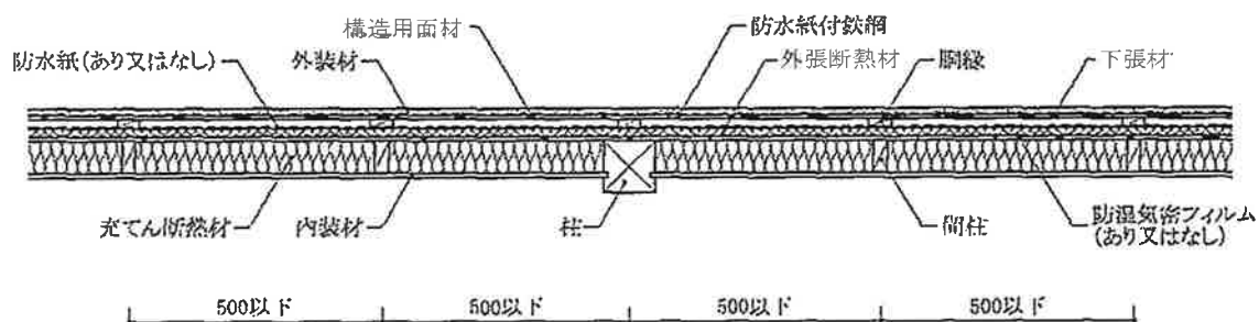
水平断面図
