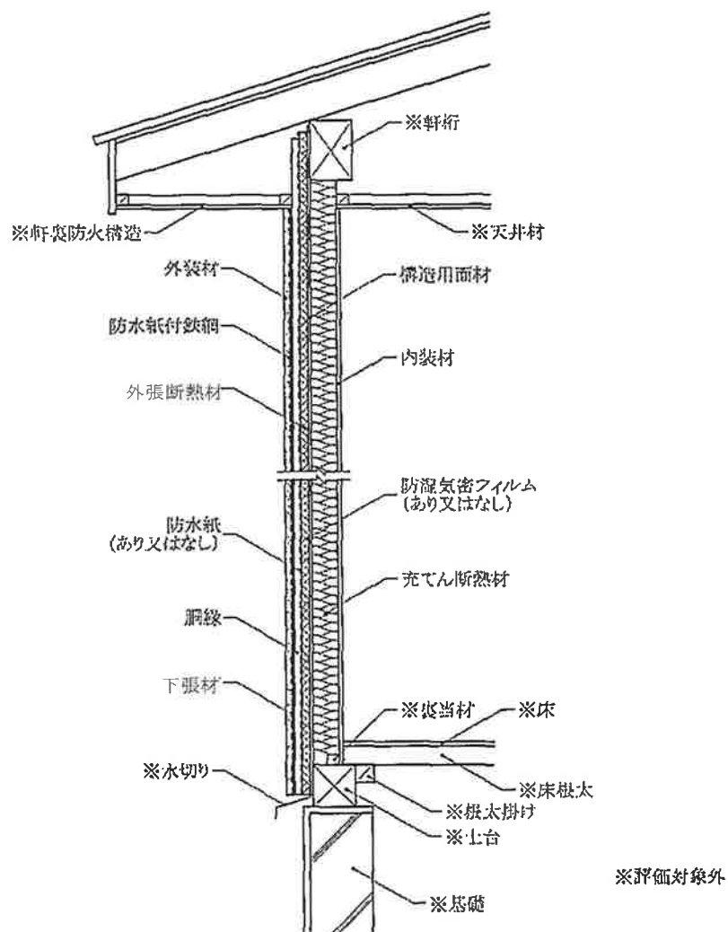
鉛直断面図
