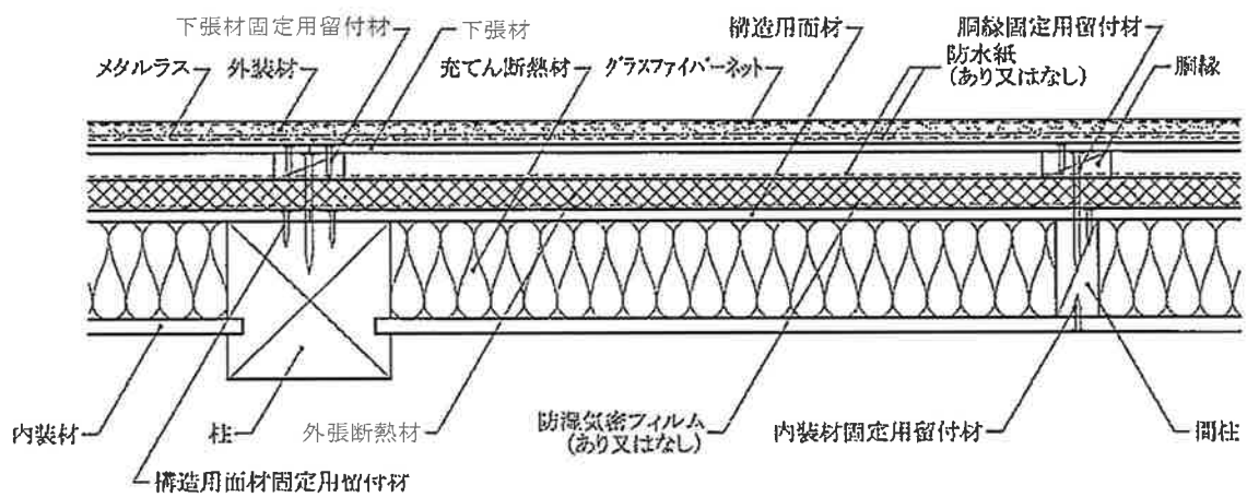
水平断面図
