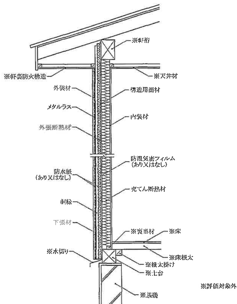
鉛直断面図
