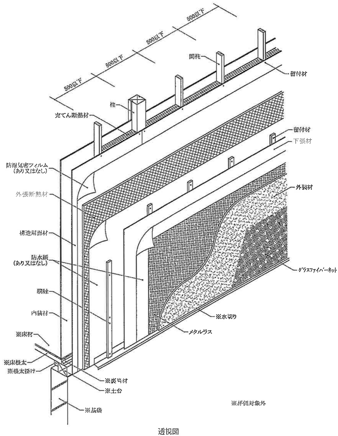
図3 構造説明図 (充てん断熱材あり／構造用面材あり／下張材あり)
