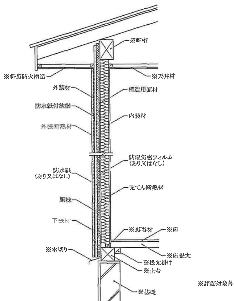
鉛直断面図
