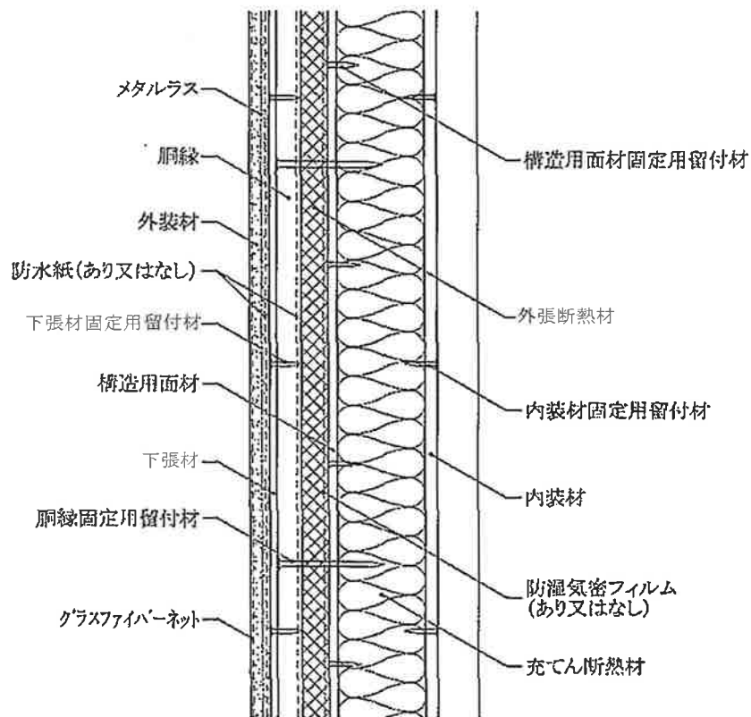
鉛直断面図
