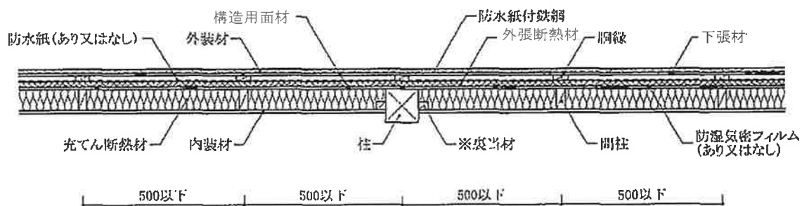
水平断面図
