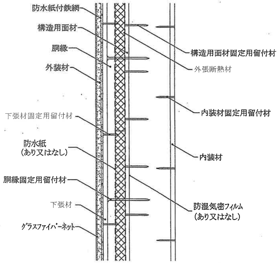
鉛直断面図
