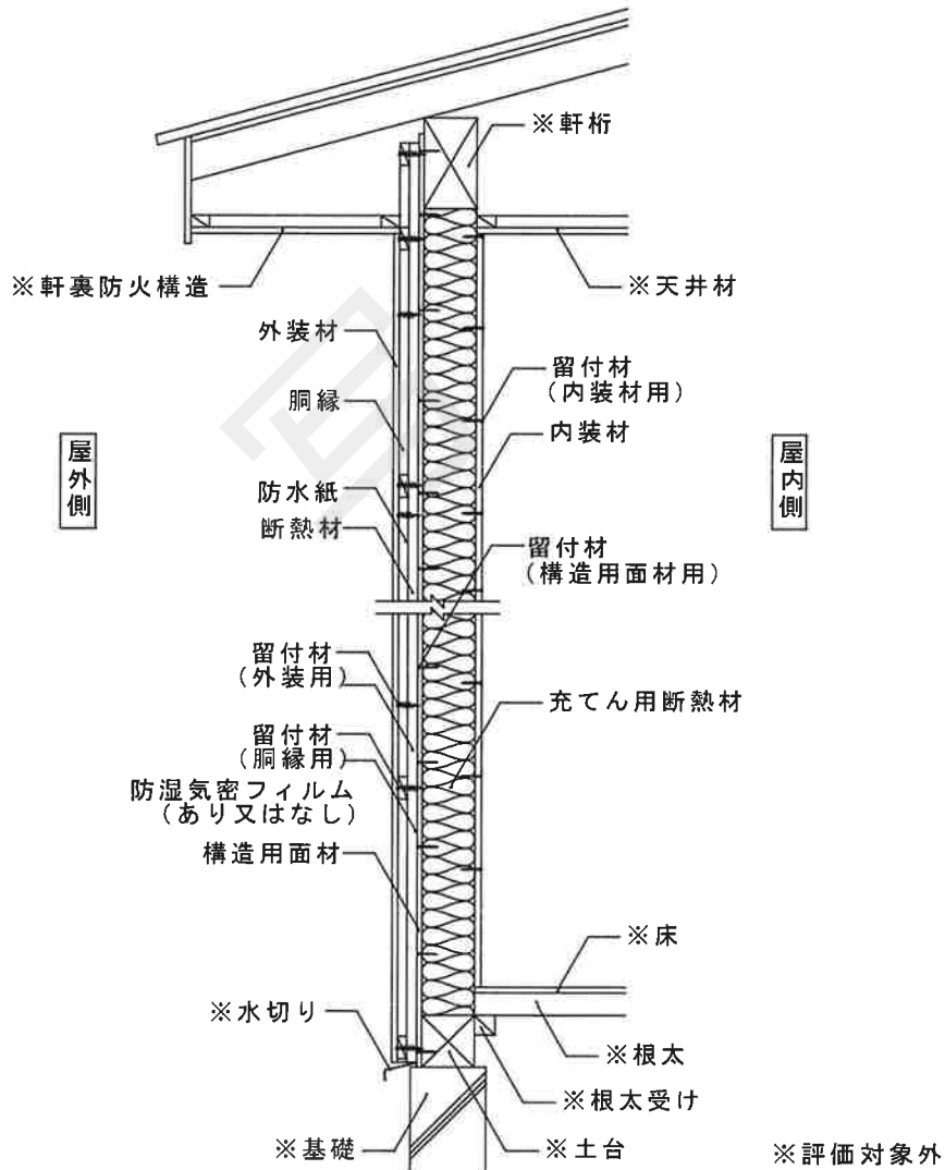
鉛直断面図
