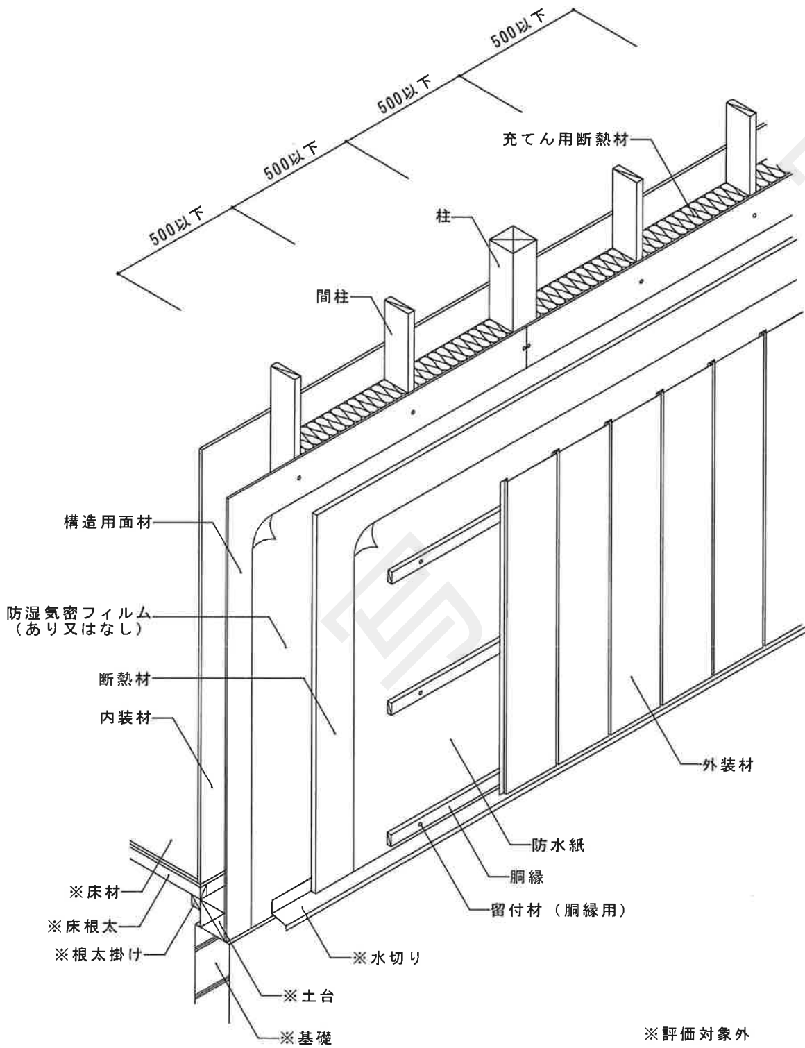
透視図
