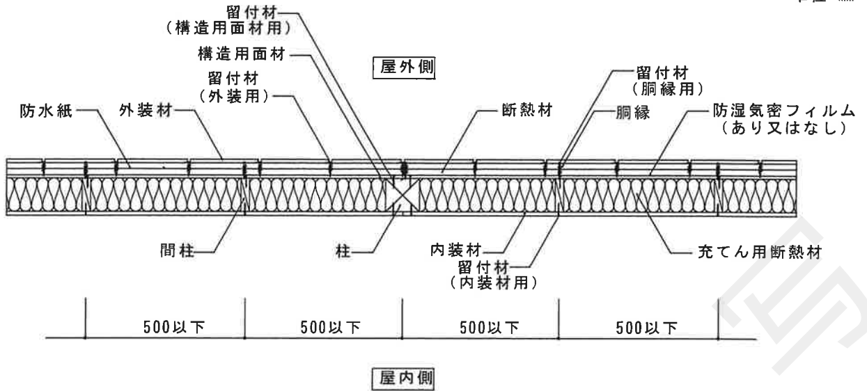
水平断面図
