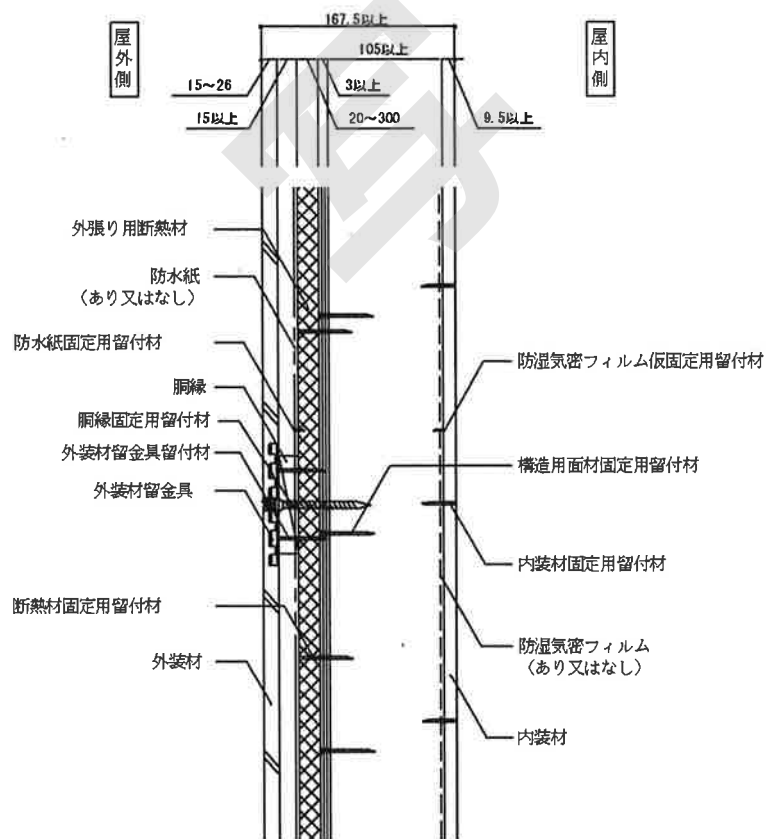
鉛直断面詳細図
