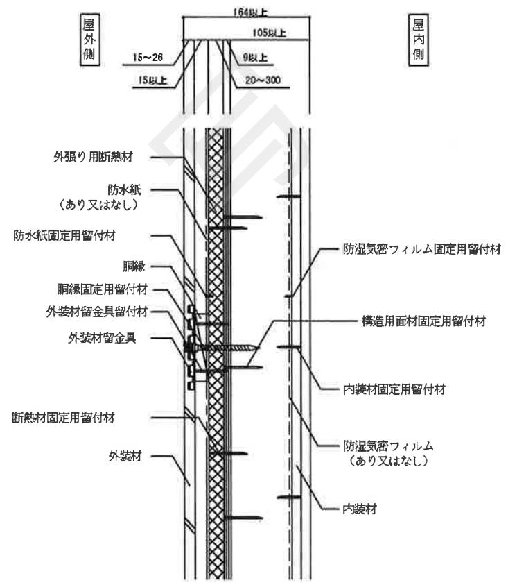
鉛直断面詳細図
