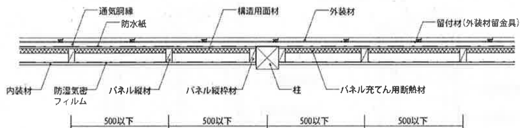
水平断面図
