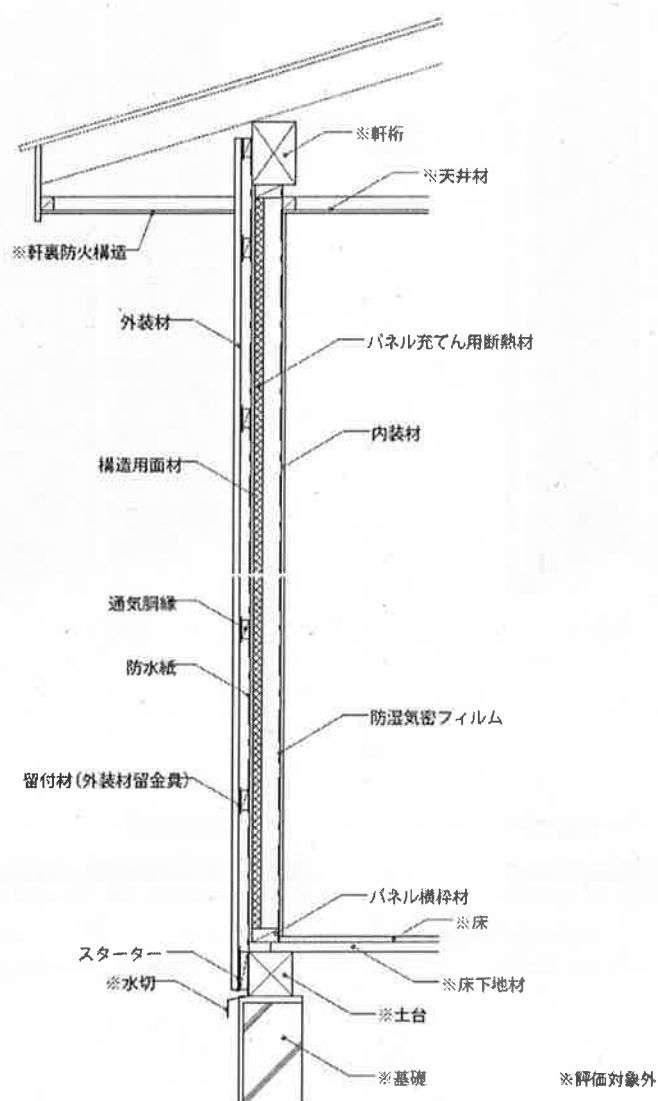
鉛直断面図
