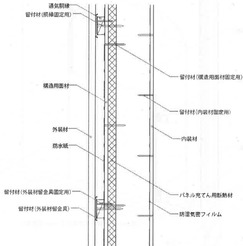
鉛直断面図
