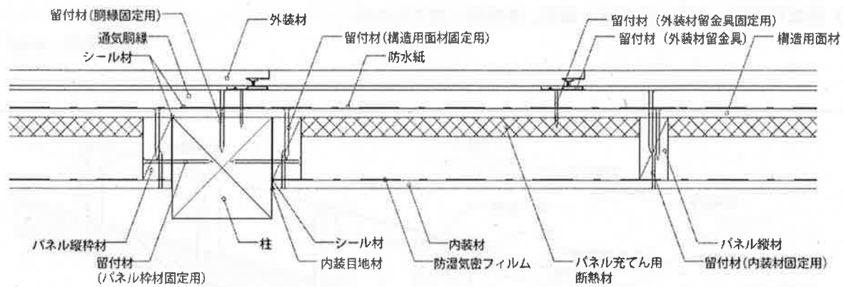
水平断面図
