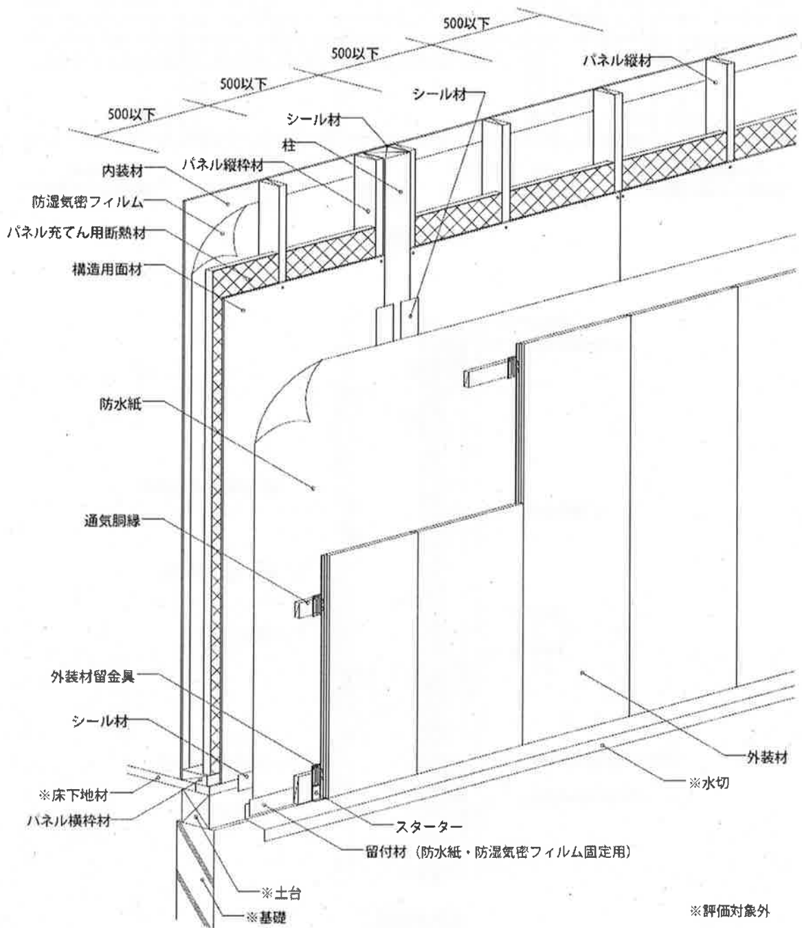
透視図
