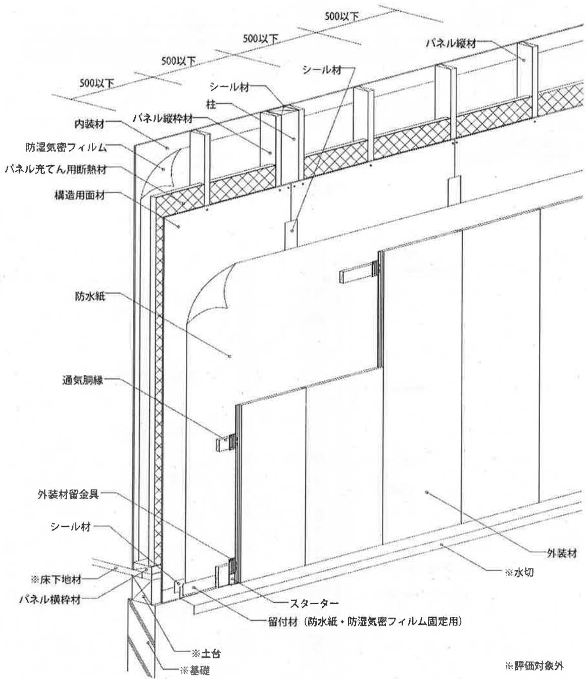
透視図
