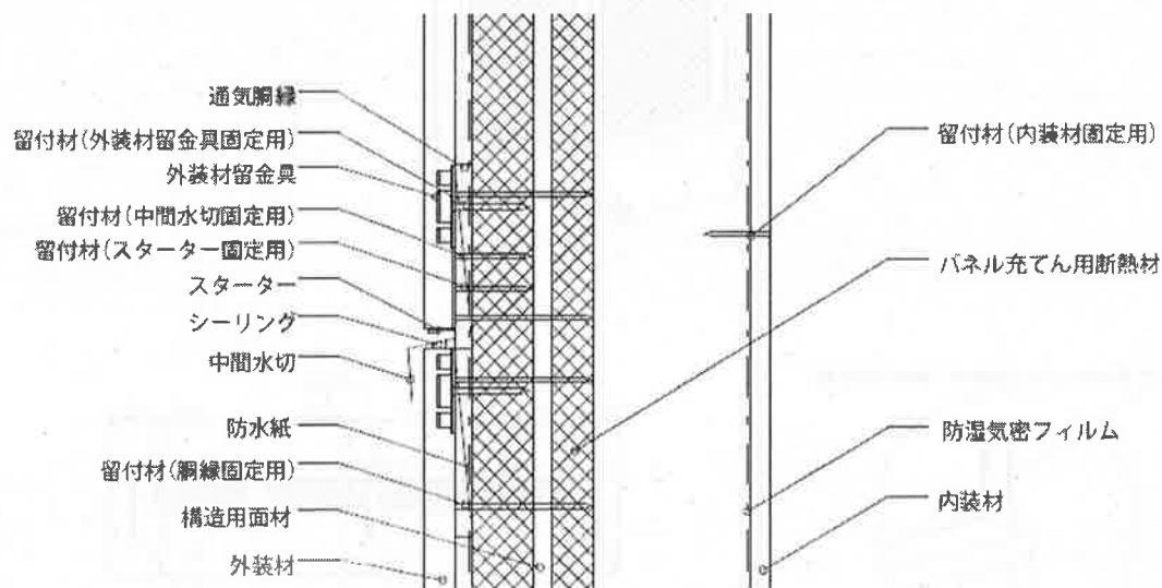
鉛直断面図
