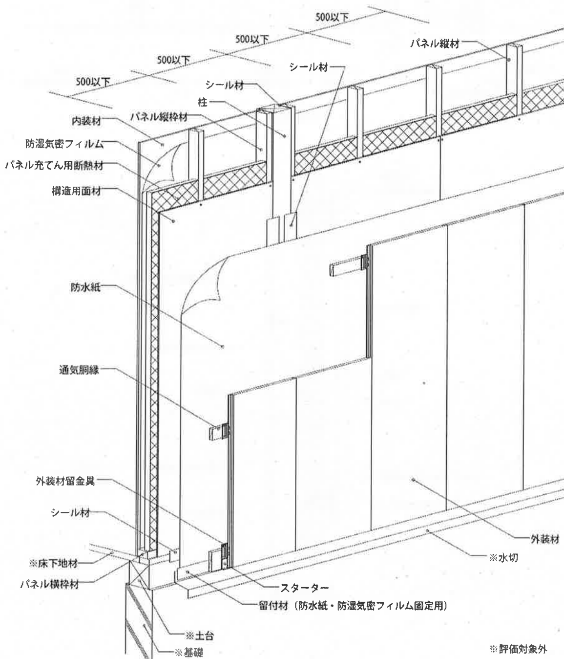
透視図
