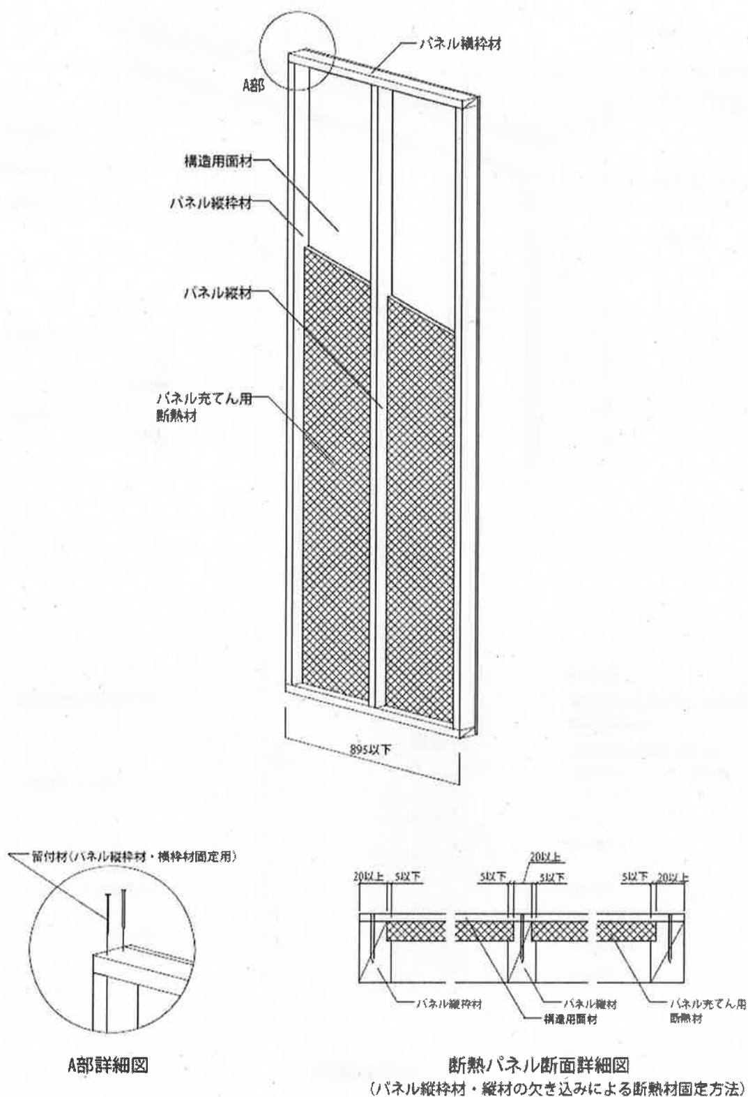
図 13 施工図
