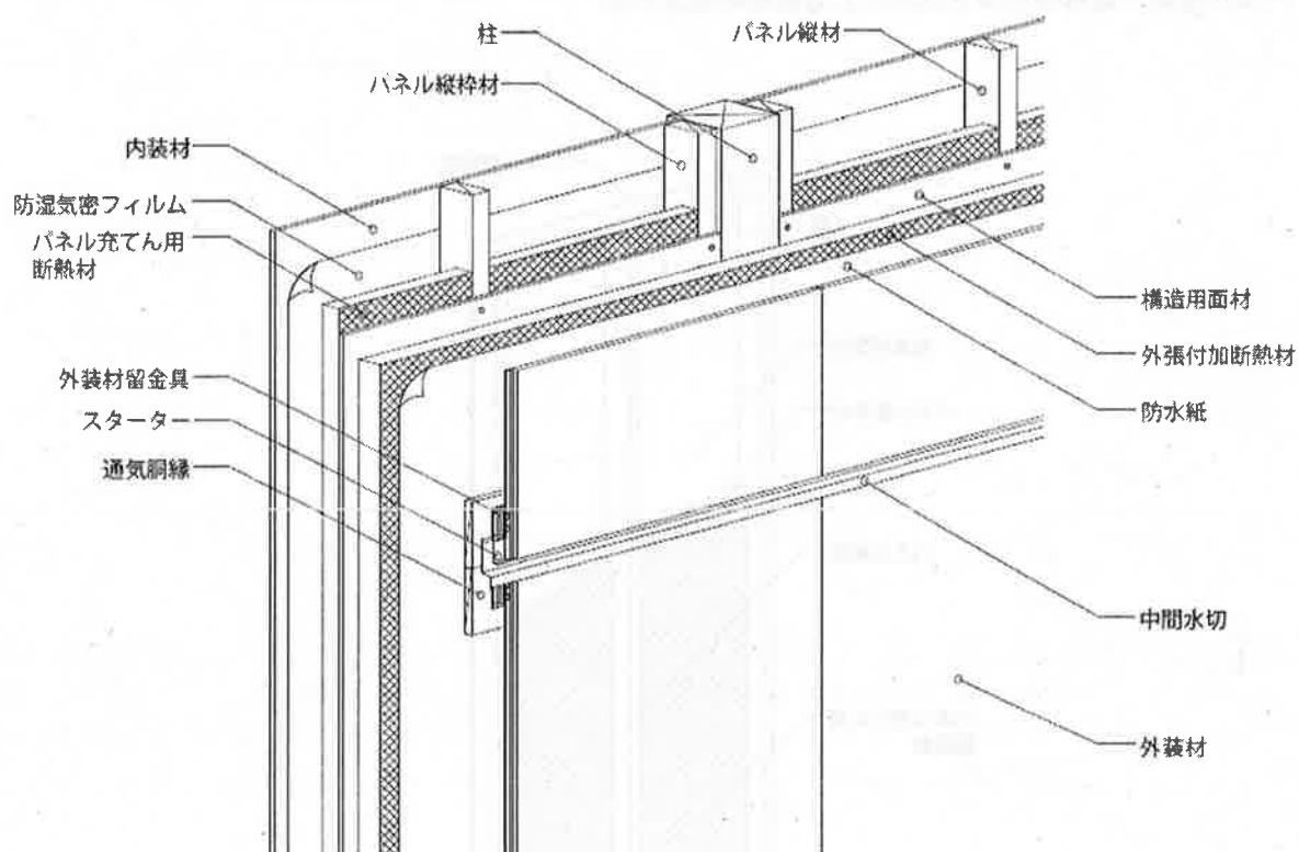
透視図
