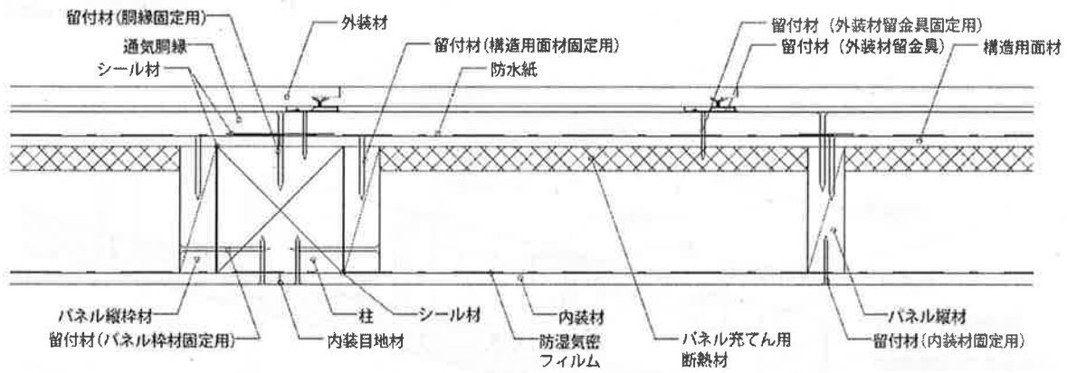
水平断面図
