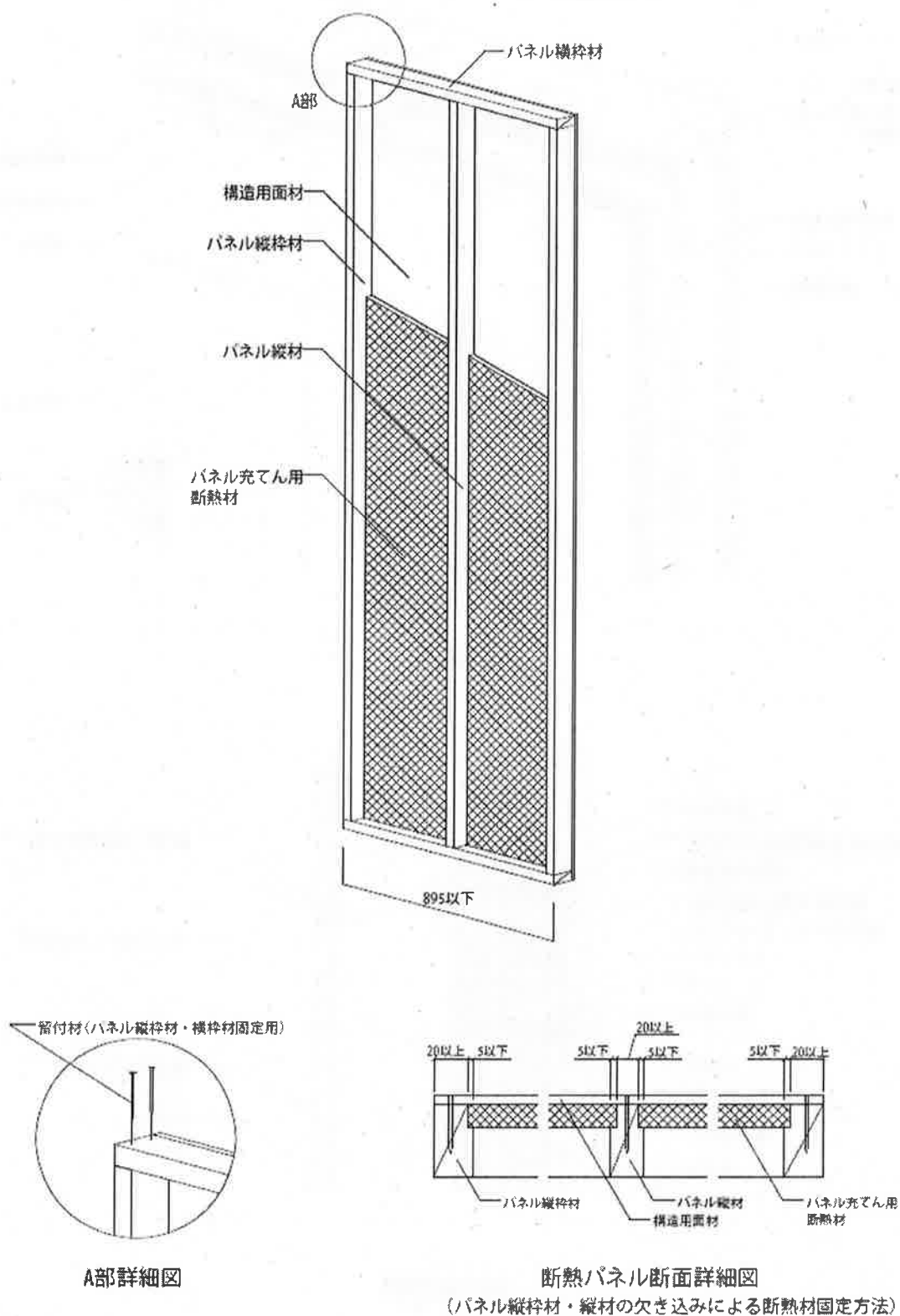
図 13 施工図
