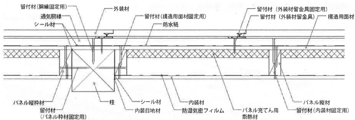
水平断面図
