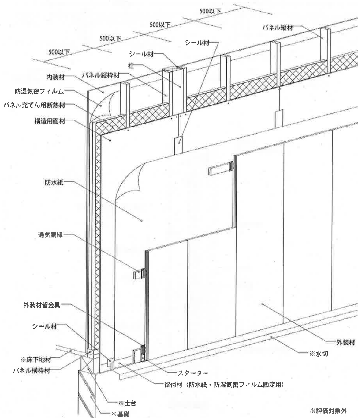
透視図
