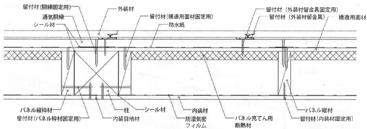
水平断面図
