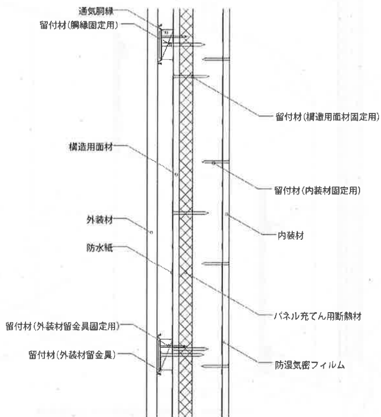
鉛直断面図
