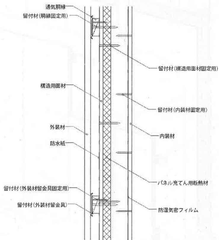
鉛直断面図
