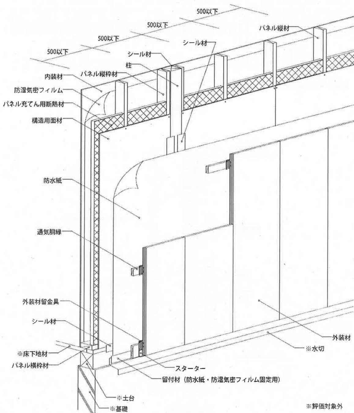
透視図
