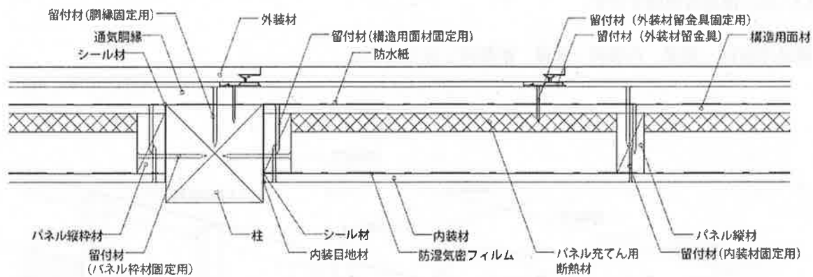
水平断面図
