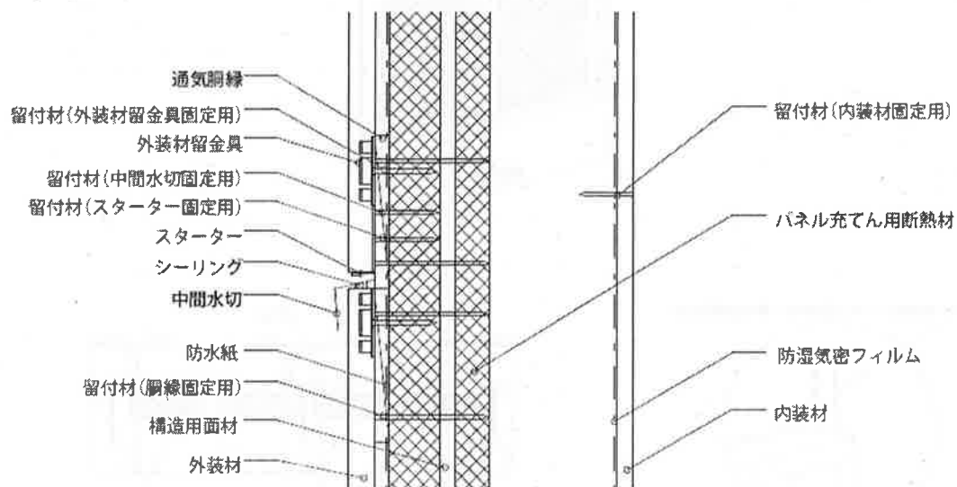
鉛直断面図
