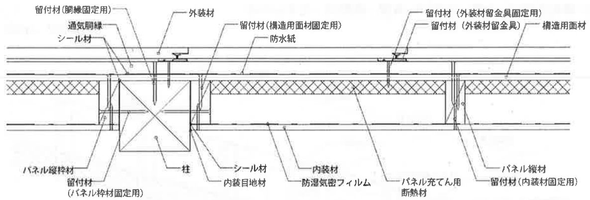
水平断面図
