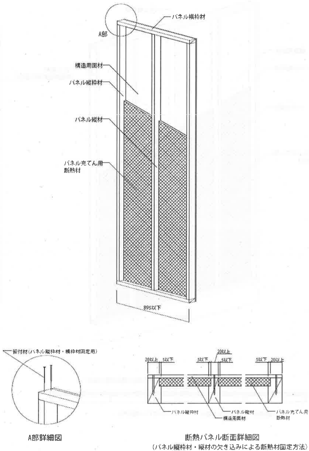
図 22 施工図
