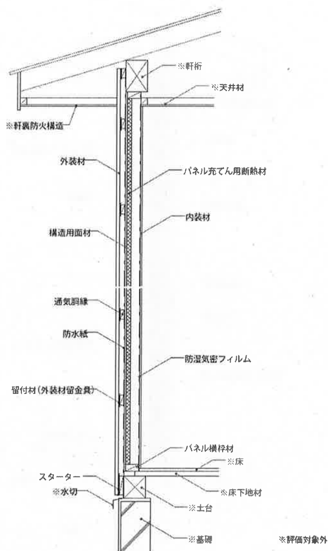
鉛直断面図
