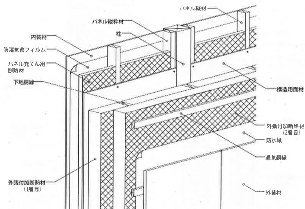
透視図
