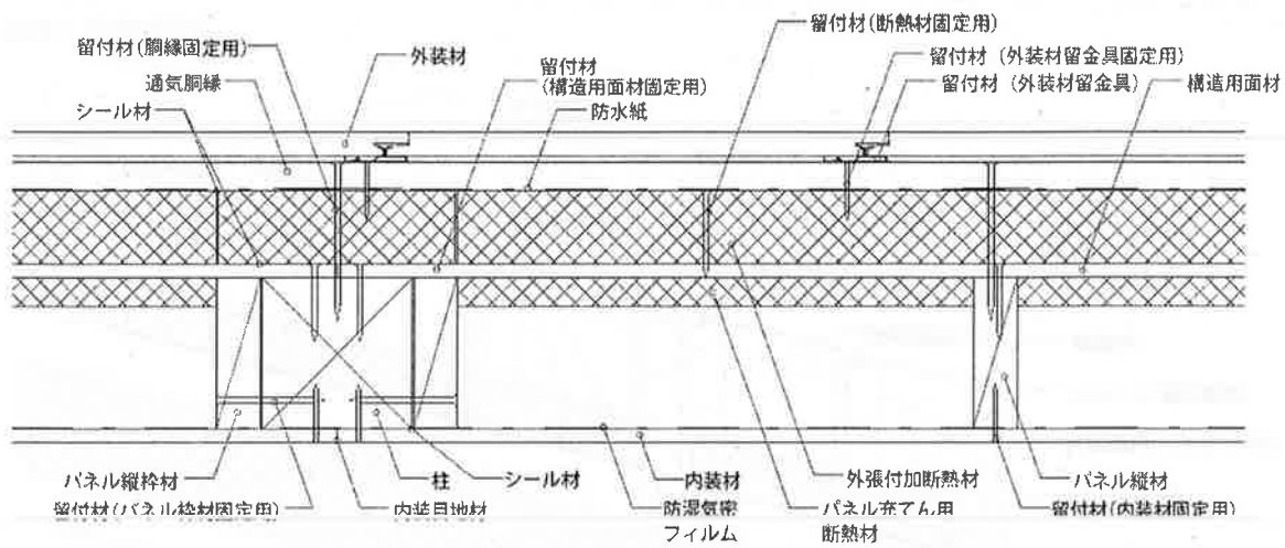
水平断面図
