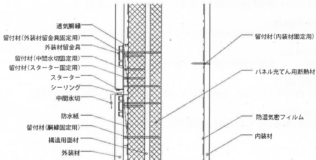
鉛直断面図
