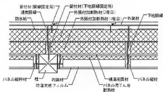
水平断面図
