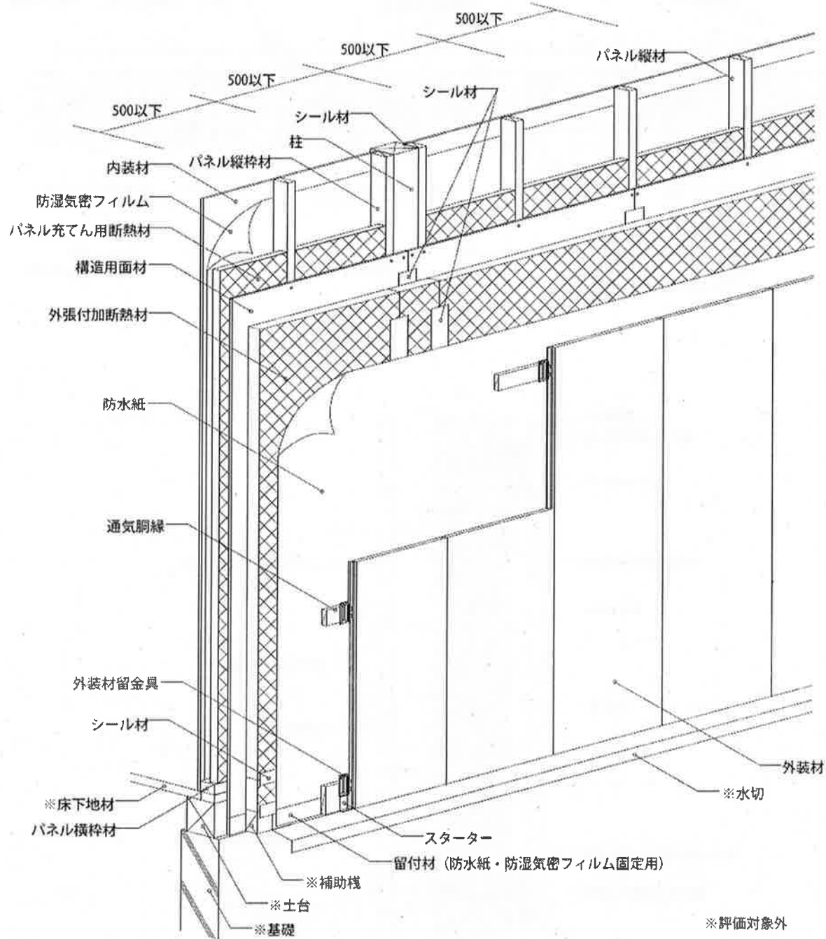
透視図
