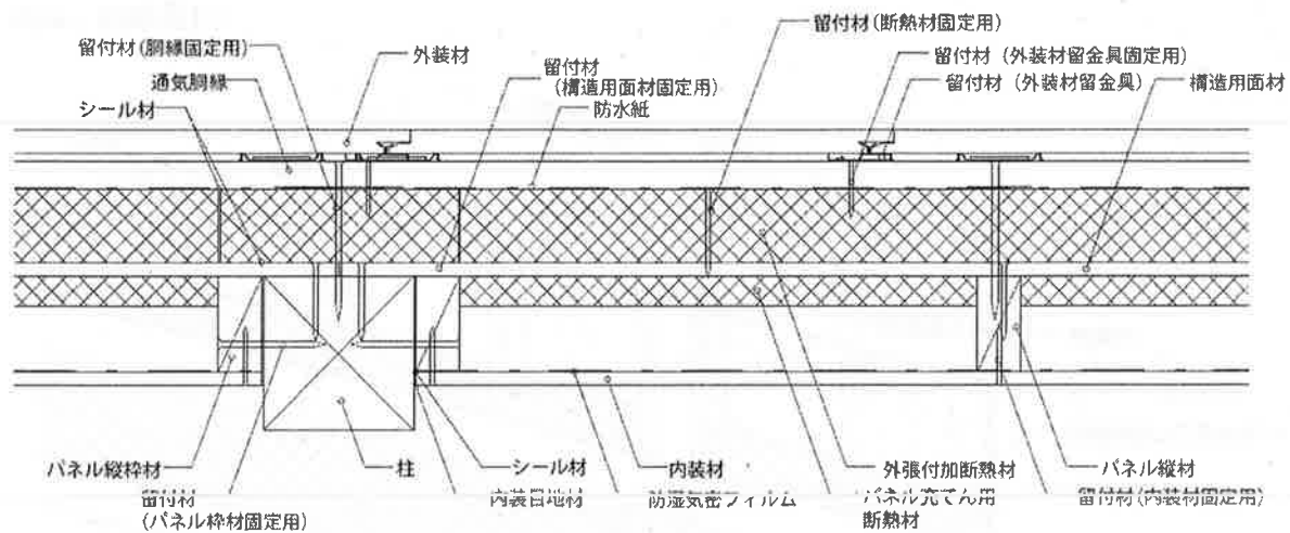
水平断面図
