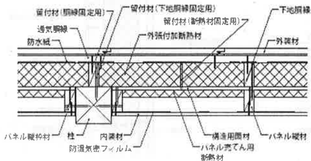
水平断面图
