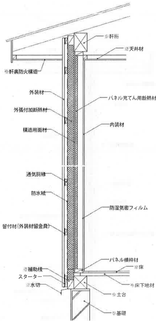
鉛直断面図
