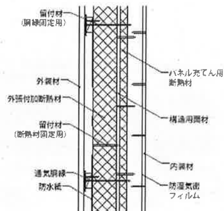
鉛直断面図
