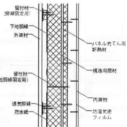
鉛直断面図
