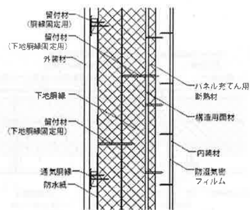
鉛直断面図
