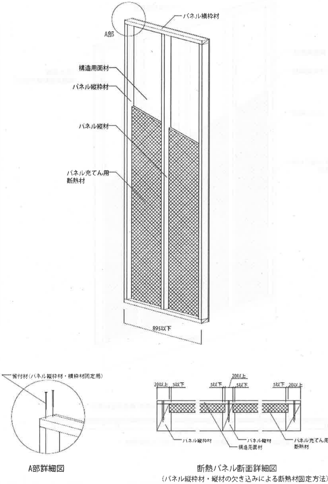
図 22 施工図
