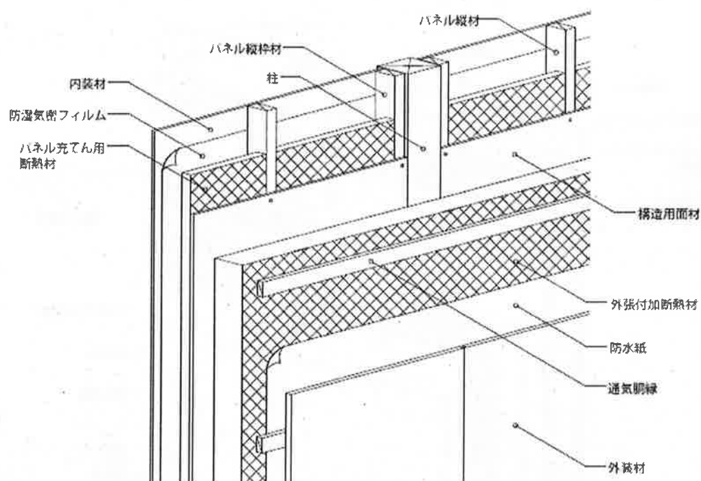
透視図
