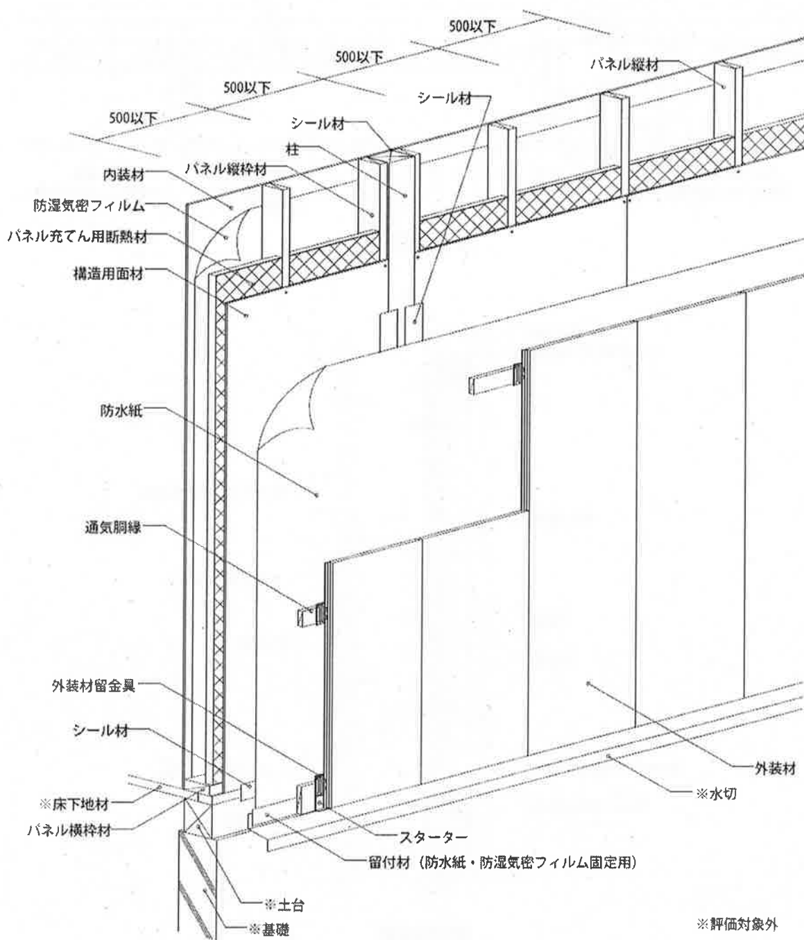
透視圖
