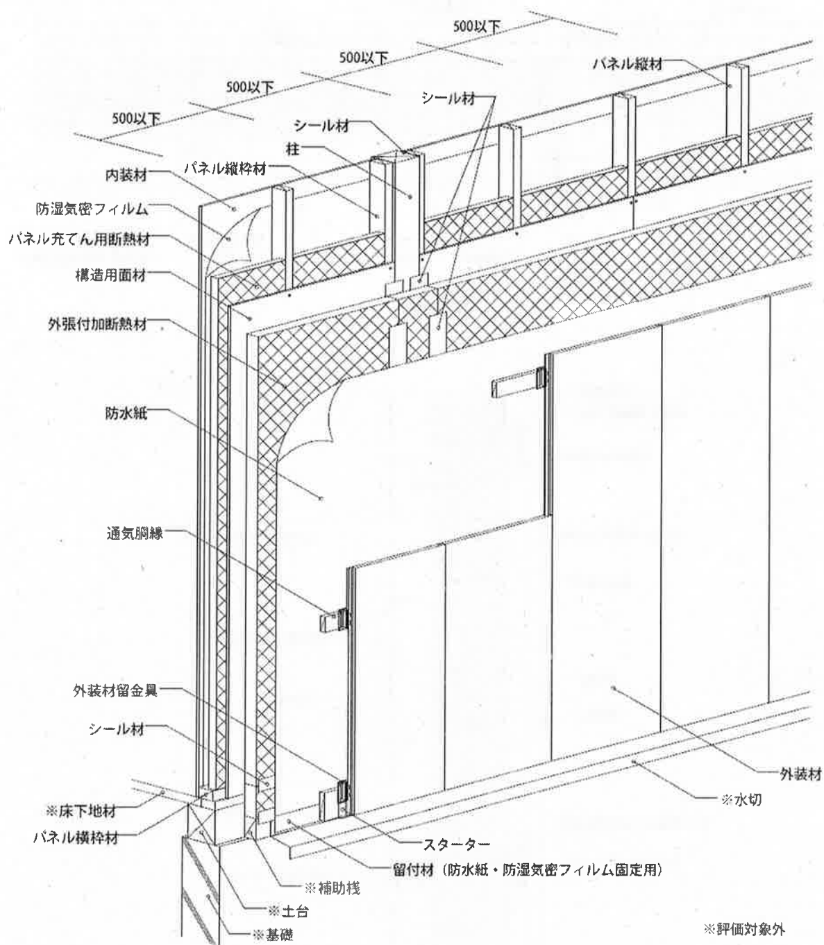
透視圖
