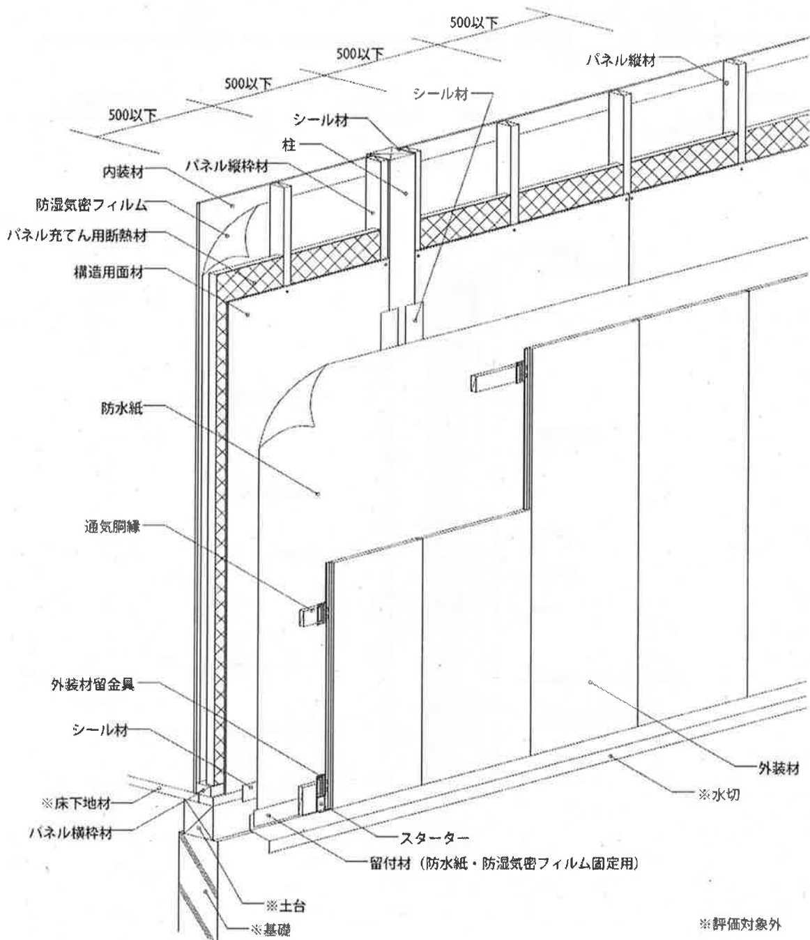
透視図
