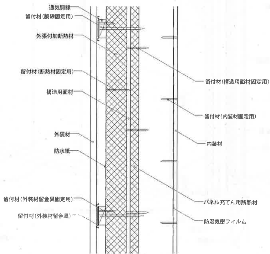
鉛直断面図
