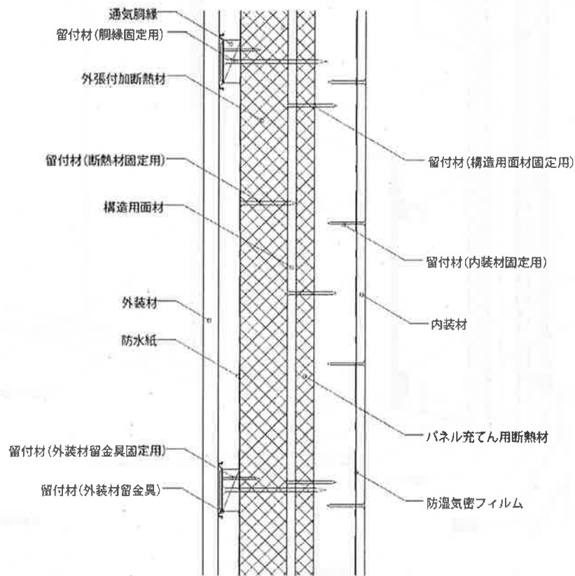
鉛直断面図
