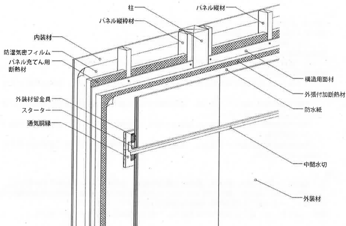
透視図
