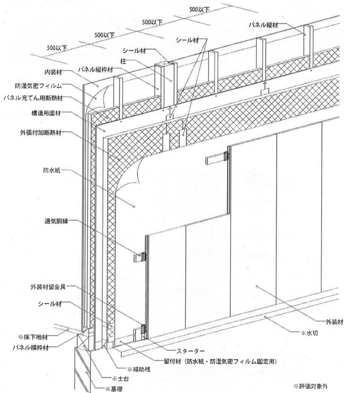
透視図
