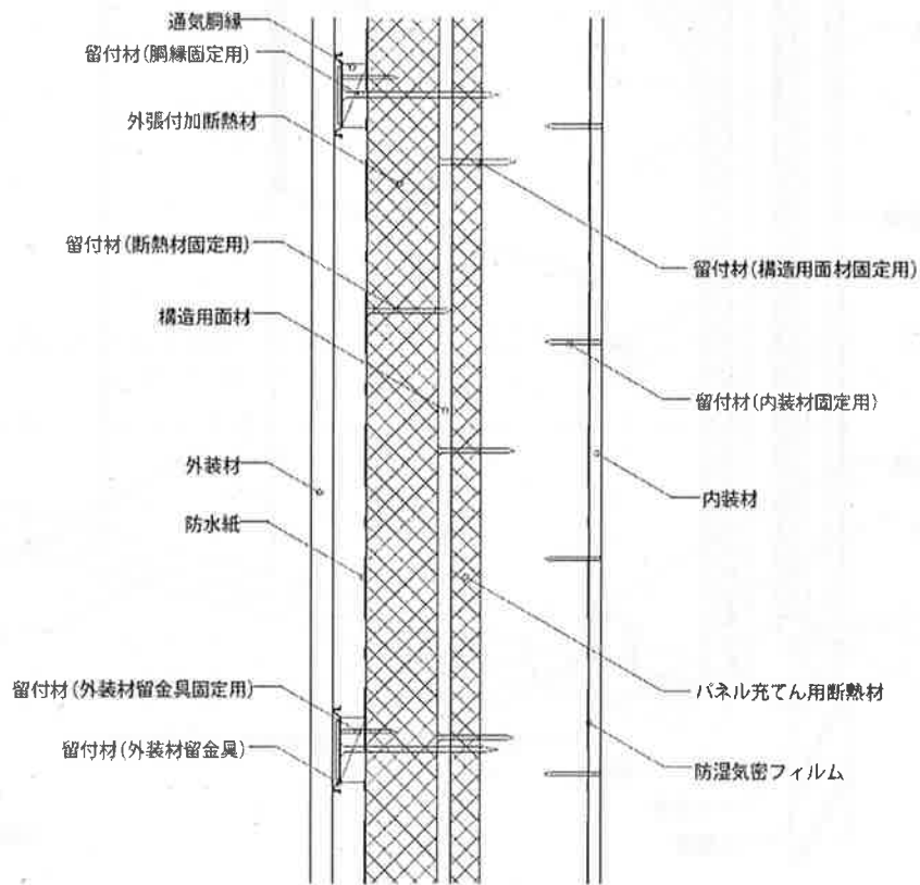
鉛直断面図
