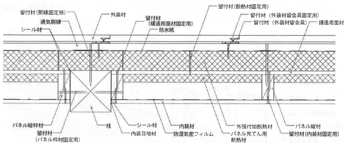
水平断面図
