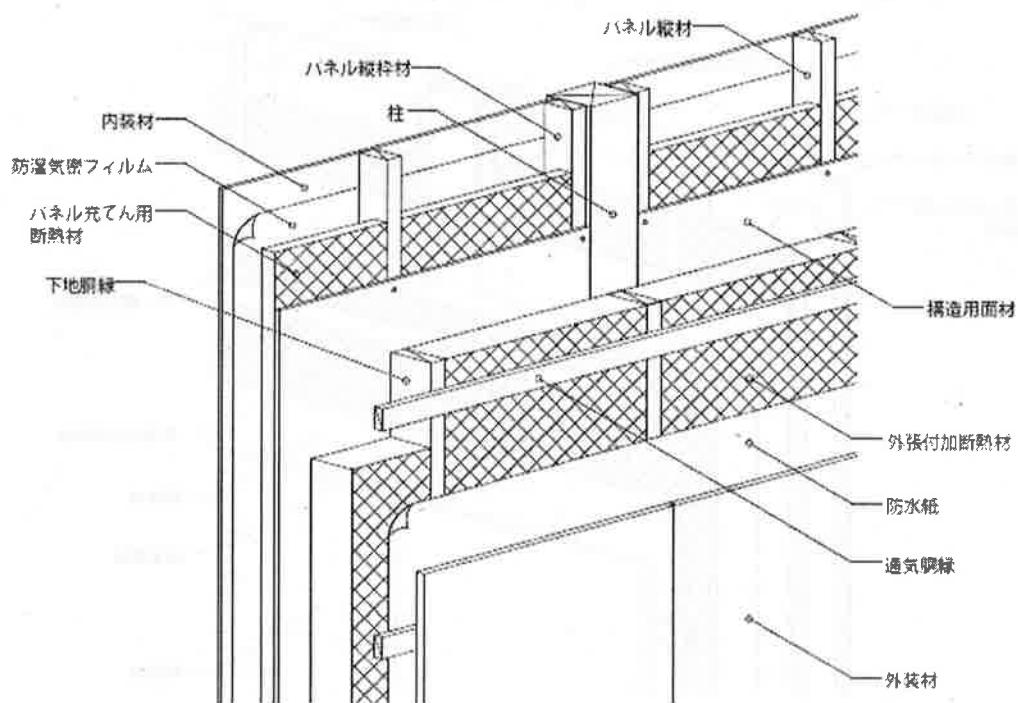
透視図
