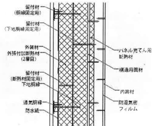
鉛直断面図
