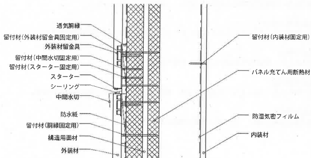
鉛直断面図
