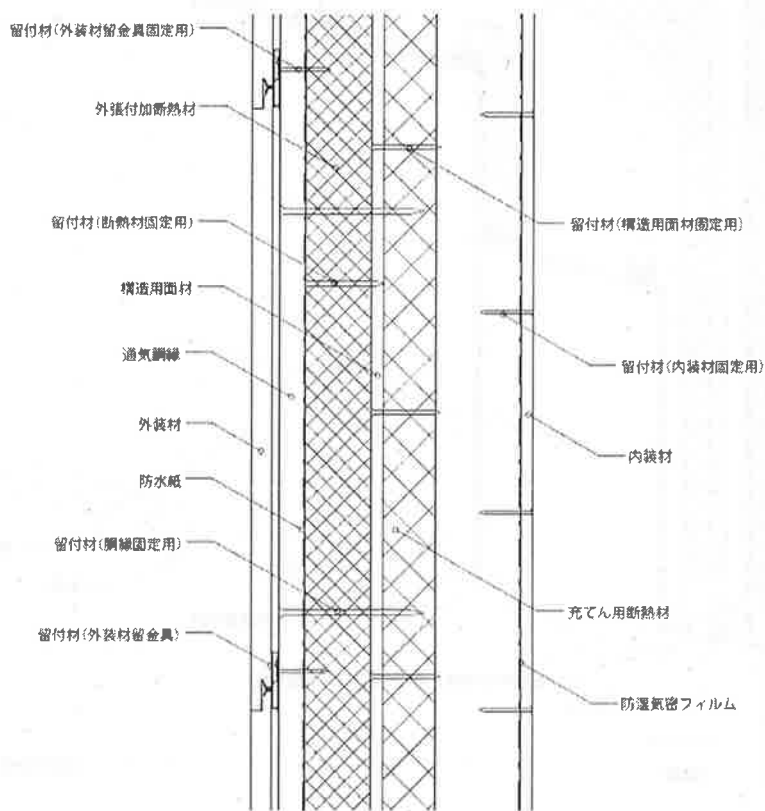
鉛直断面図
