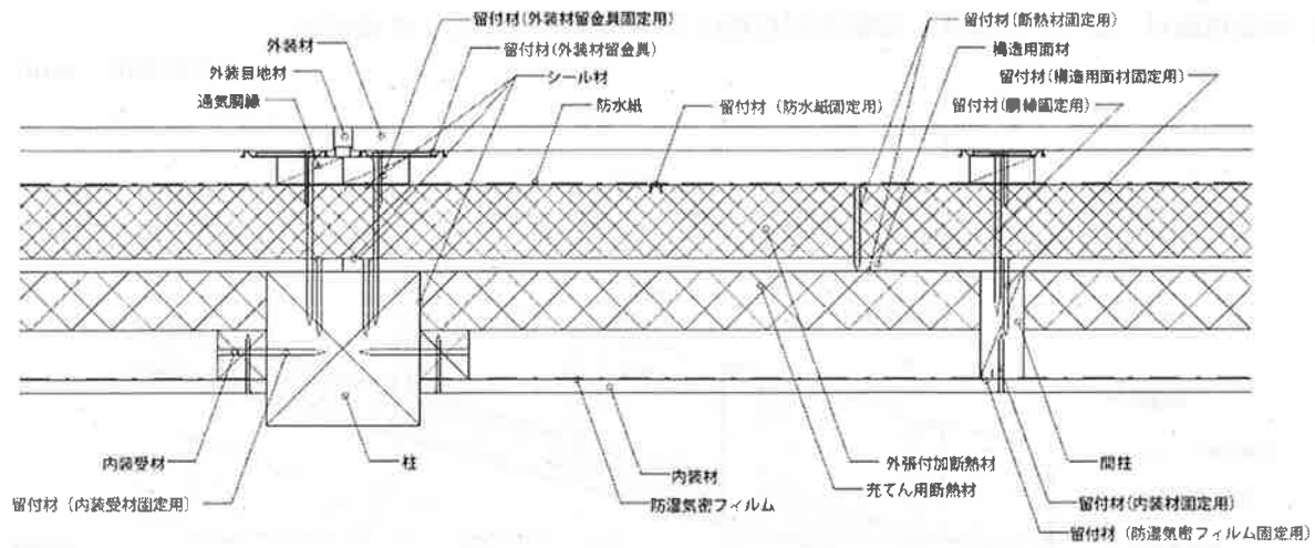
水平断面図
