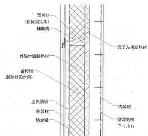
鉛直断面図
