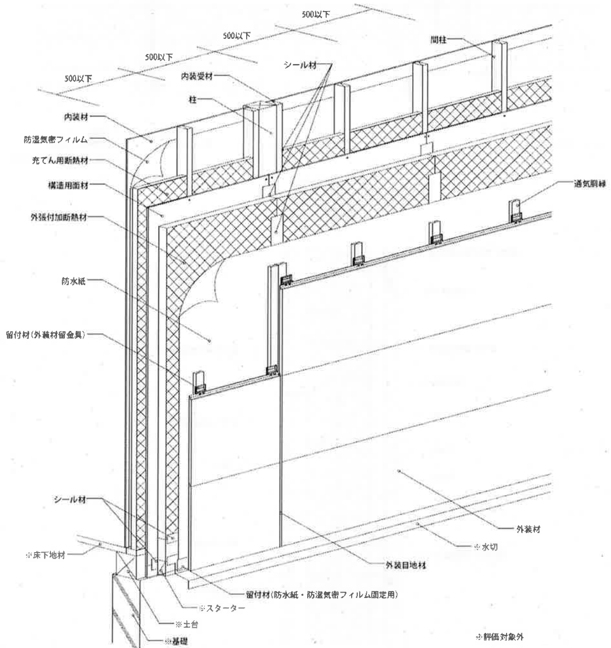
透視図
