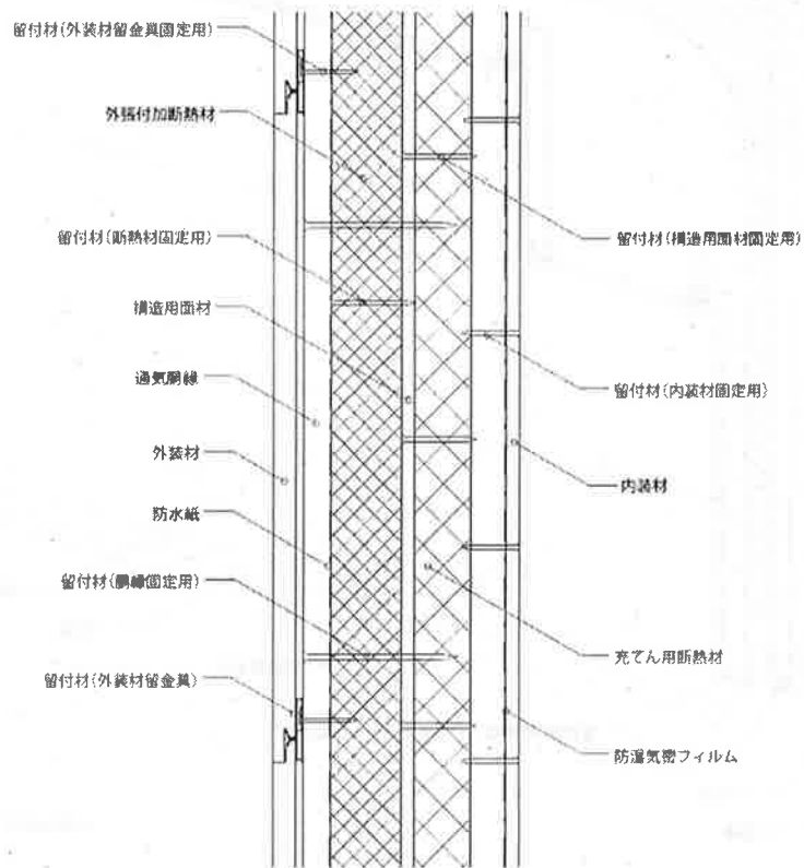
鉛直断面図
