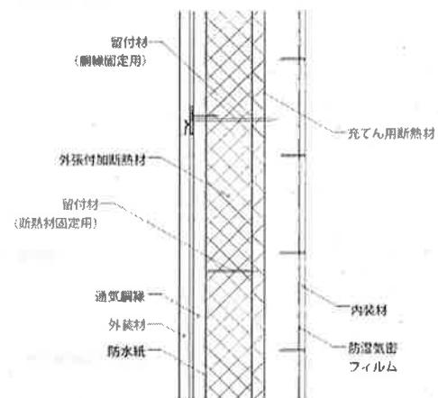
鉛直断面図
