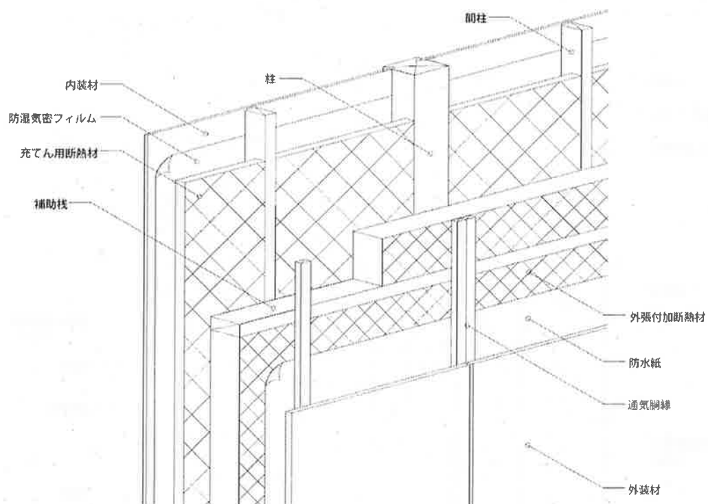
透視図
