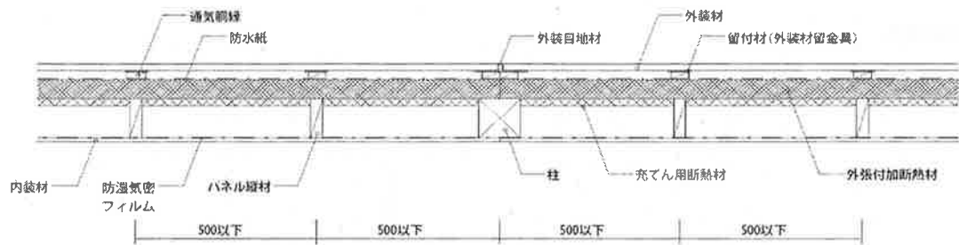
水平断面図
