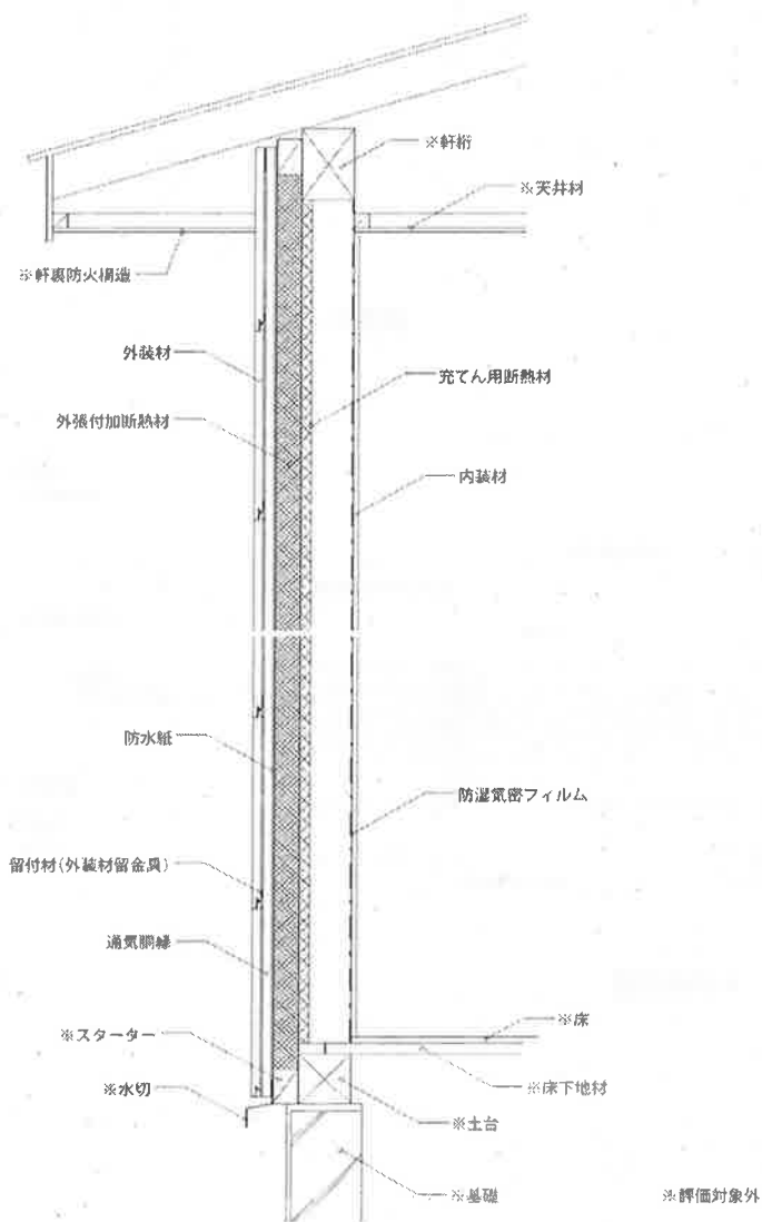
鉛直断面図
