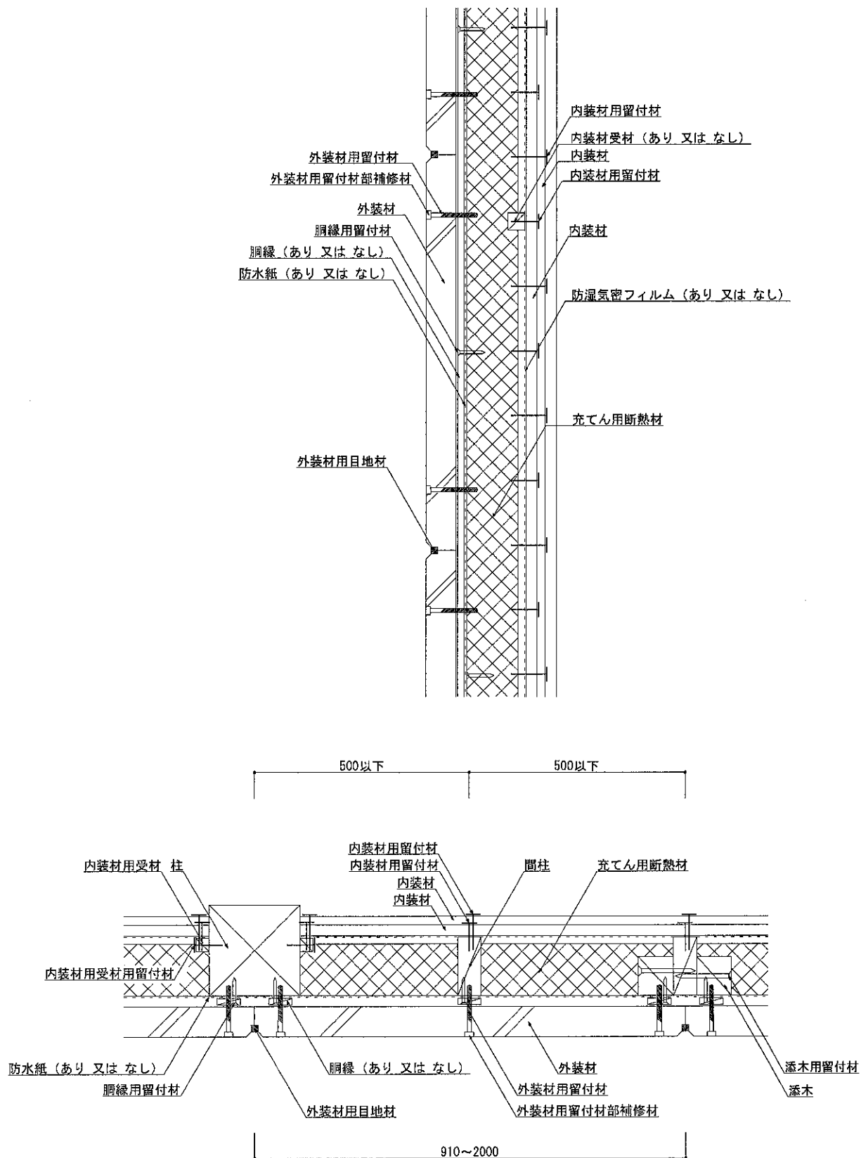
図4 構造説明図 (水平垂直断面詳細図・構造用面材なし／内装材真壁②(重張り))
