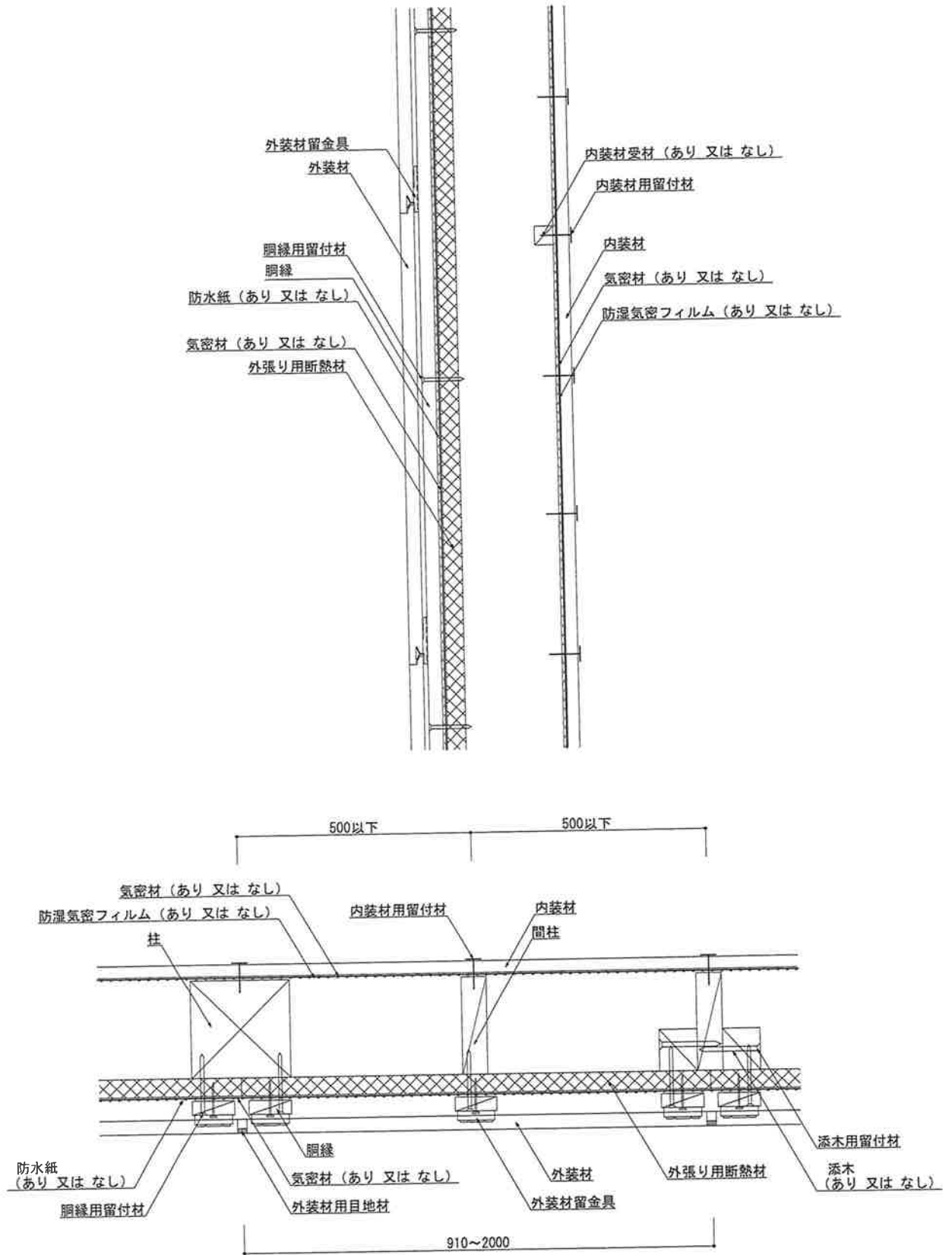
図2 構造説明図 (断面図・充てん断熱材なし/構造用面材なし/内装材大壁)
