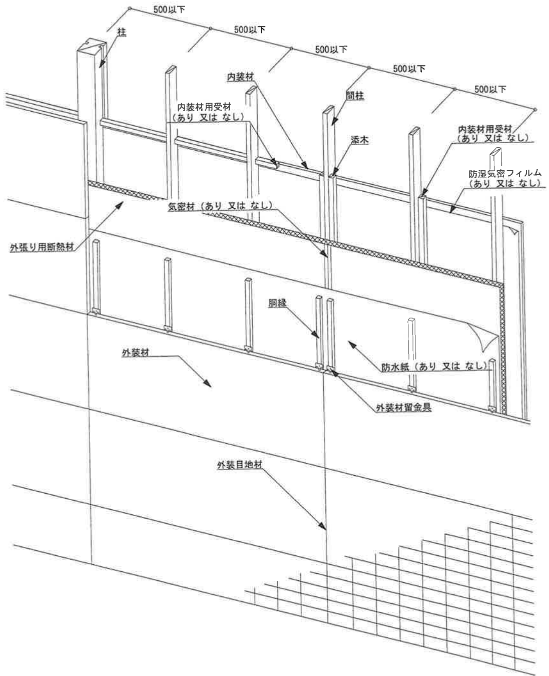
図3 構造説明図 (透視図・充てん断熱材なし/構造用面材なし/内装材真壁①)
