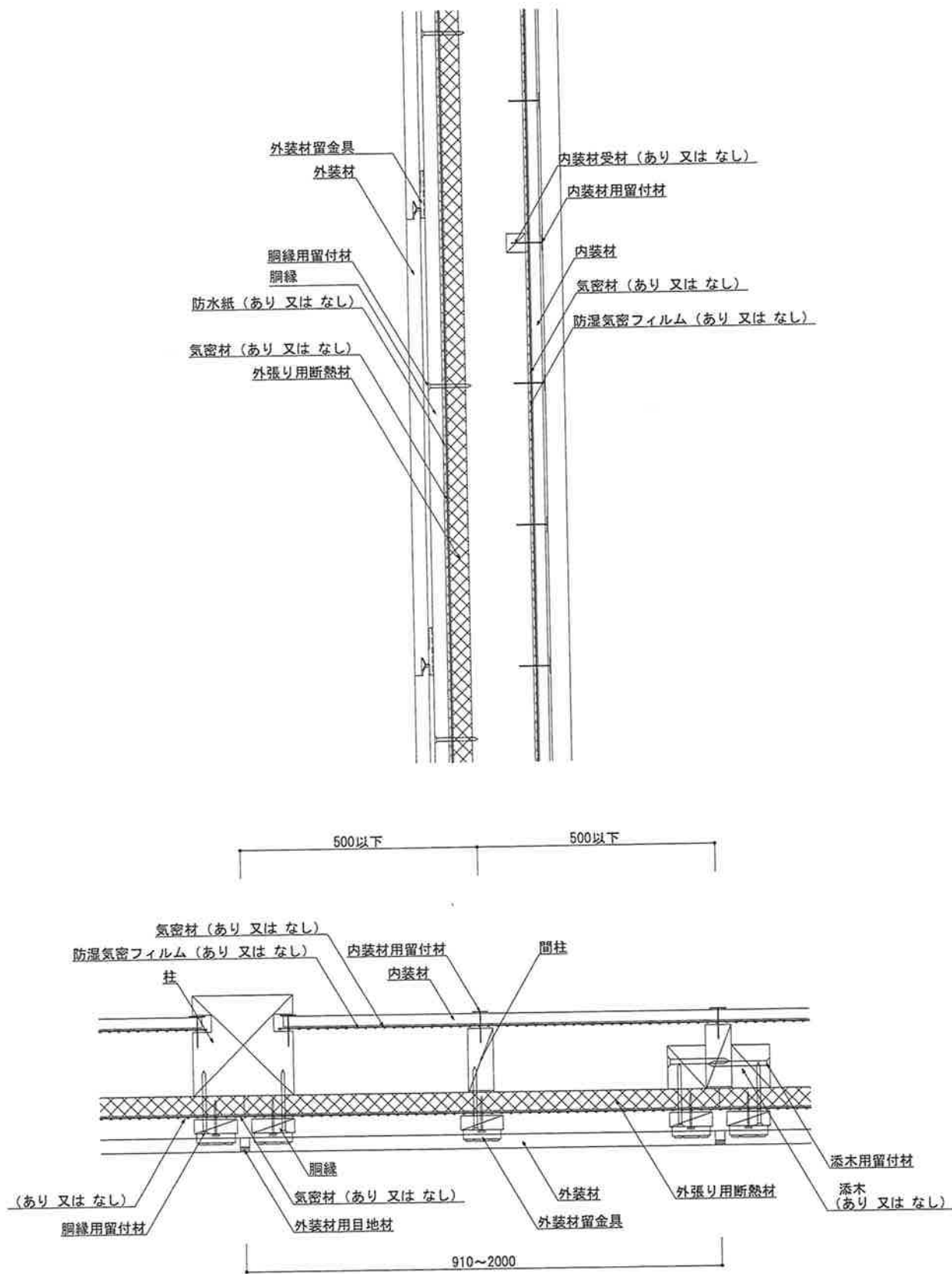
図4 構造説明図 (断面図・充てん断熱材なし/構造用面材なし/内装材真壁①)
