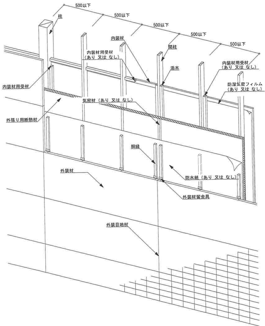
図5 構造説明図 (透視図・充てん断熱材なし/構造用面材なし/内装材真壁②)
