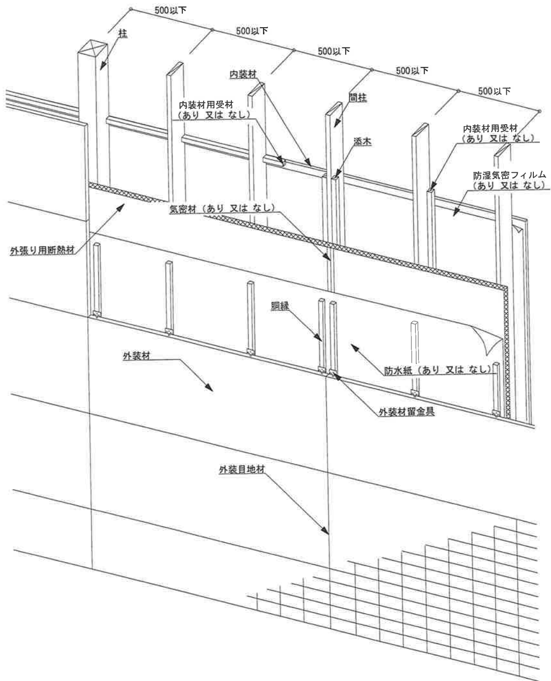
図1 構造説明図 (透視図・充てん断熱材なし／構造用面材なし／内装材大壁)
