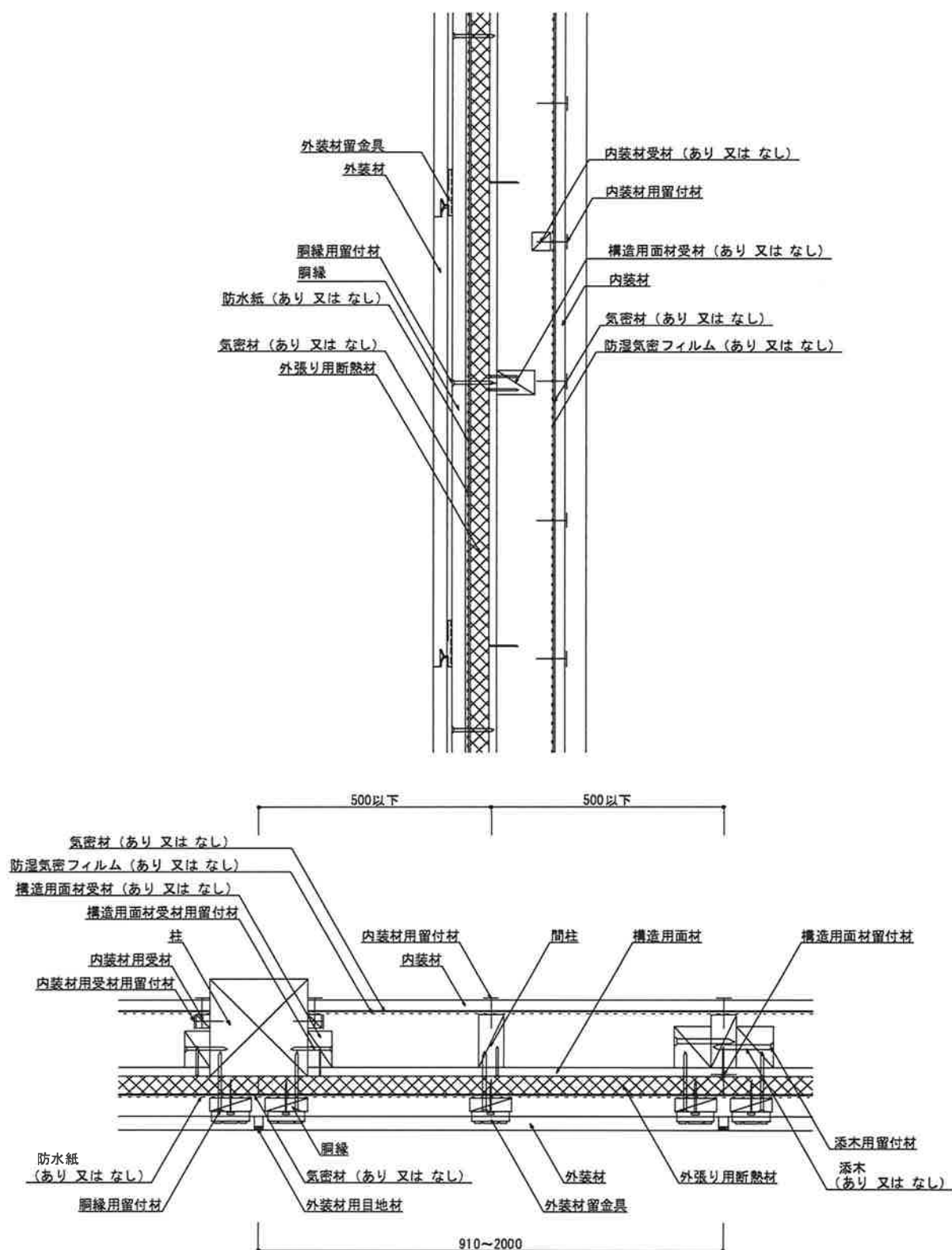
図12 構造説明図 (断面図・充てん断熱材なし／構造用面材真壁／内装材真壁②)
