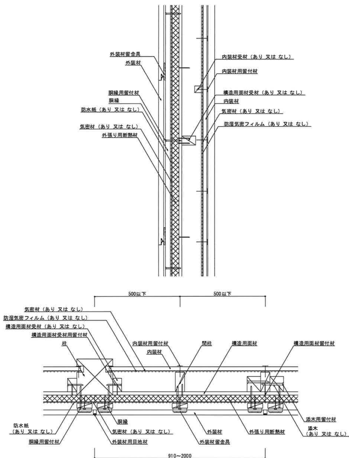
図10 構造説明図 (断面図・充てん断熱材なし／構造用面材真壁／内装材真壁①)
