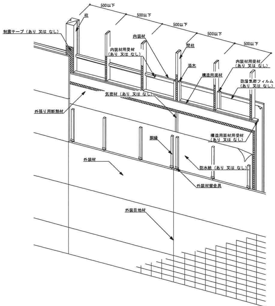
図3 構造説明図 (透視図・充てん断熱材なし／構造用面材大壁／内装材真壁①)
