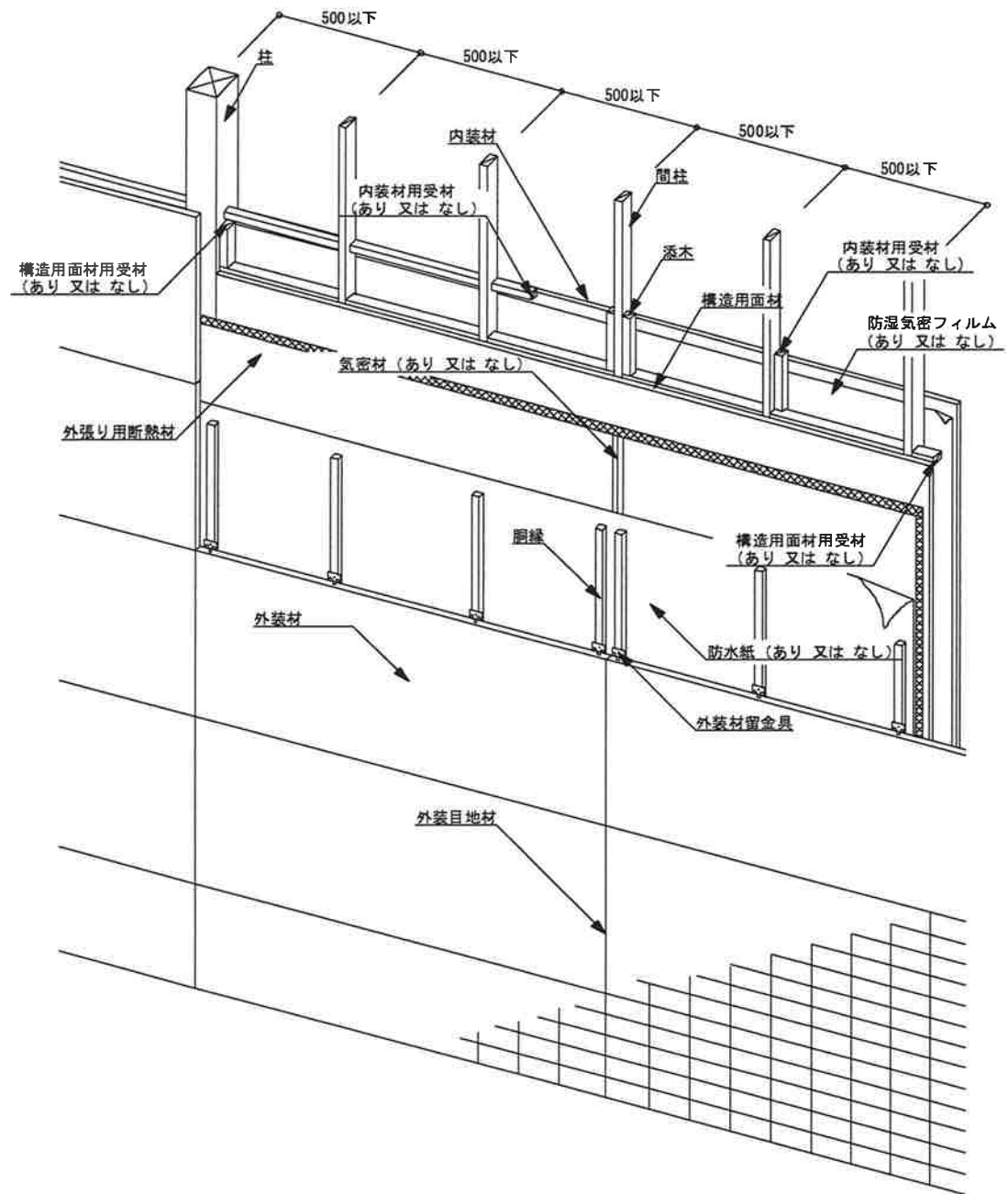
図11 構造説明図 (透視図・充てん断熱材なし／構造用面材真壁／内装材真壁②)
