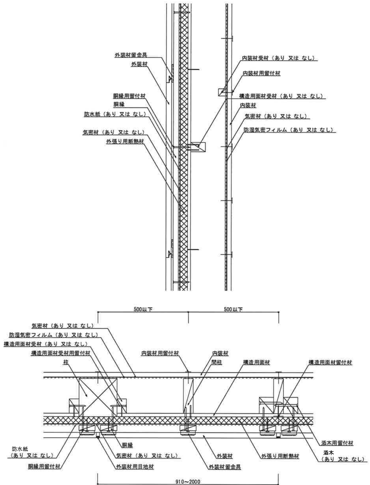
図8 構造説明図 (断面図・充てん断熱材なし／構造用面材真壁／内装材大壁)
