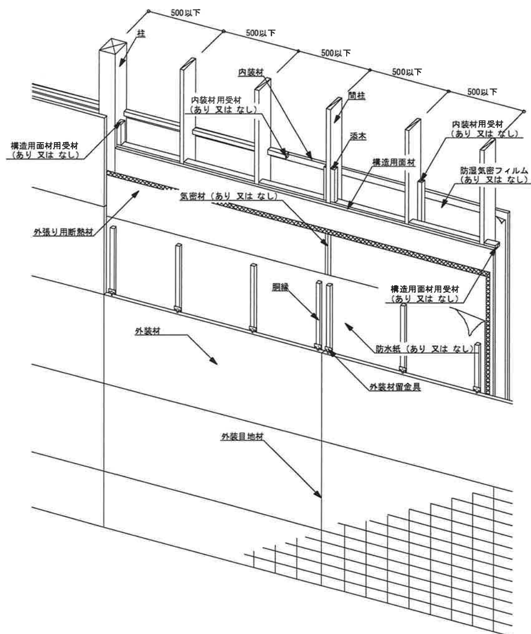
図7 構造説明図 (透視図・充てん断熱材なし／構造用面材真壁／内装材大壁)
