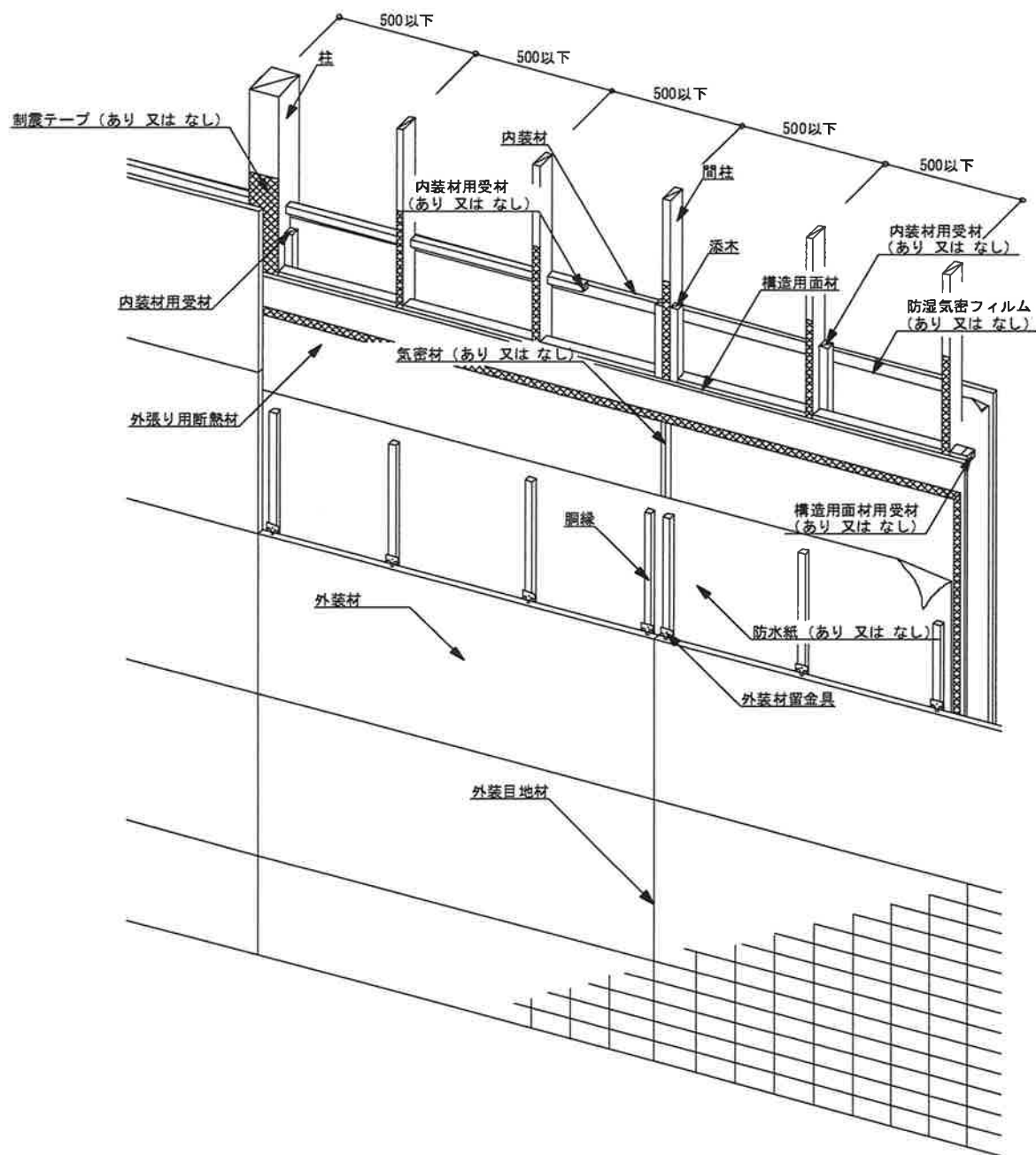
図5 構造説明図 (透視図・充てん断熱材なし／構造用面材大壁／内装材真壁②)
