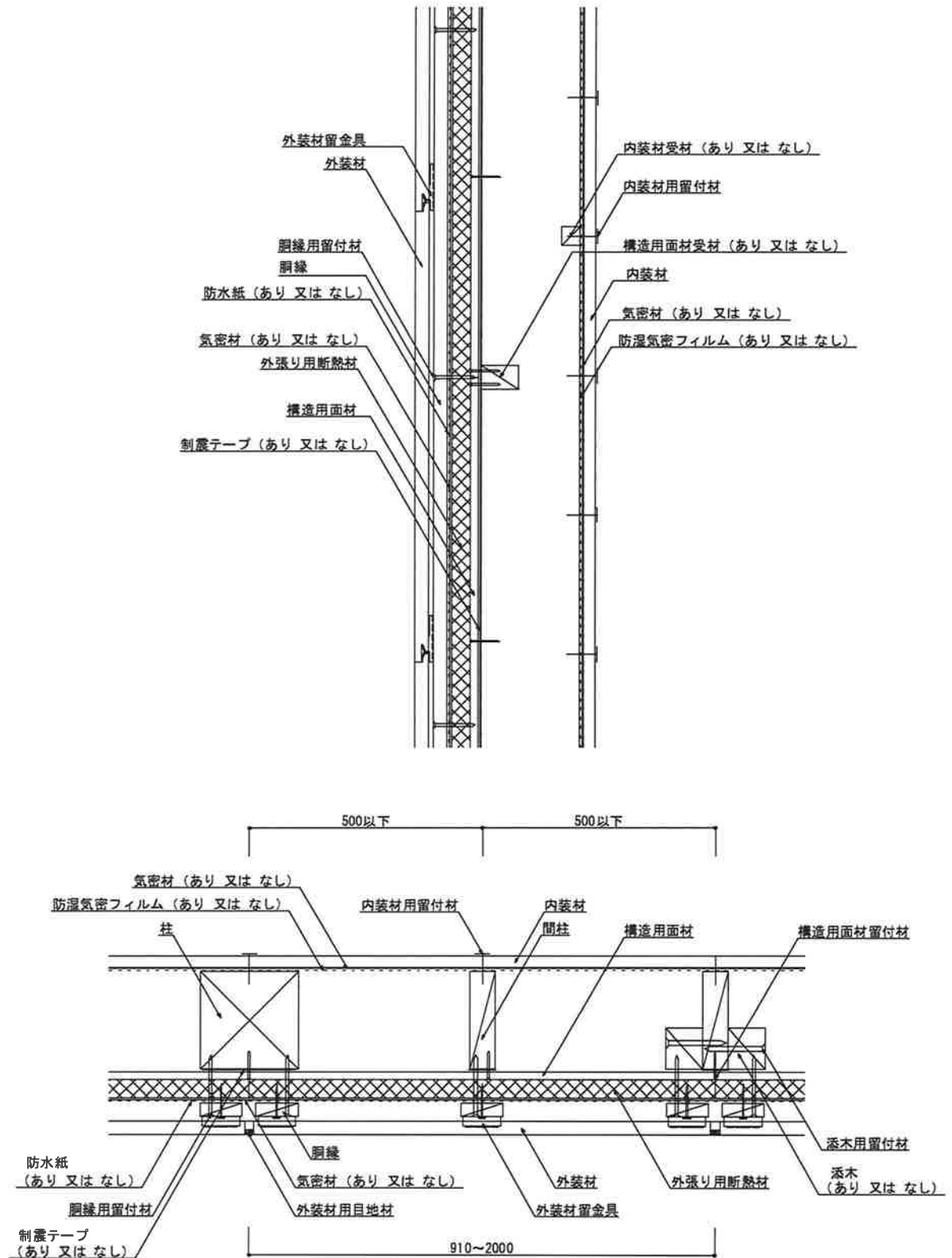
図2 構造説明図 (断面図・充てん断熱材なし／構造用面材大壁／内装材大壁)
