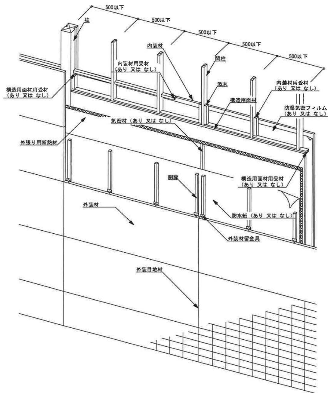
図9 構造説明図 (透視図・充てん断熱材なし／構造用面材真壁／内装材真壁①)
