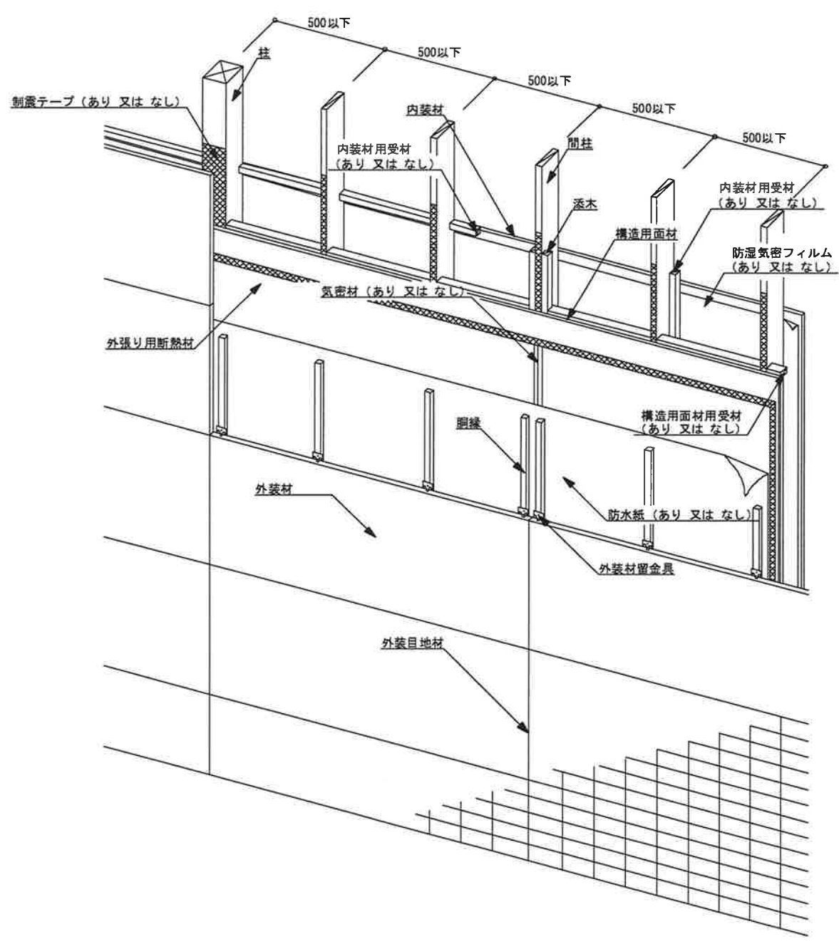
図1 構造説明図 (透視図・充てん断熱材なし／構造用面材大壁／内装材大壁)
