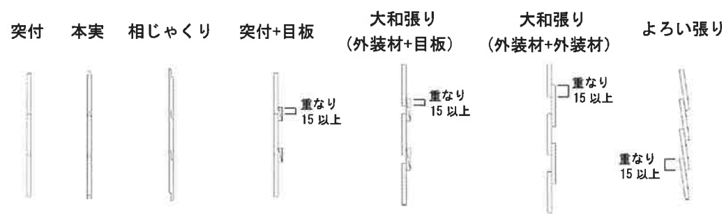
図 1 9 構造説明図
