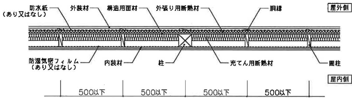
水平断面図
