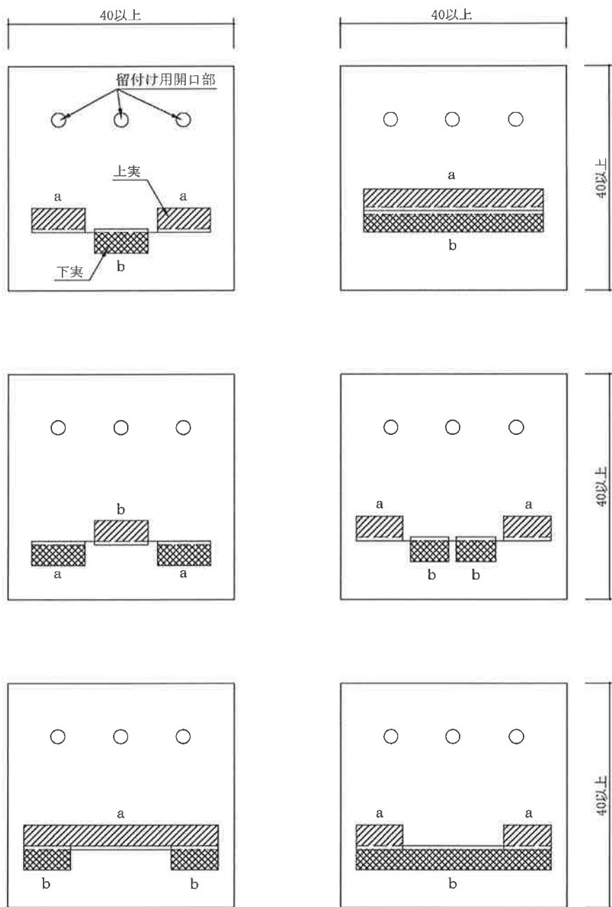
(正面図)
