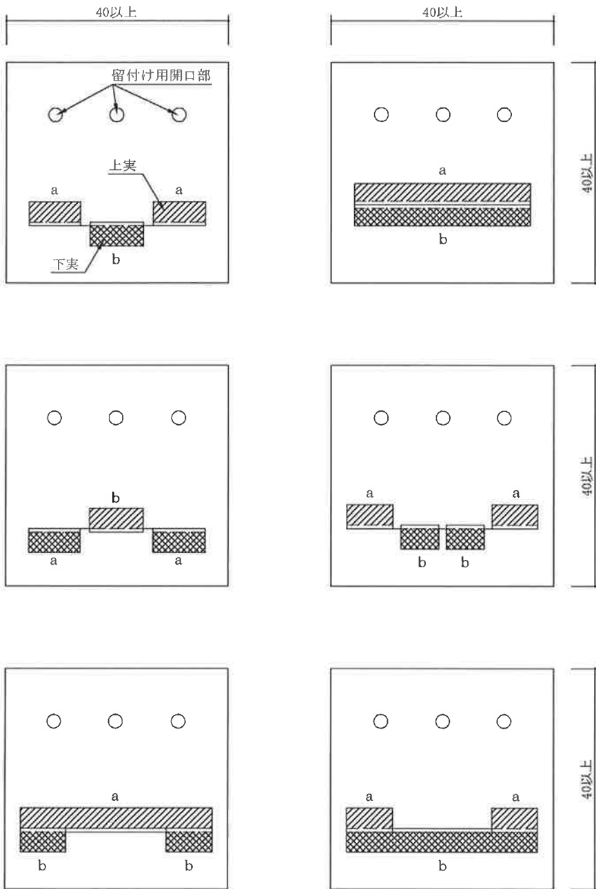
(正面図)
