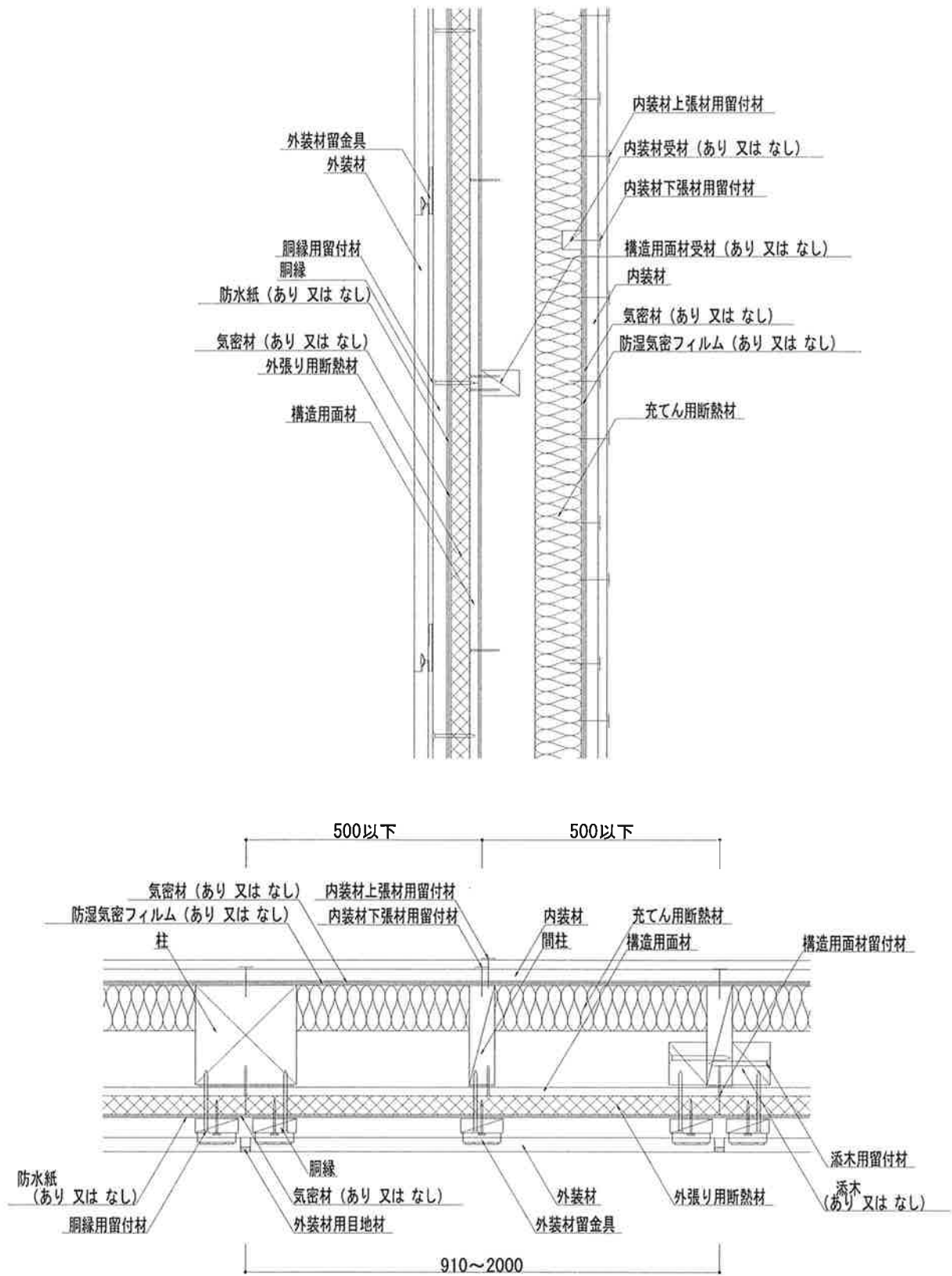
図2 構造説明図 (充てん断熱材あり)
