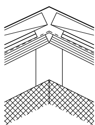
一般棟部の納まり図
