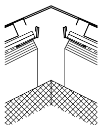
一般棟部の納まり図
