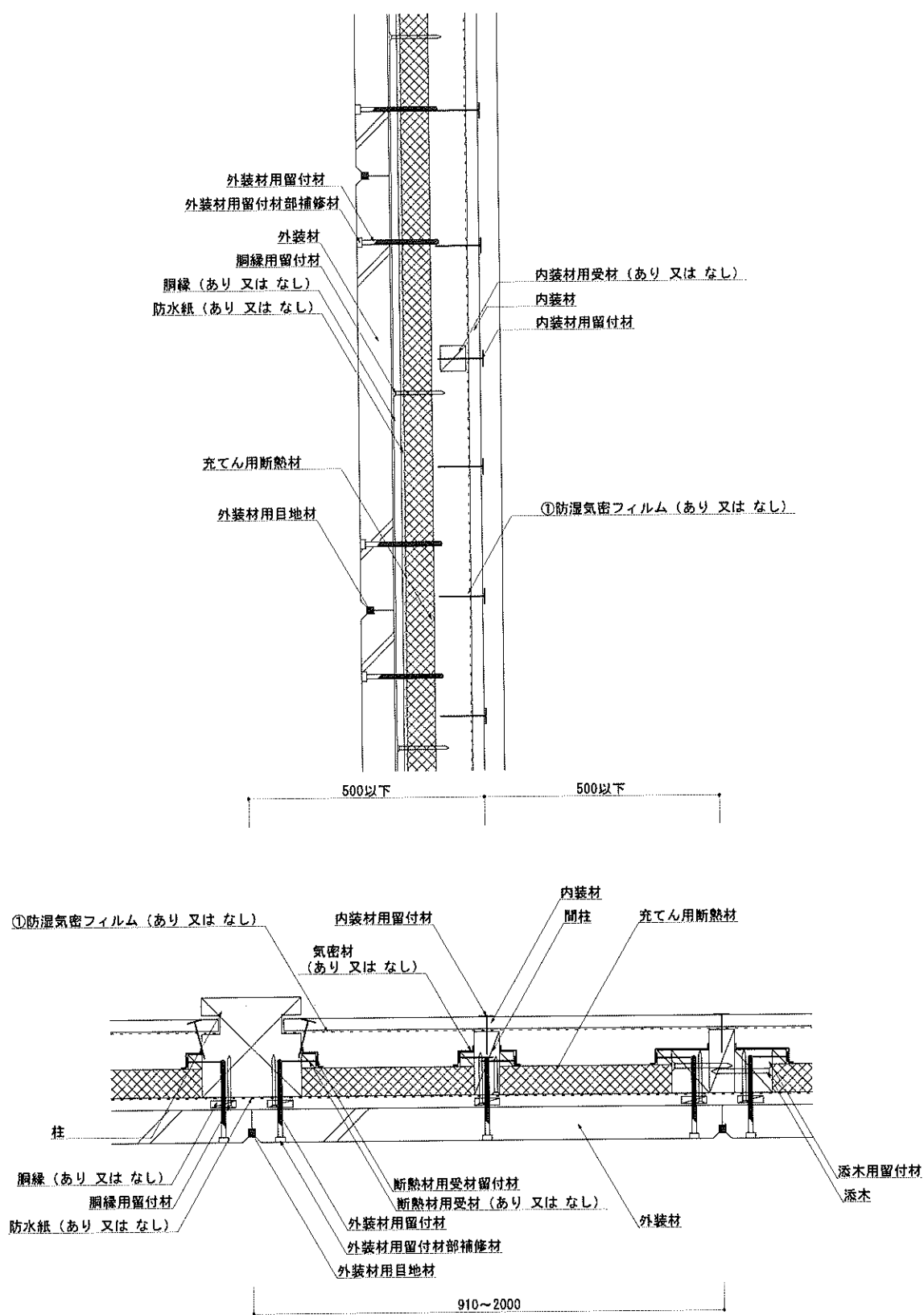
図6 構造説明図(水平垂直断面詳細図・構造用面材なし/内装材真壁②/充てん断熱材)
