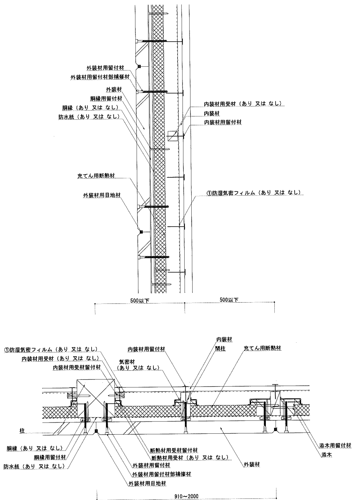
図4 構造説明図(水平垂直断面詳細図・構造用面材なし/内装材真壁①/充てん断熱材)
