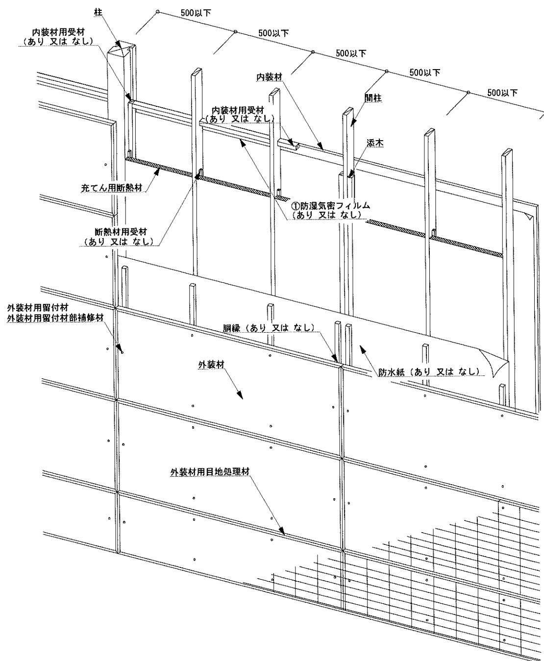
図5 構造説明図(透視図・構造用面材なし/内装材真壁②/充てん断熱材)
