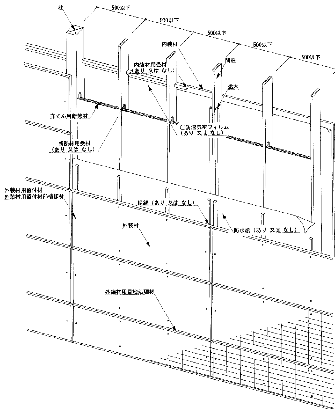
図1 構造説明図(透視図・構造用面材なし/内装材大壁/充填断熱材)
