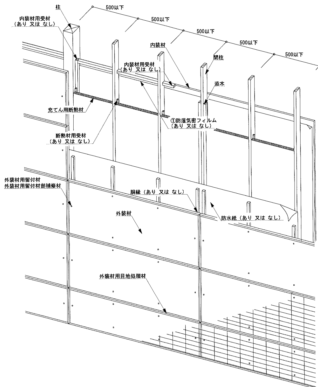
図3 構造説明図(透視図・構造用面材なし／内装材真壁①／充てん断熱材)
