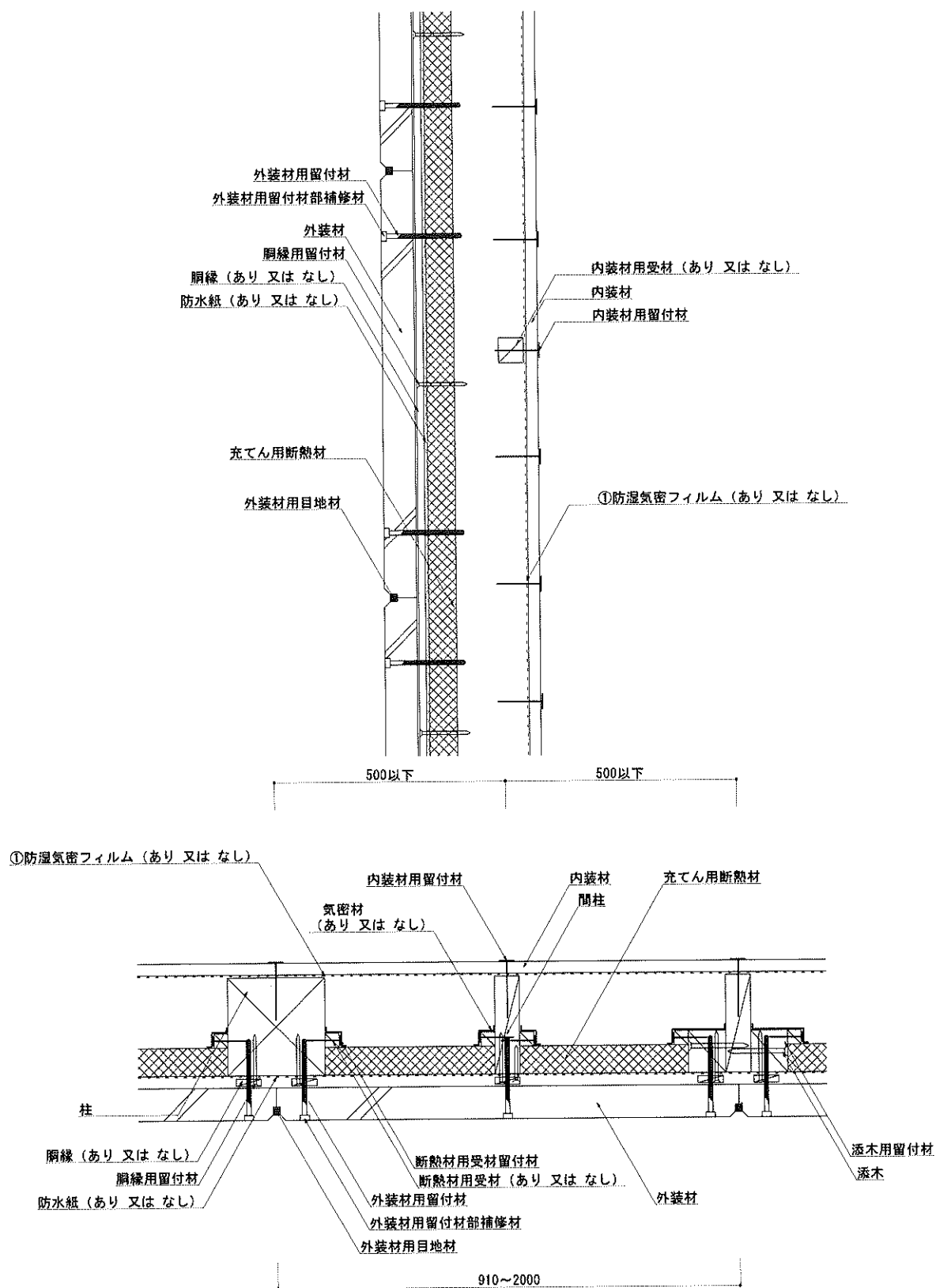
図2 構造説明図(水平垂直断面詳細図・構造用面材なし/内装材大壁/充てん断熱材)
