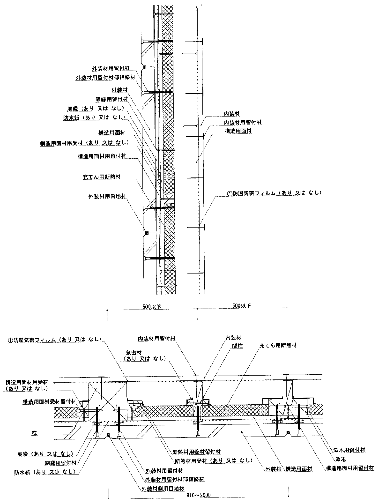
図8 構造説明図(水平垂直断面詳細図・構造用面材 屋外側真壁/屋内側なし/内装材大壁/充てん断熱材)
