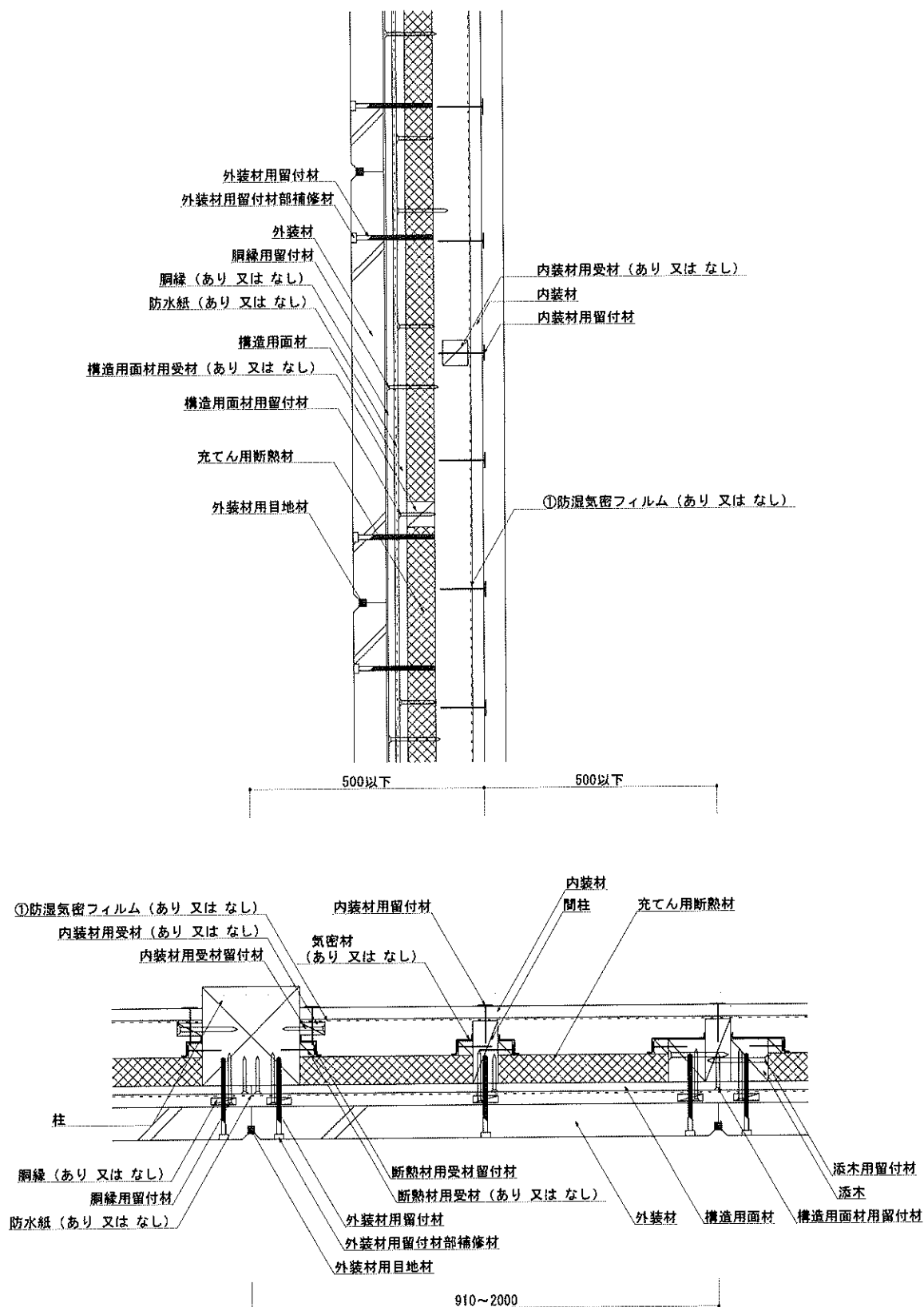
図4 (水平垂直断面詳細図・構造用面材 屋外側大壁／屋内側なし／内装材真壁①／充てん断熱材)
