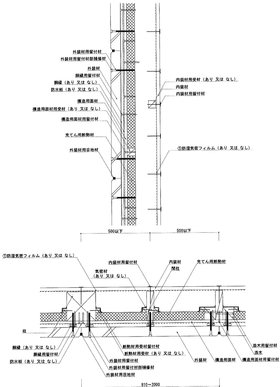
図2 構造説明図(水平垂直断面詳細図・構造用面材 屋外側大壁/屋内側なし/内装材大壁/充てん断熱材)
