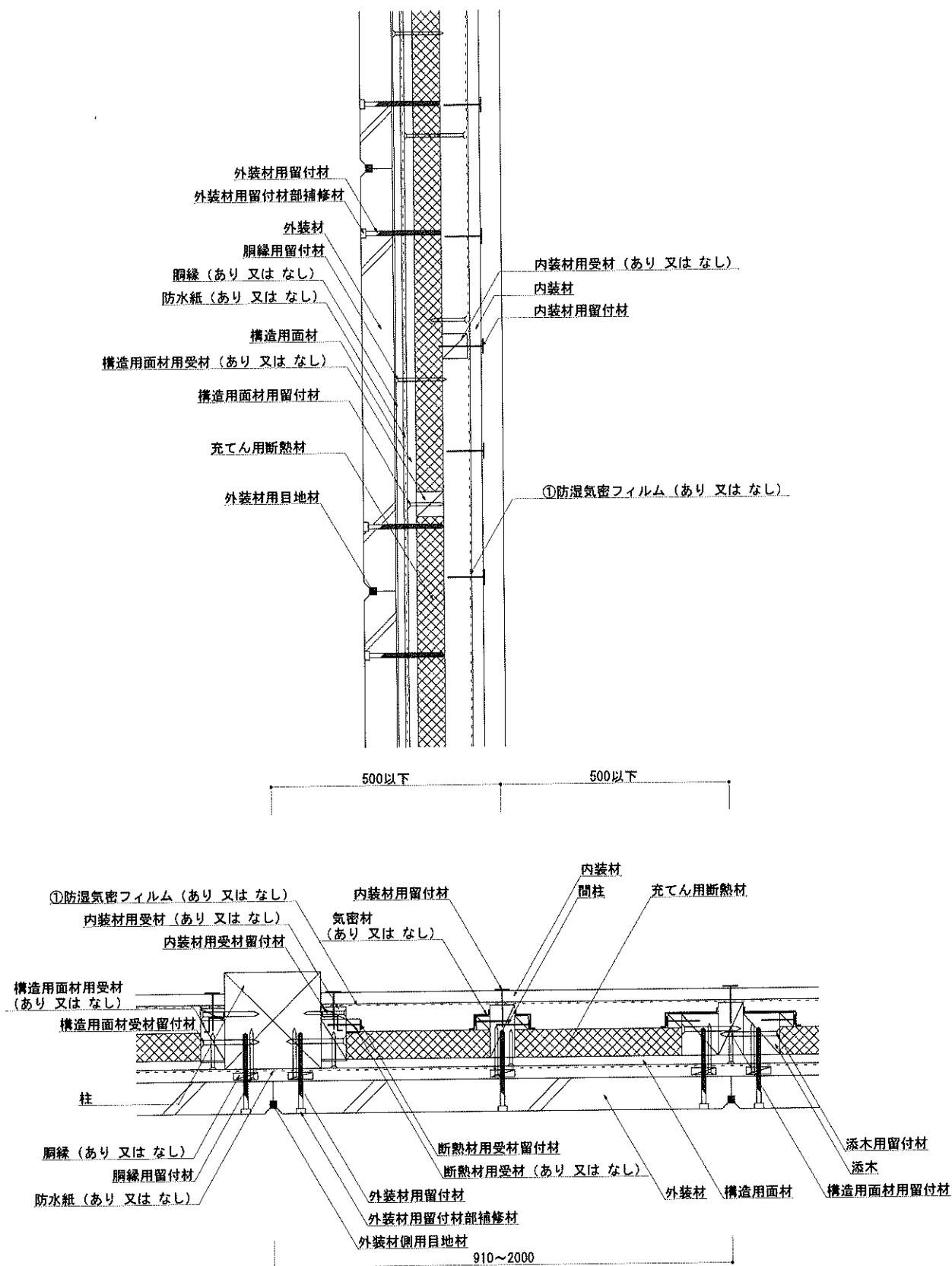
図10 構造説明図(水平垂直断面詳細図・構造用面材 屋外側真壁/屋内側なし/内装材真壁①/充てん断熱材)
