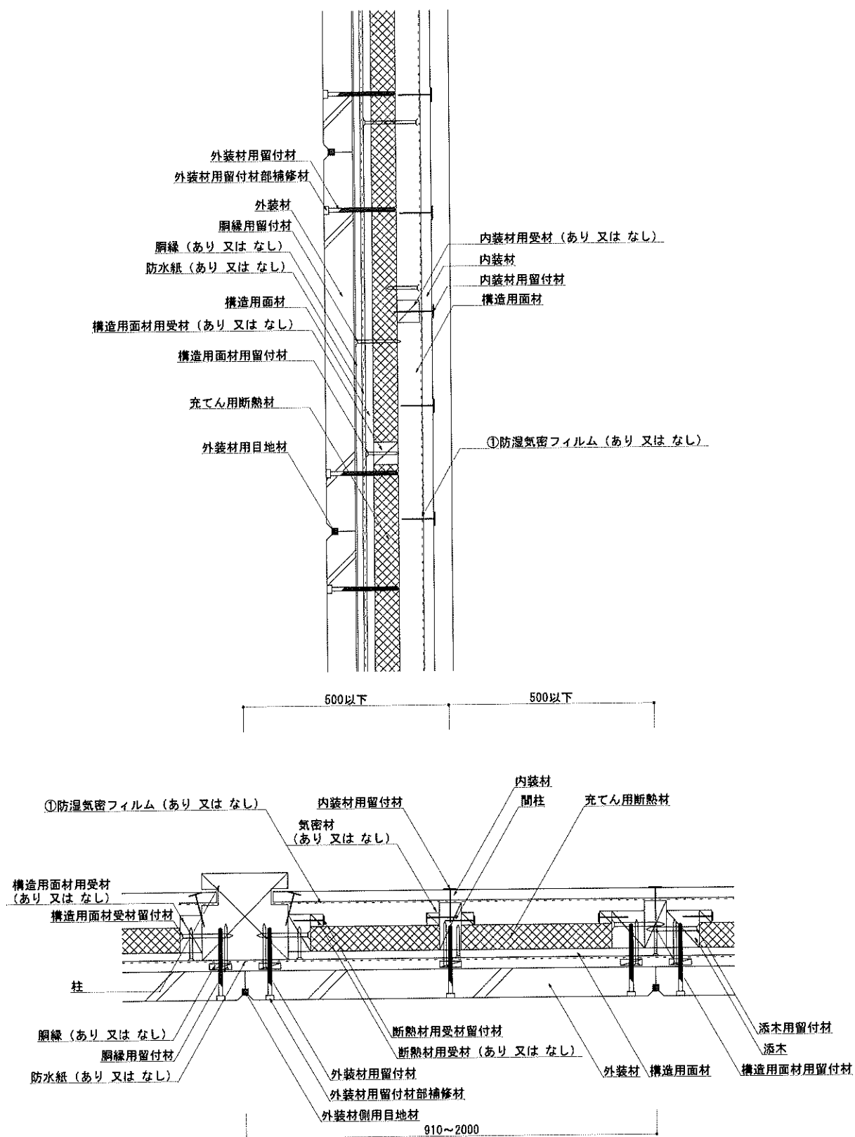
図12 構造説明図(水平垂直断面詳細図・構造用面材 屋外側真壁/屋内側なし/内装材真壁②/充てん断熱材)
