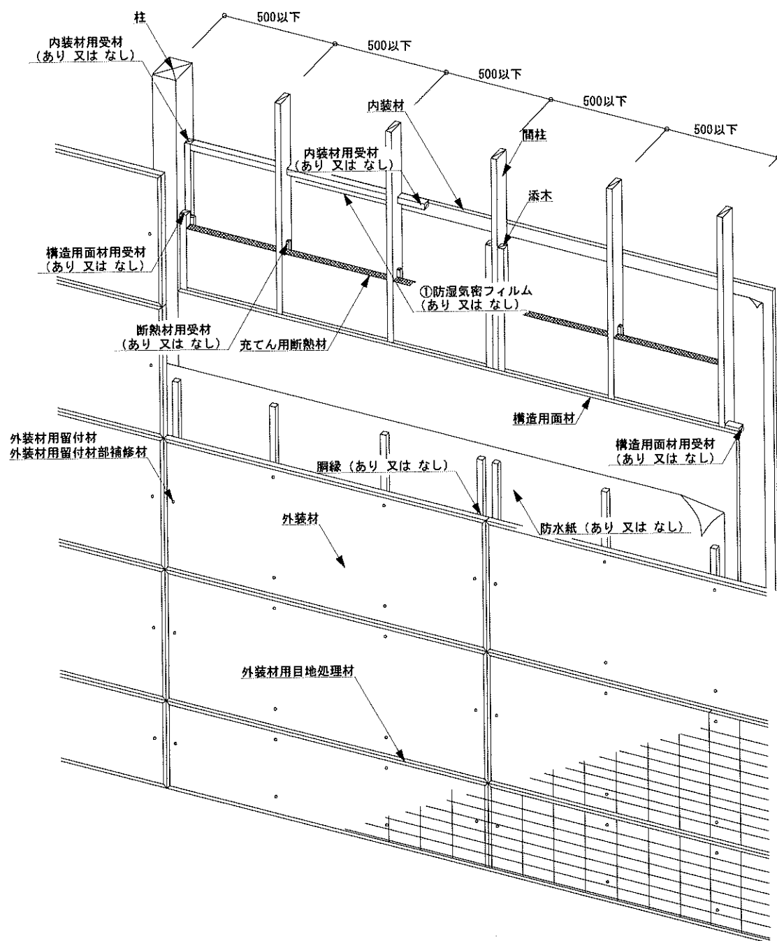
図9 構造説明図(透視図・構造用面材 屋外側真壁/屋内側なし/内装材真壁①/充てん断熱材)
