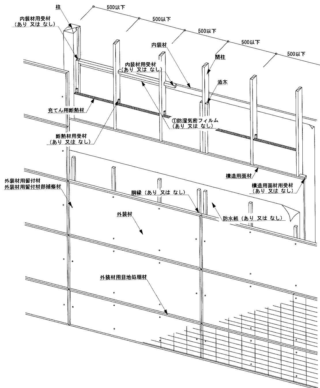
図5 構造説明図(透視図・構造用面材 屋外側大壁/屋内側なし/内装材真壁②/充てん断熱材)
