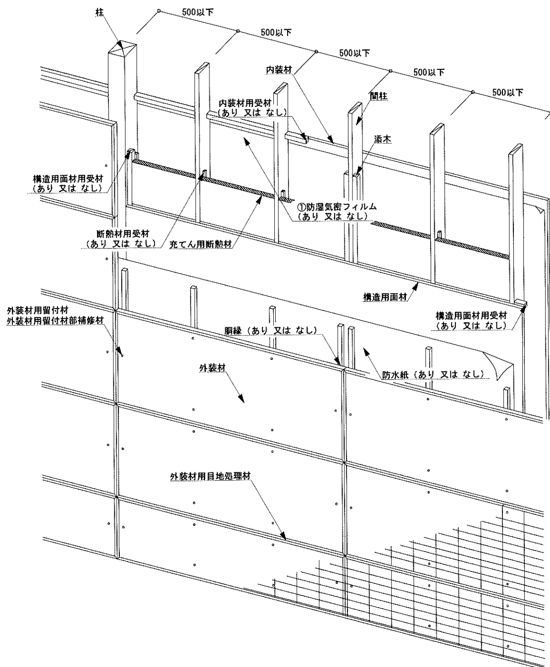
図7 構造説明図(透視図・構造用面材 屋外側真壁/屋内側なし/内装材大壁/充てん断熱材)
