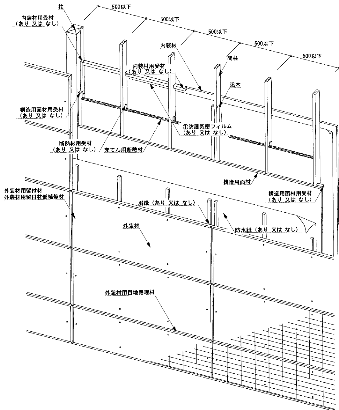
図11 構造説明図(透視図・構造用面材 屋外側真壁/屋内側なし/内装材真壁②/充てん断熱材)
