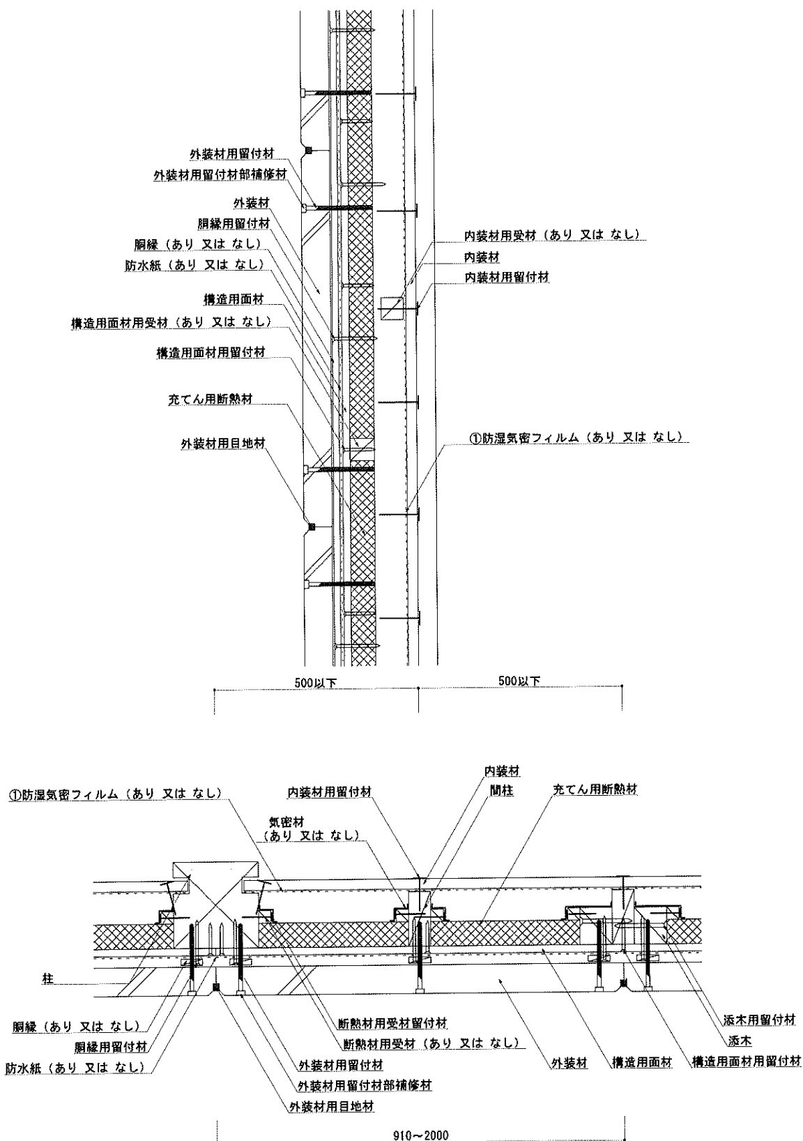
図6 構造説明図(水平垂直断面詳細図・構造用面材 屋外側大壁/屋内側なし/内装材真壁②/充てん断熱材)
