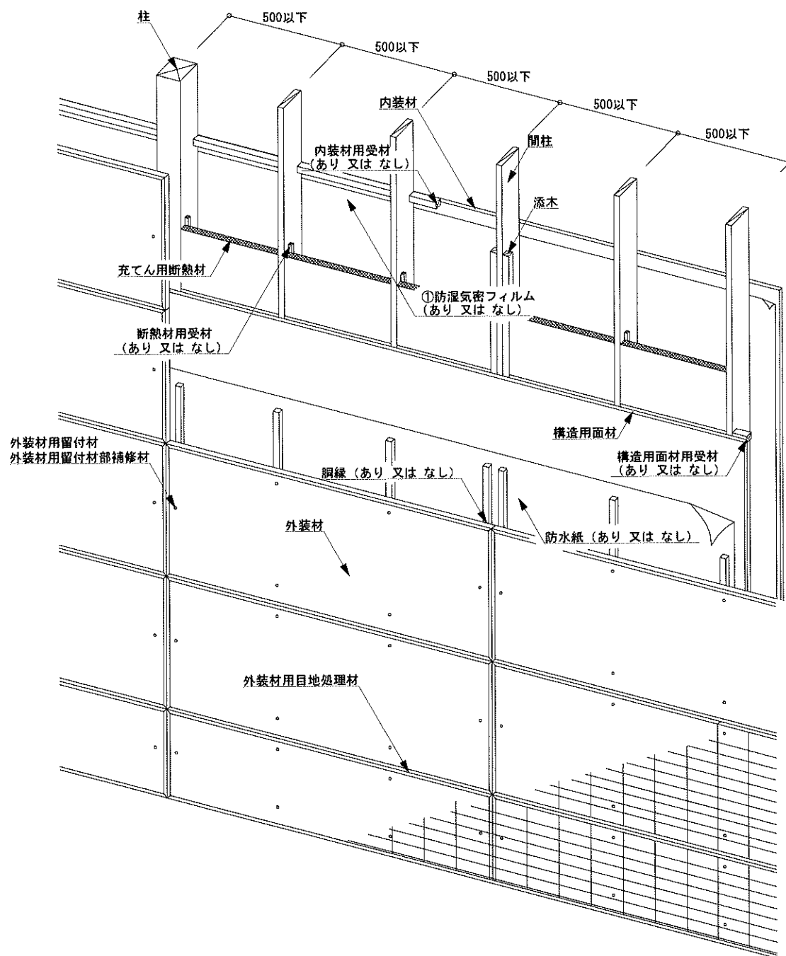
図1 構造説明図(透視図・構造用面材 屋外側大壁/屋内側なし/内装材大壁/充てん断熱材)
