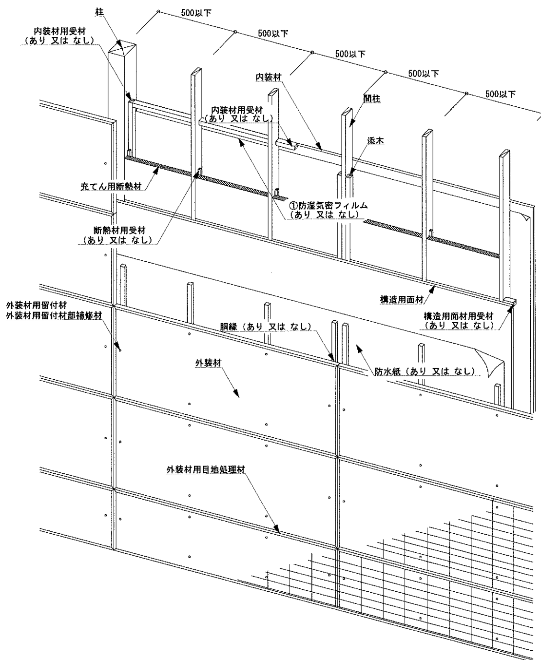
図3 構造説明図(透視図・構造用面材 屋外側大壁/屋内側なし/内装材真壁①/充填断熱材)
