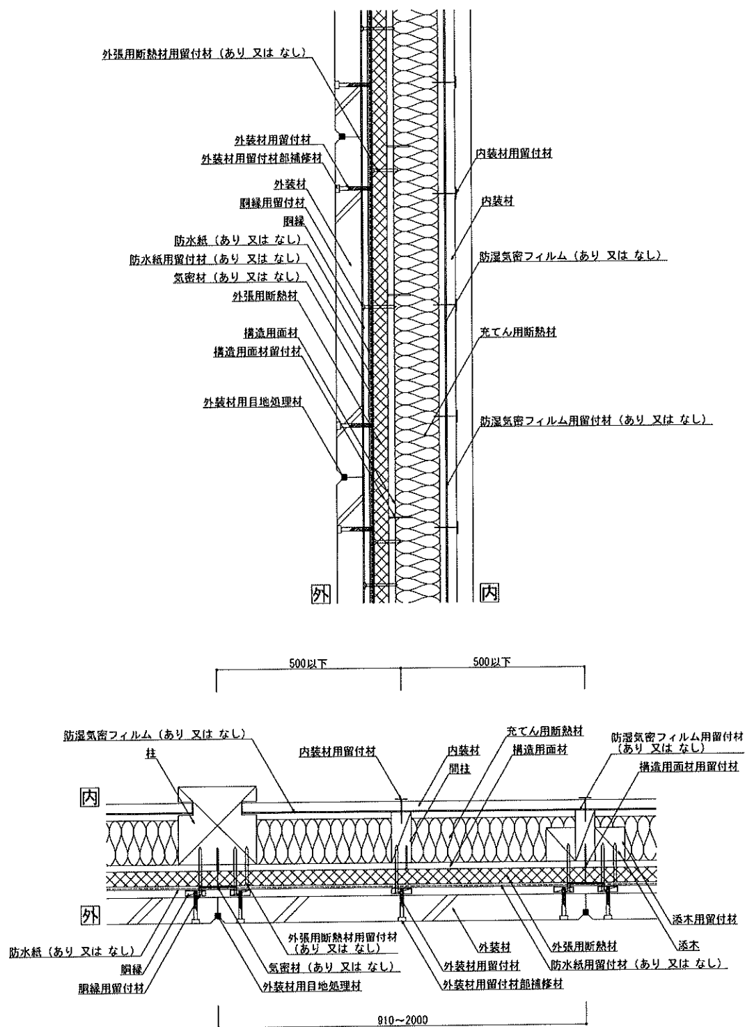
図8 構造説明図(水平垂直断面詳細図・構造用面材大壁／内装材真壁①／充てん用断熱材あり)
