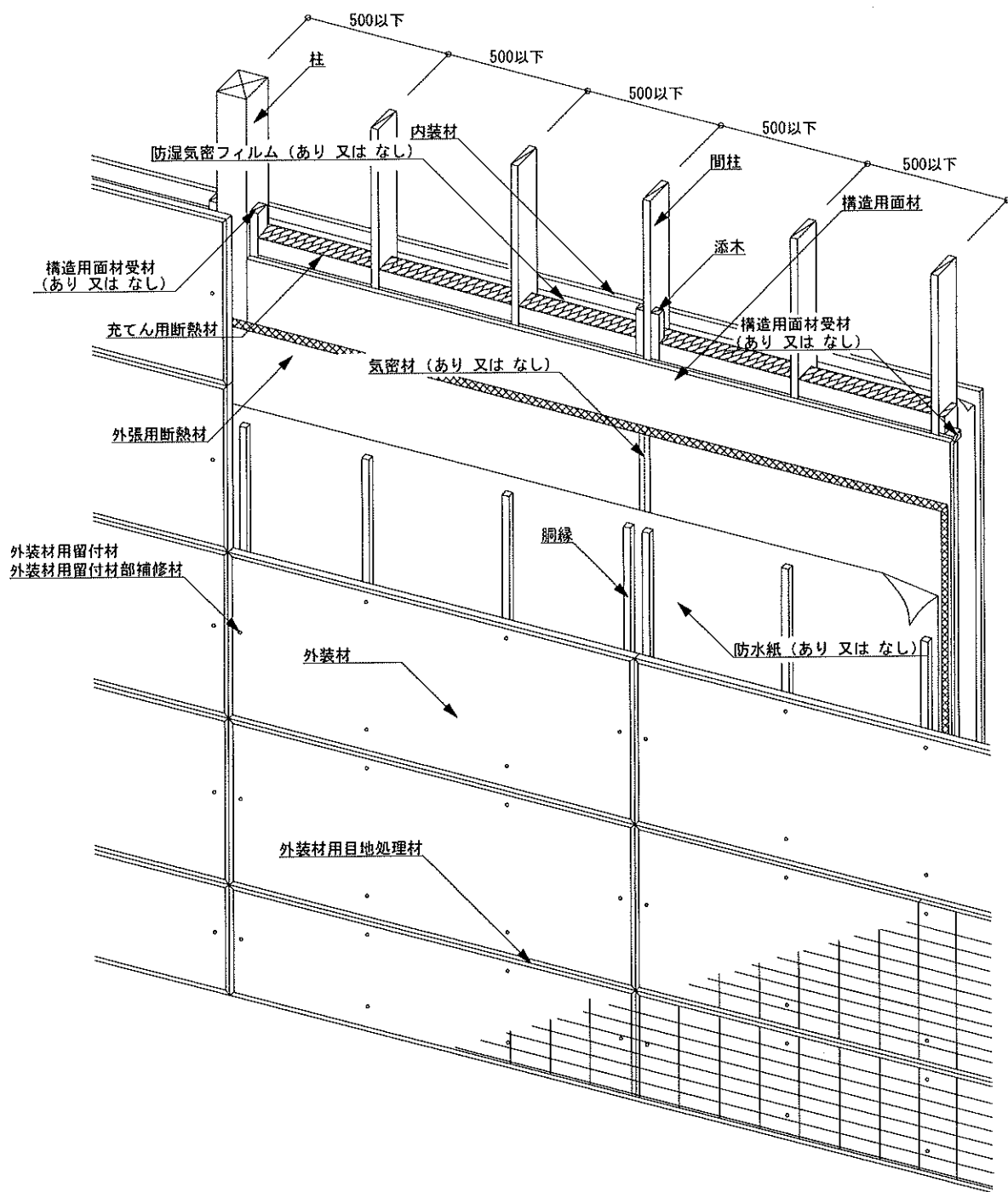
図5 構造説明図(透視図・構造用面材真壁／内装材大壁／充てん用断熱材あり)
