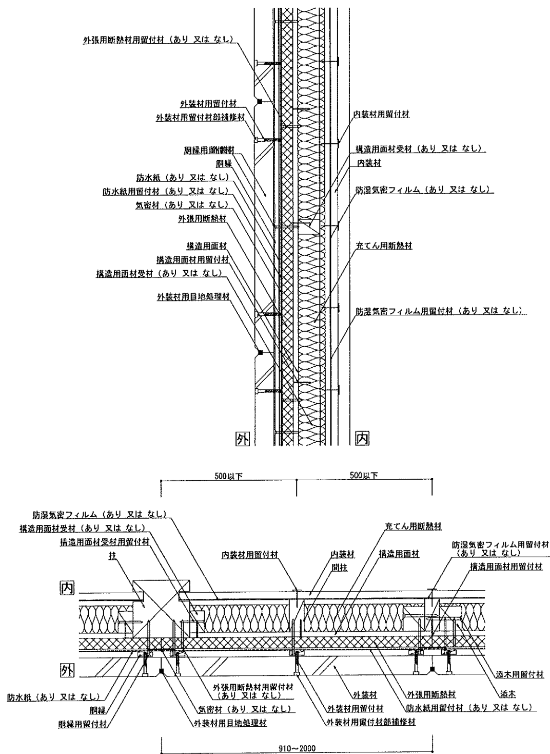
図2 構造説明図(水平垂直断面詳細図・構造用面材真壁／内装材真壁①／充てん用断熱材あり)
