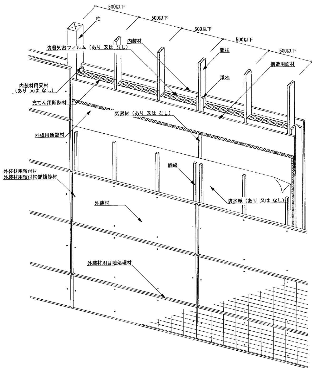
図9 構造説明図(透視図・構造用面材大壁／内装材真壁②／充填用断熱材あり)
