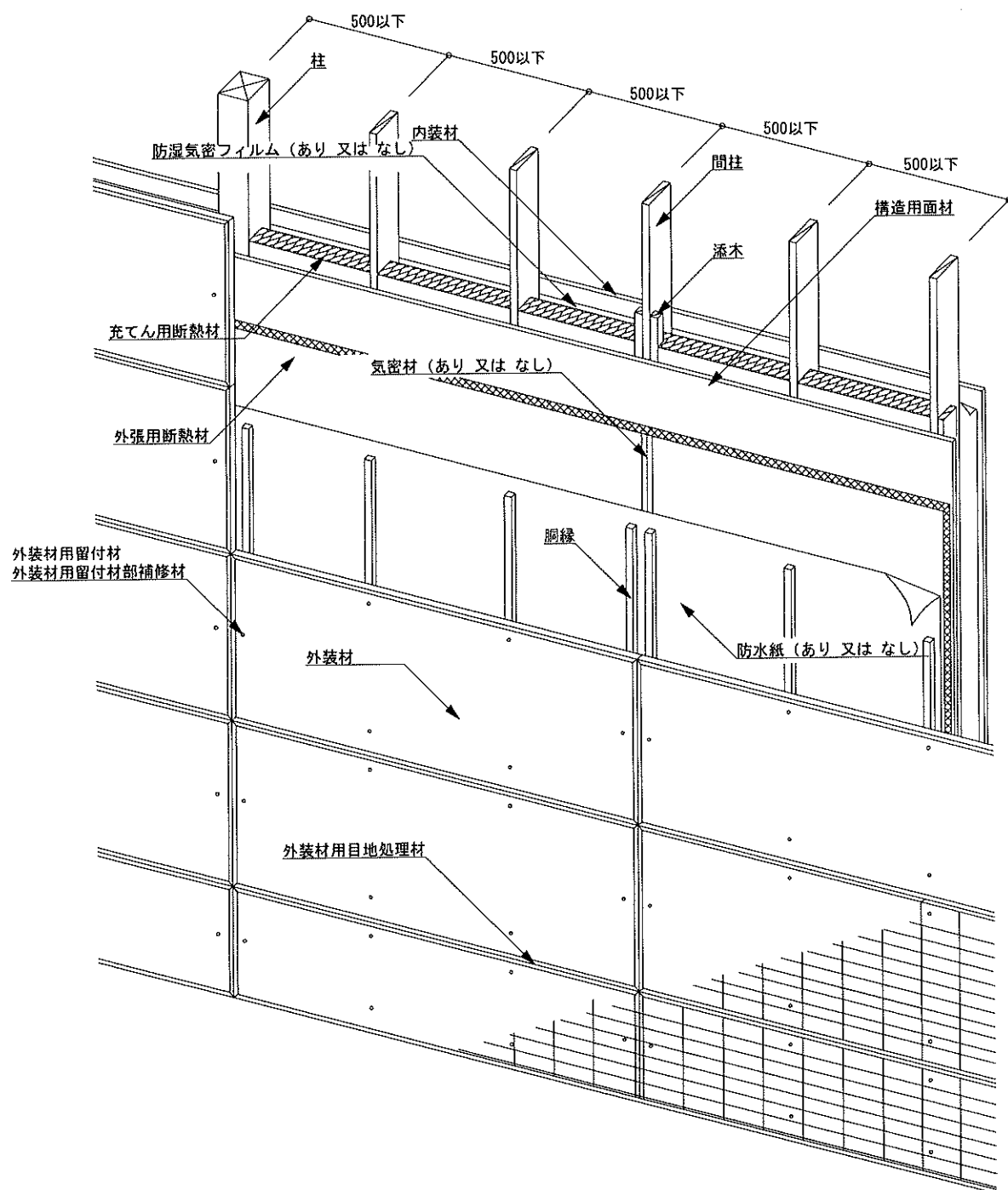
図11 構造説明図(透視図・構造用面材大壁／内装材大壁／充てん用断熱材あり)
