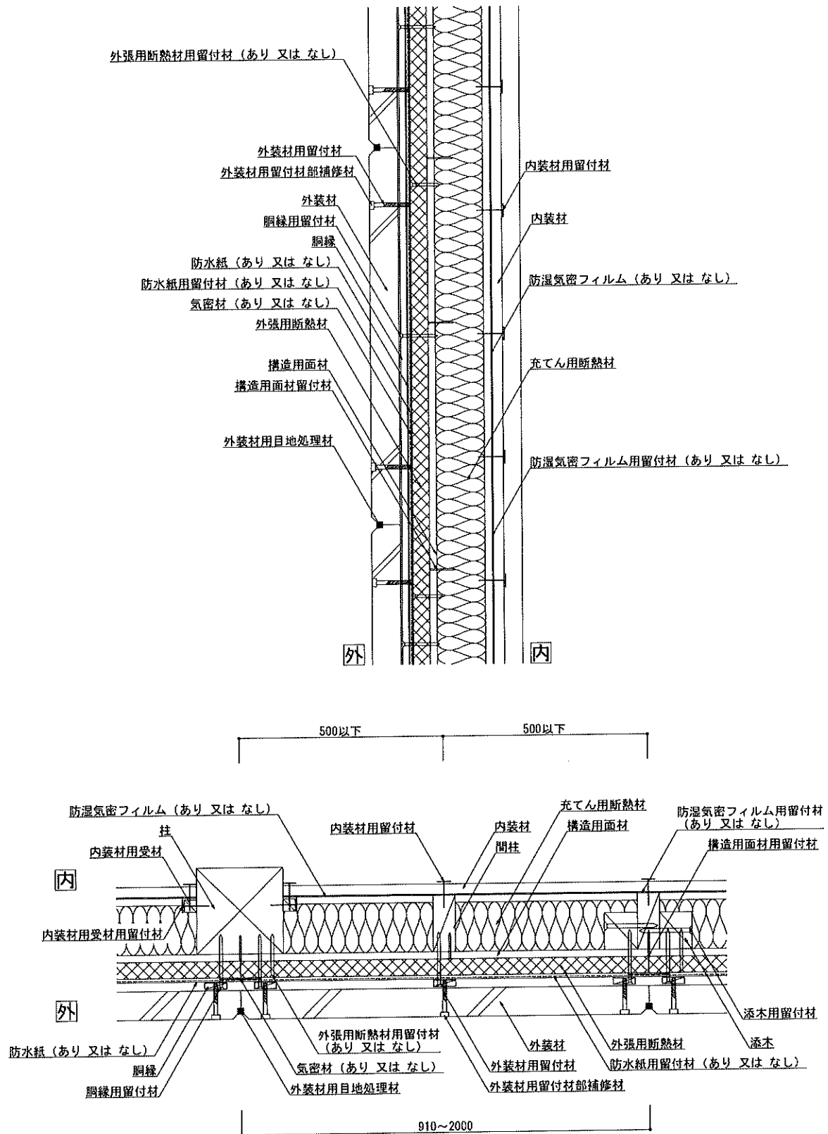
図10 構造説明図(水平垂直断面詳細図・構造用面材大壁／内装材真壁②／充てん用断熱材あり)
