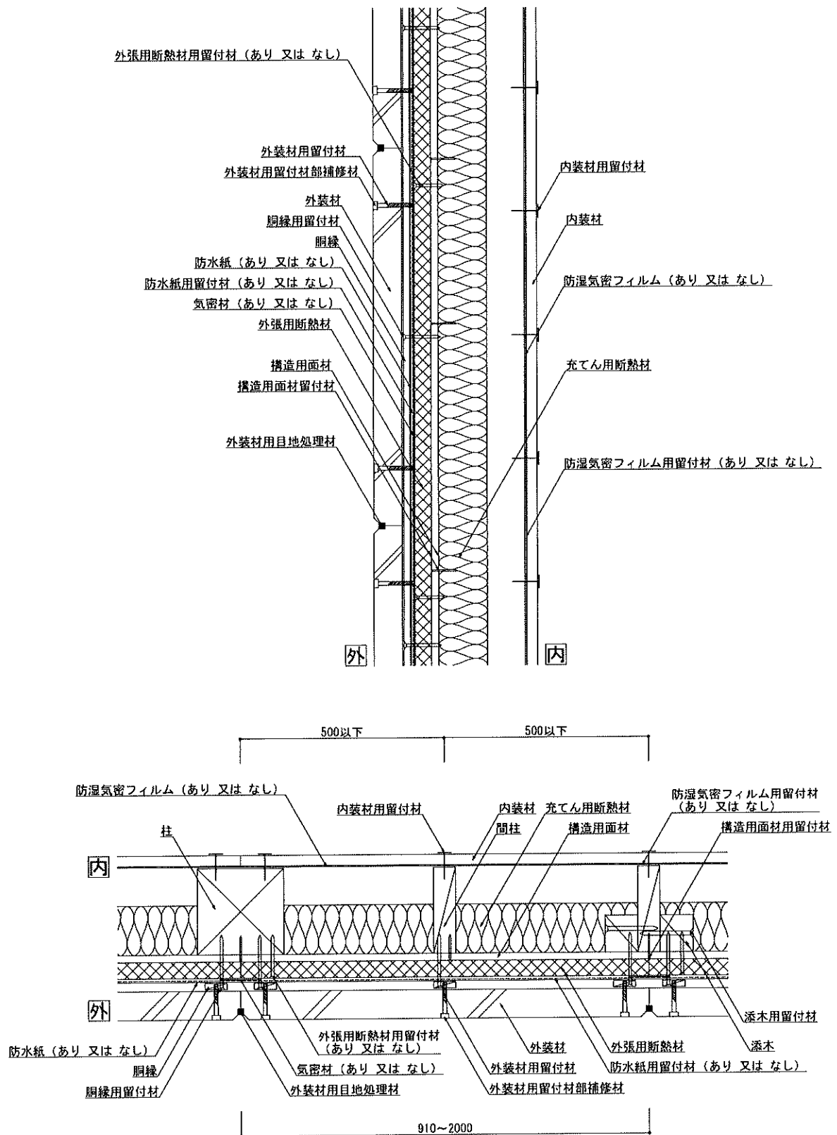
図12 構造説明図(水平垂直断面詳細図・構造用面材大壁／内装材大壁／充填用断熱材あり)
