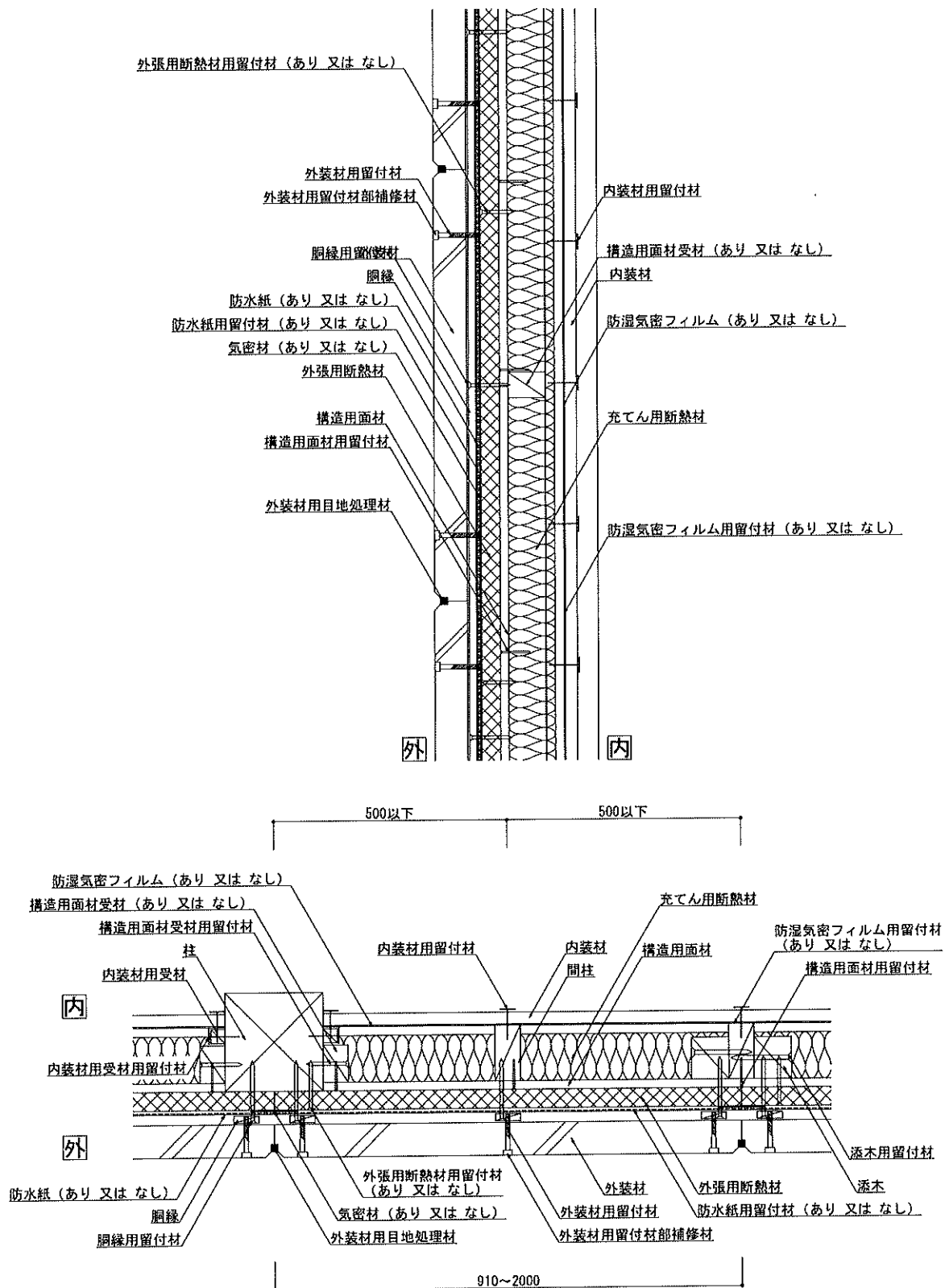
図4 構造説明図(水平垂直断面詳細図・構造用面材真壁／内装材真壁②／充てん用断熱材あり)
