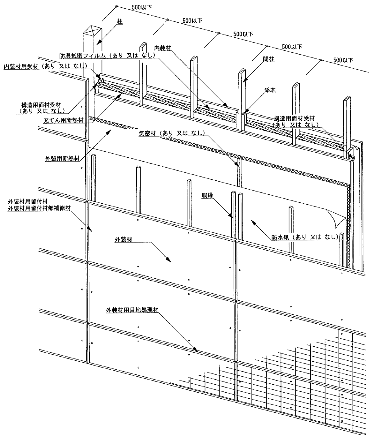
図3 構造説明図(透視図・構造用面材真壁／内装材真壁②／充てん用断熱材あり)
