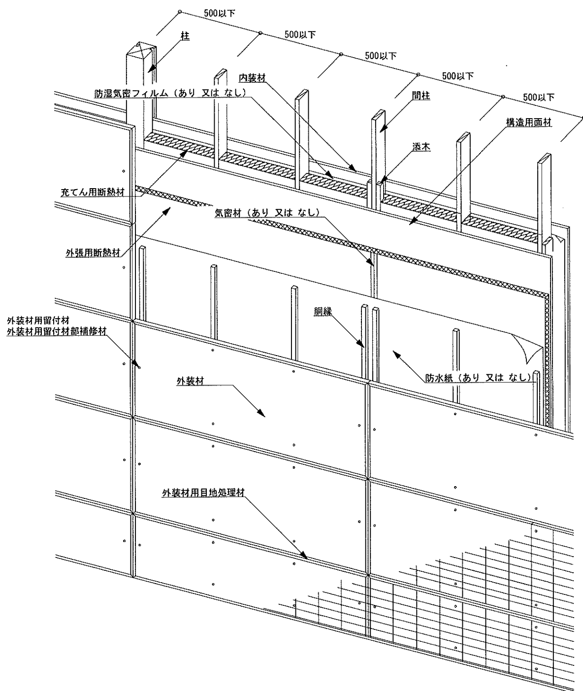
図7 構造説明図(透視図・構造用面材大壁／内装材真壁①／充てん用断熱材あり)
