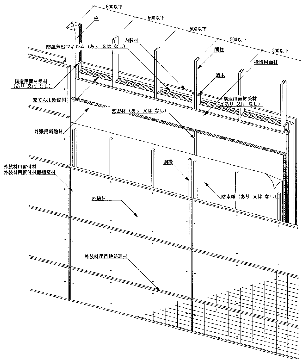
図1 構造説明図(透視図・構造用面材真壁／内装材真壁①／充てん用断熱材あり)
