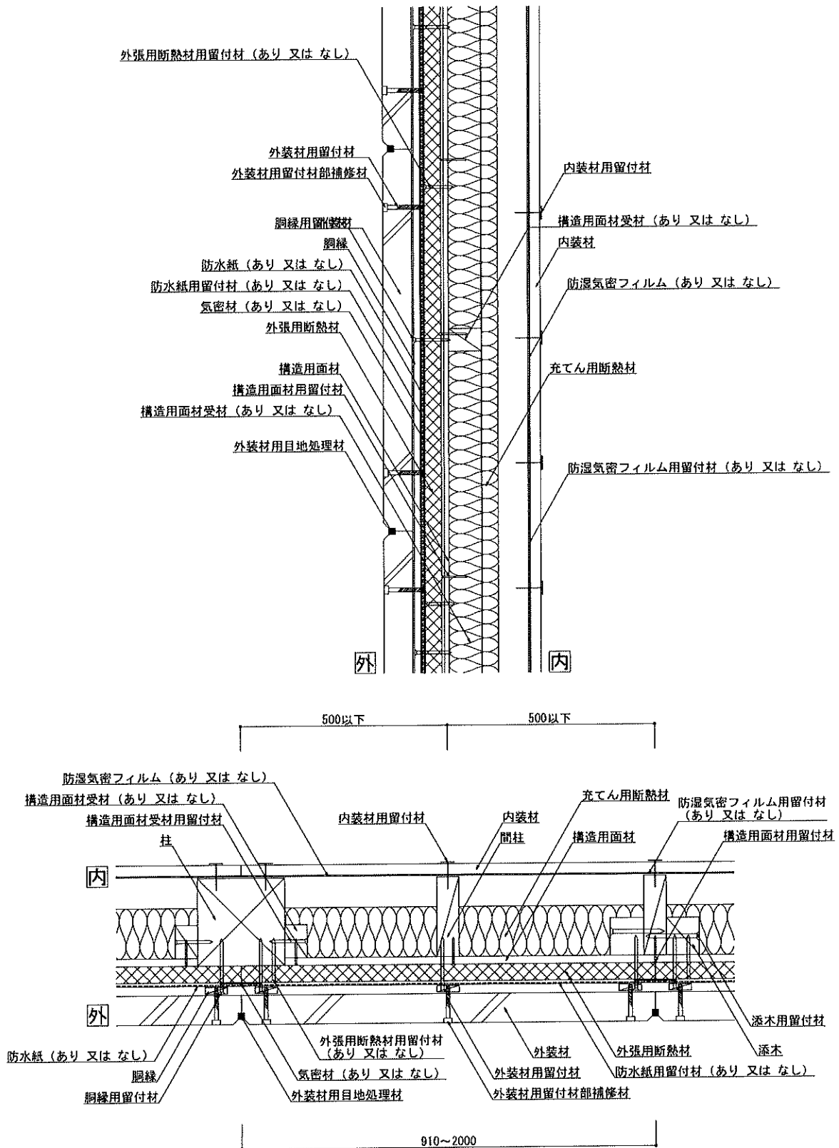
図6 構造説明図(水平垂直断面詳細図・構造用面材真壁／内装材大壁／充てん用断熱材あり)
