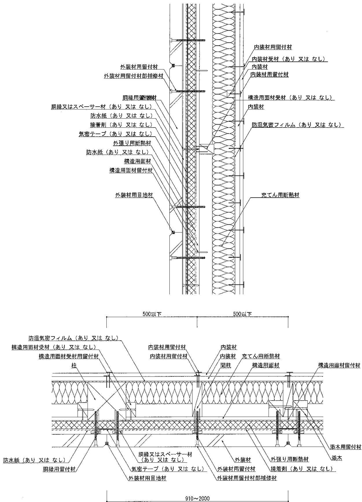
図4 構造説明図 (断面図・構造用面材真壁／内装材（重張）／充てん用断熱材あり）
